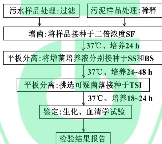
图 B.1 污水、污泥中沙门氏菌检验程序
