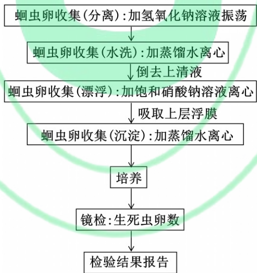
图 D.1 污泥中蛔虫卵检验程序
