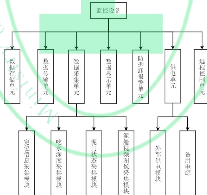
图 1 监控设备功能单元组成示意图
