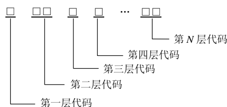
图 1 代码结构
