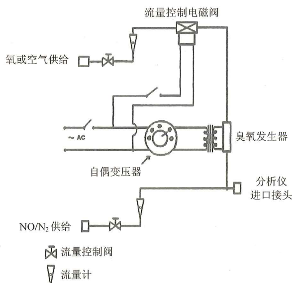
图 C.4 \text{NO}_x 转化器效率测试装置示意图
