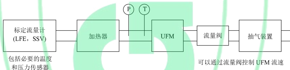
图 CD.8 UFM 标定布置图
