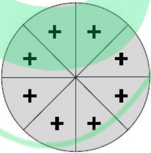
图 CD.2 圆形出口的风机
