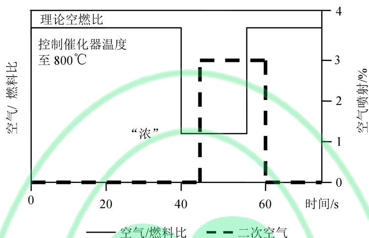
图 GA.1 标准台架循环
