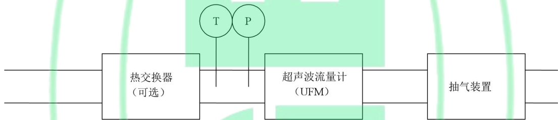
图 CD.5 超声波流量计 (UFM) 示意图
