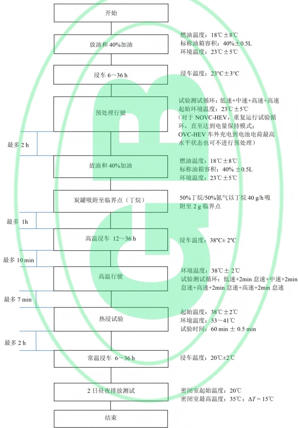
图 F.1a 装备整体炭罐、非整体炭罐系统（NIRC0 除外）汽车的蒸发污染物排放测定规程
