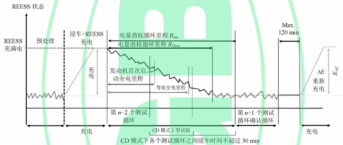
图 RA.1 电量消耗 I 型试验
