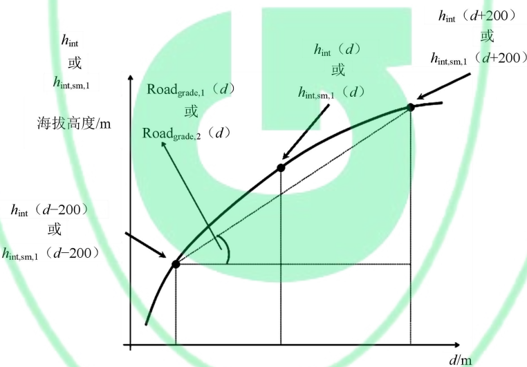
图 DH.1 插值高度信号光滑处理程序示意图
