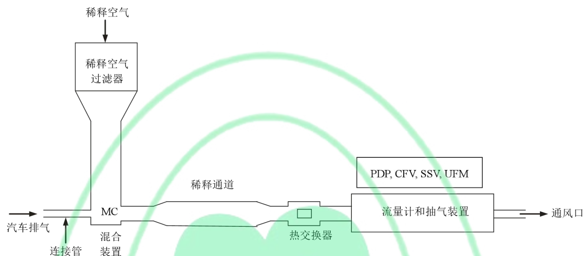
图 CD.3 排气稀释系统
