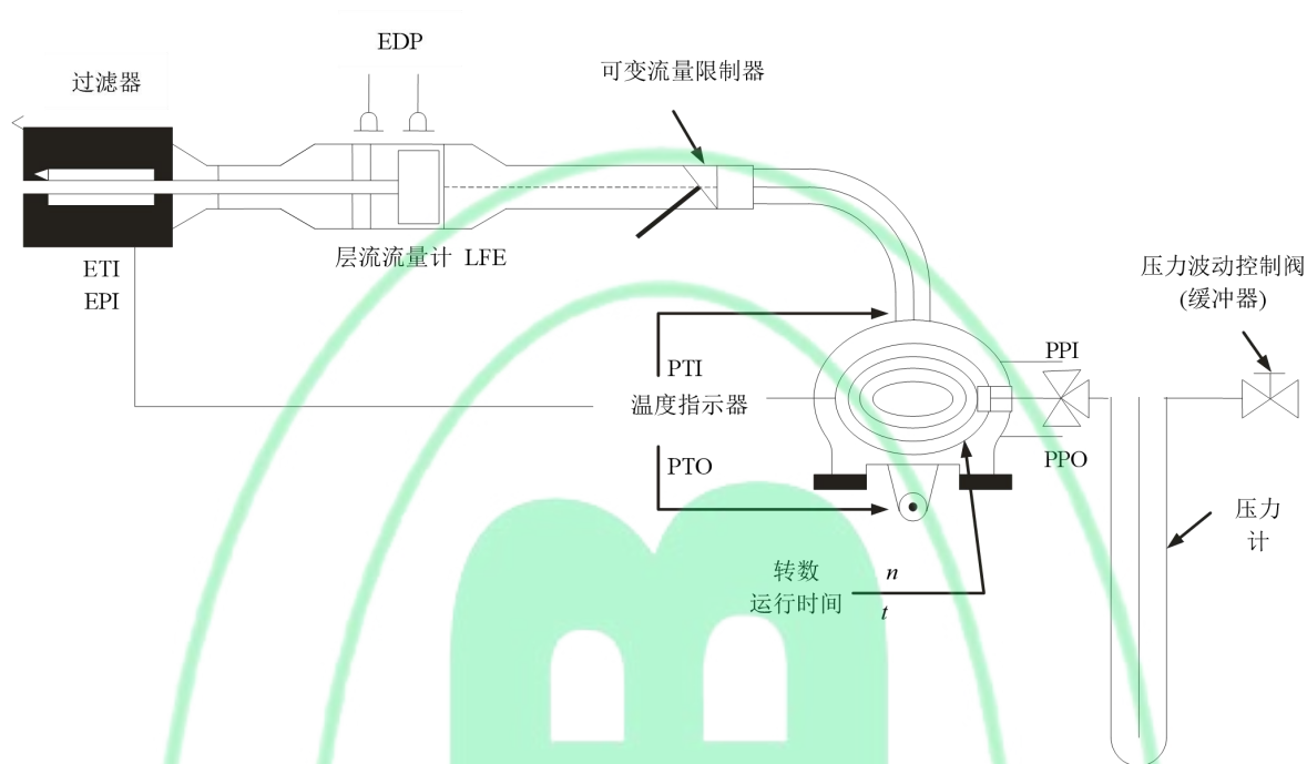
图 CD.6 PDP 标定布置图
