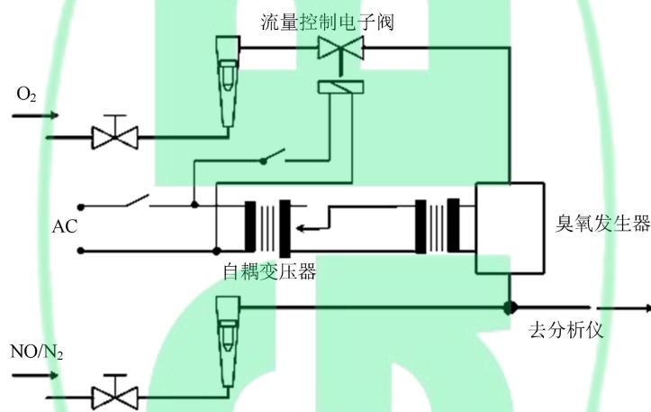
图 CD.15 \text{NO}_x 转换器效率试验装置
