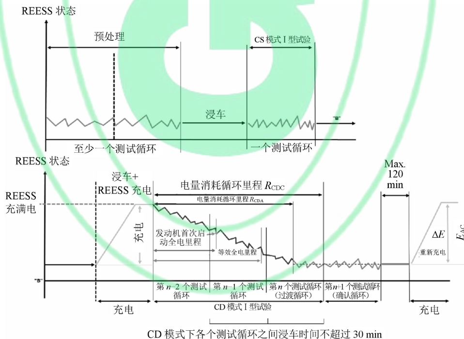
图 RA.4 电量保持 I 型试验和电量消耗 I 型试验
