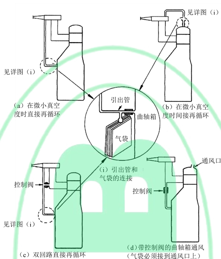
图 E.1 III 型试验
