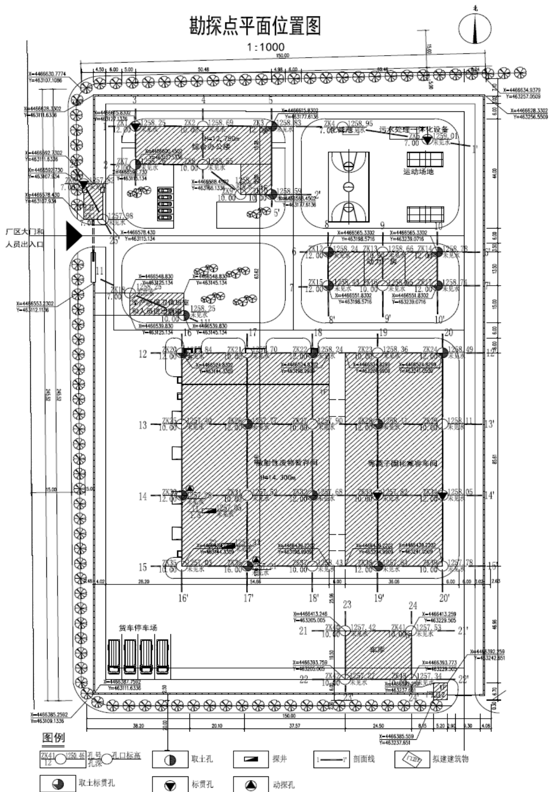
图 2.15 勘探点布置
