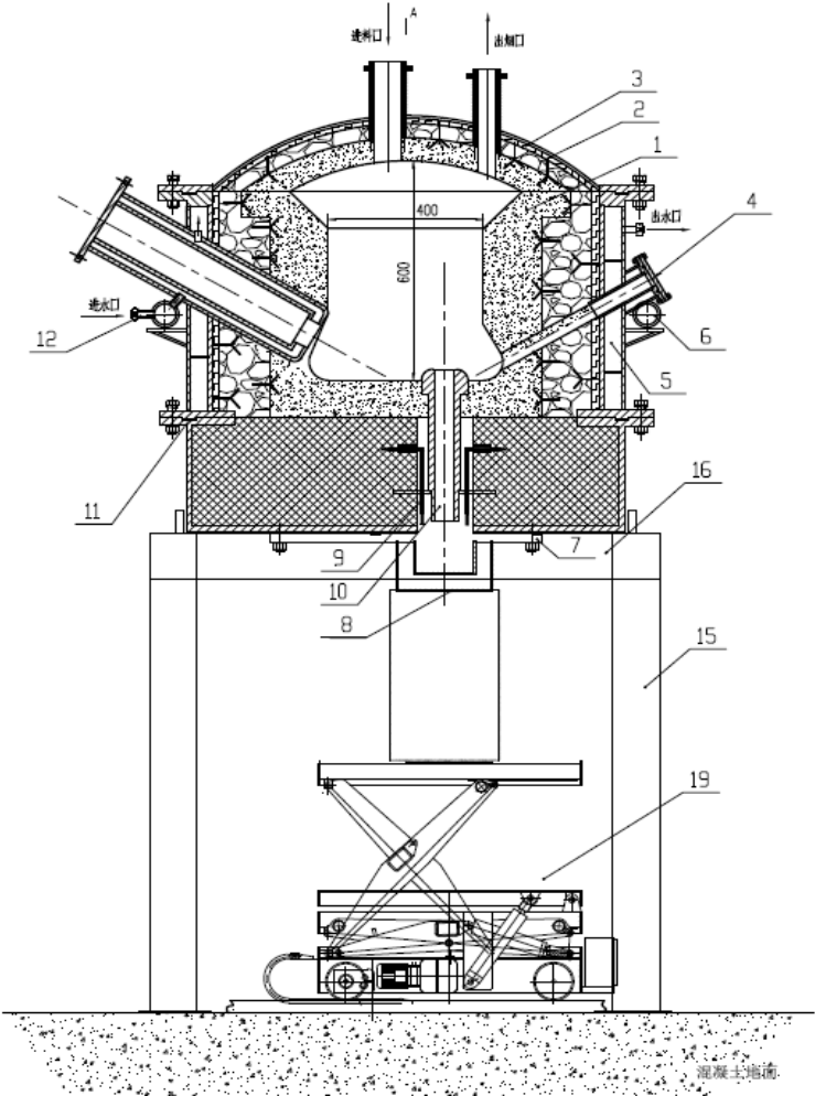
图 3.11 等离子熔融炉简图
