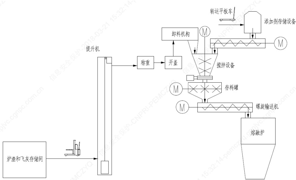
图 3.3 熔融炉预处理和进料系统流程图
