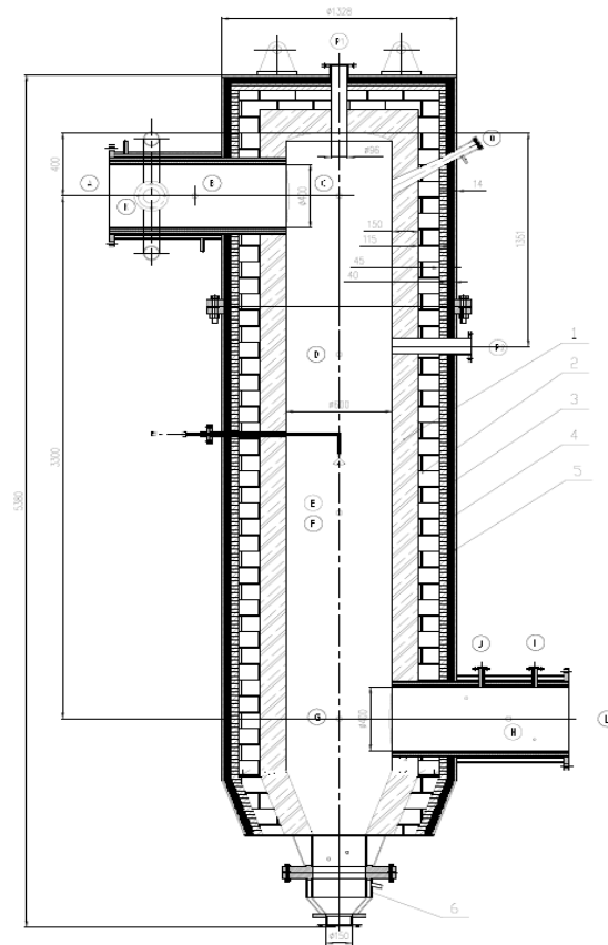
图 3.10 二燃室简图
