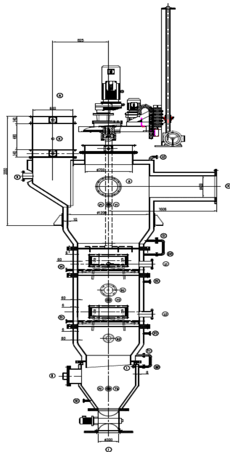
图 3.9 气化炉简图
