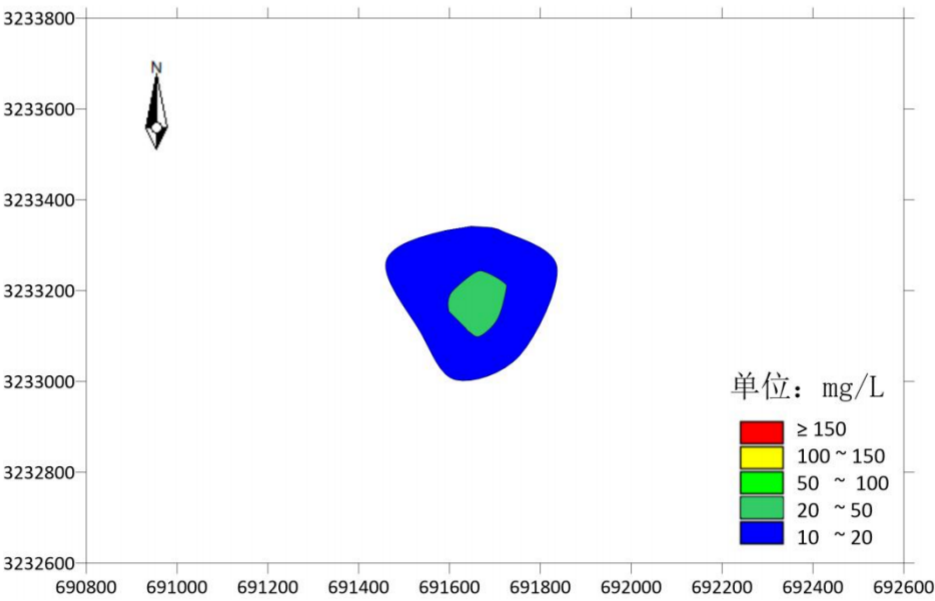
图 4.1 A 平台钻屑排放产生悬浮物的影响范围（表层）
