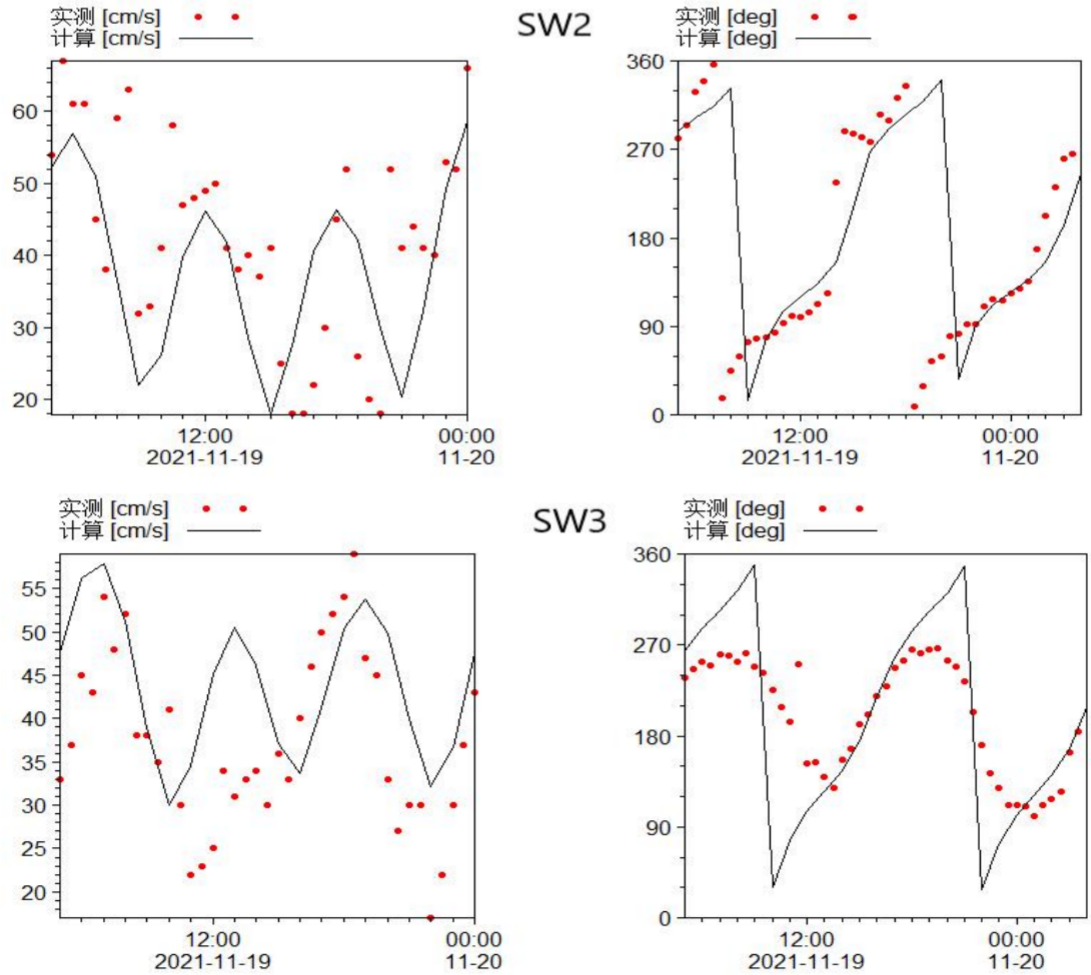
图 5 潮流验证曲线图（表层）
