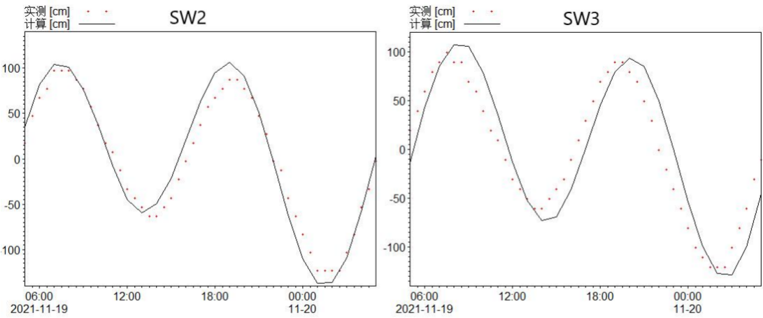
图 4 潮位验证曲线图
