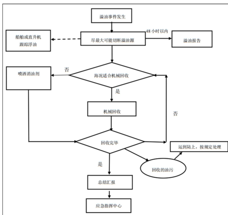
图 5.7 施工期-小型溢油事故应急反应程序
