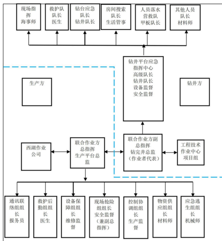
图 5.3 钻完井作业期间联合作业溢油应急组织机构示意图
