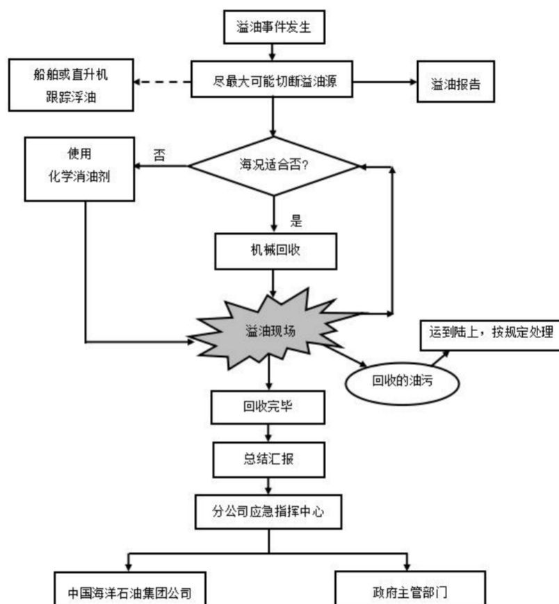
图 5.8 运营期-溢油事故应急反应程序
