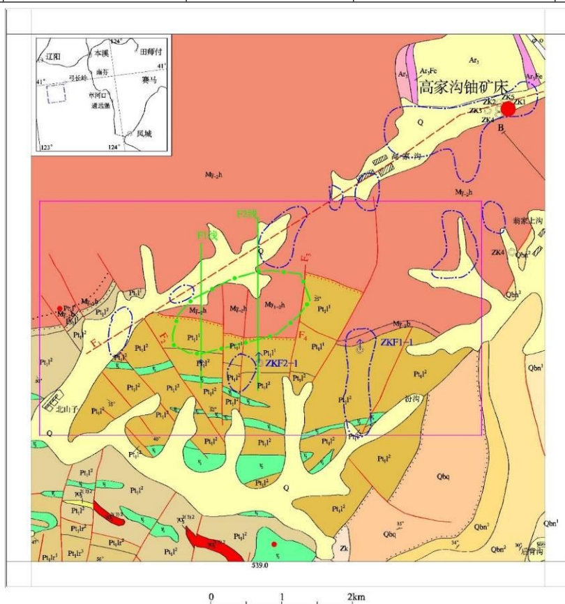
图 6-1 钻孔工程部署图
