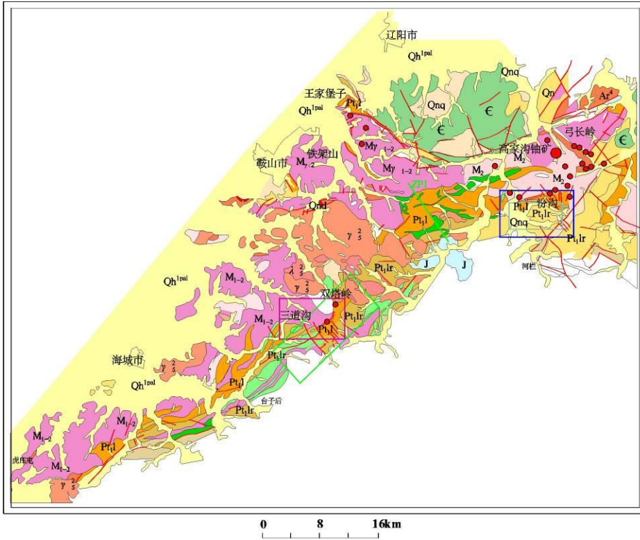
图 3-3 区域地质图
