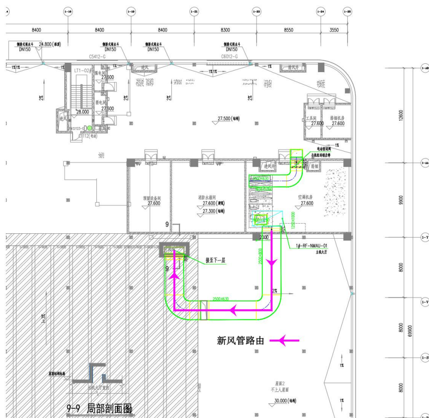
b) 主机车间屋面新风管路由 附图 10 主机车间新风管路由
