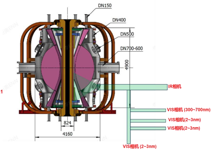
图 2-35 极向布局图
