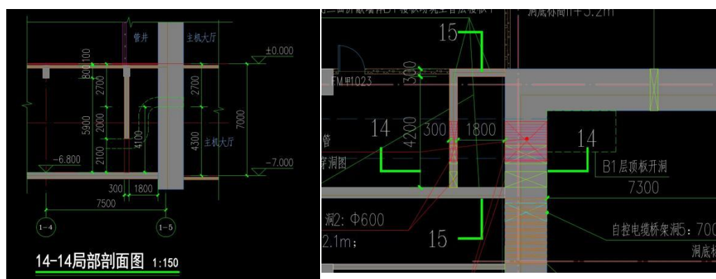
图 4-6 负一层工艺风洞迷道设计图
