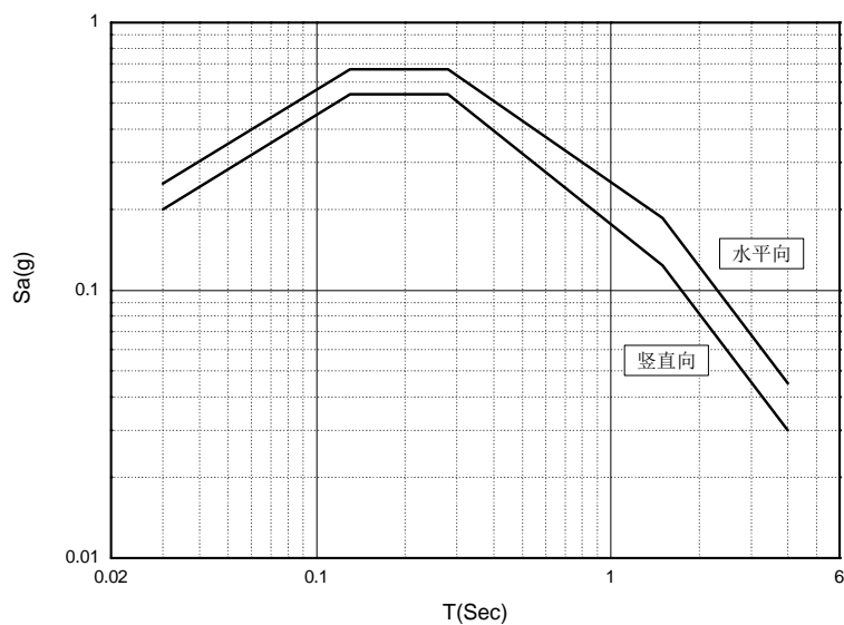
附图 场址特定 SL-2 级地面运动加速度反应谱 (5%阻尼比)
