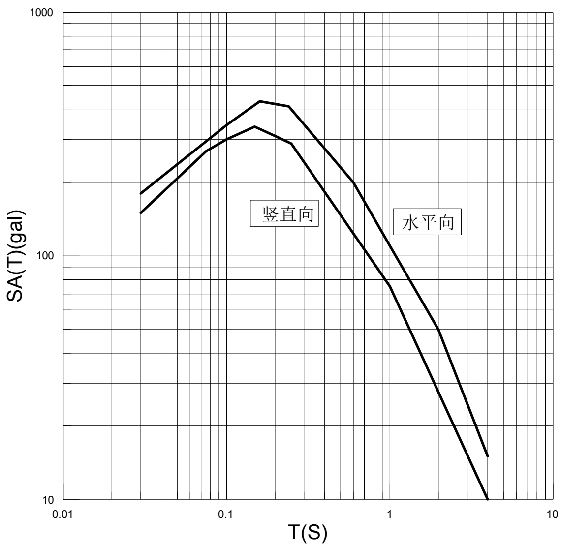
附图 1 厂址特定 SL-2 级地面运动基岩加速度反应谱 (5%阻尼比)
