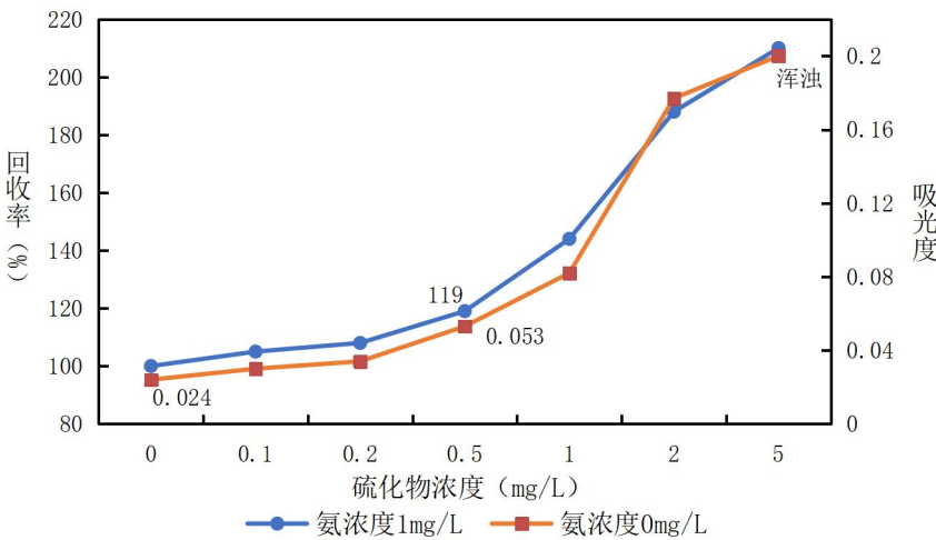
图 5-11 不同浓度硫化物对氨吸收液的影响 (n=3)
