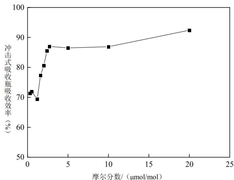
图 5-25 相同流量采集不同摩尔分数氨气吸收效率的对比
