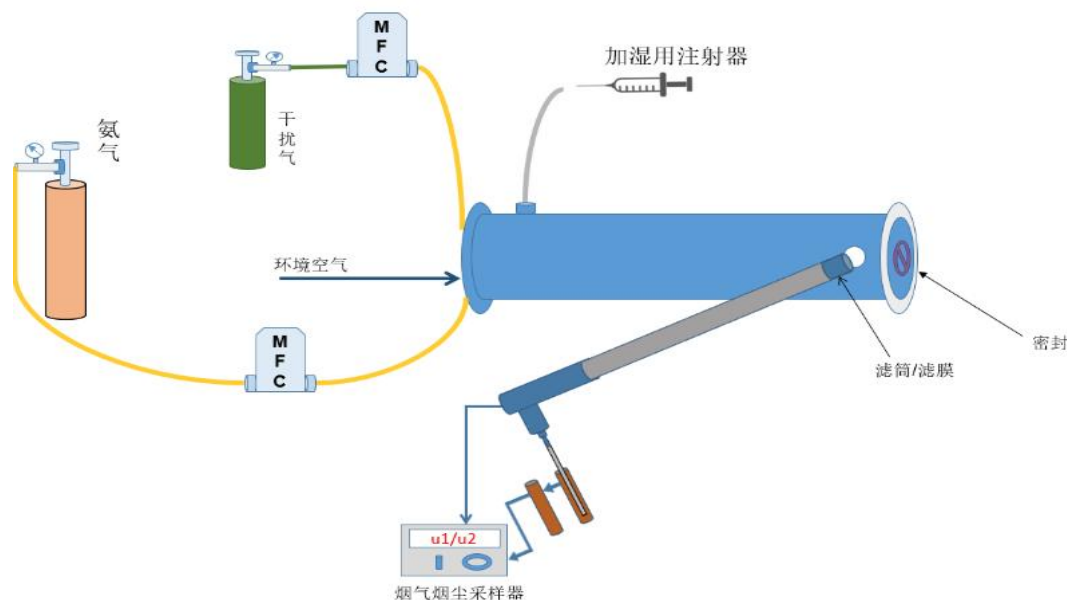
图 5-6 分流采样器干扰考察示意图
