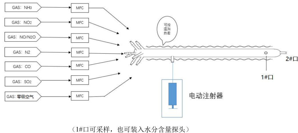
图 5-3 模拟烟道结构示意图
