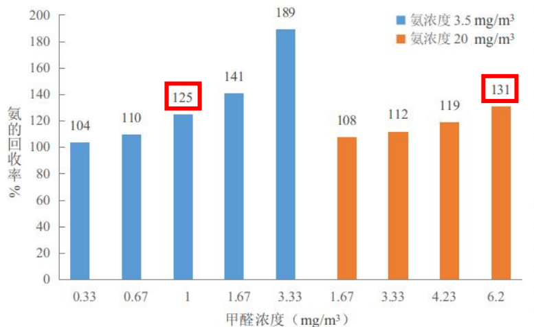
图 5-14 不同浓度甲醛对氨测定的影响 (n=3)
