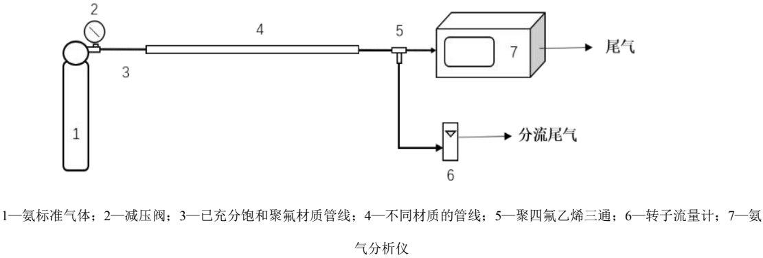
图 5-1 管线吸附性测试流路示意图
