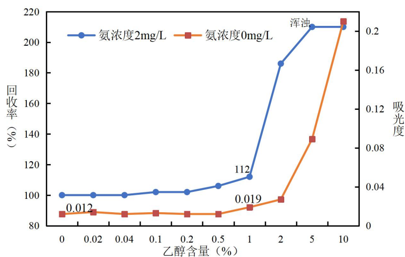
图 5-17 不同浓度的乙醇对氨吸收液的影响 (n=3)
