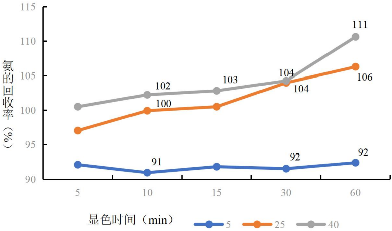
图 5-31 不同显色温度时间对氨测定的影响（ \text{HgCl}_2 纳氏试剂）
