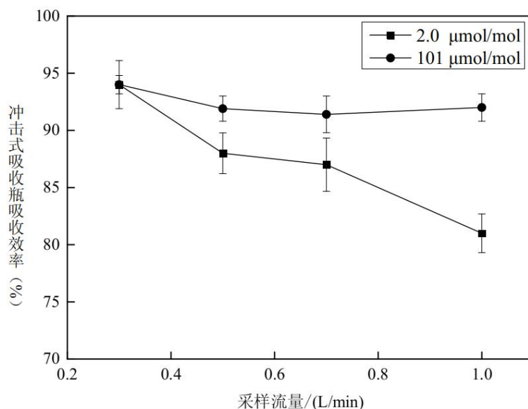
图 5-26 采样流量对不同摩尔分数样品吸收效率差异的对比
