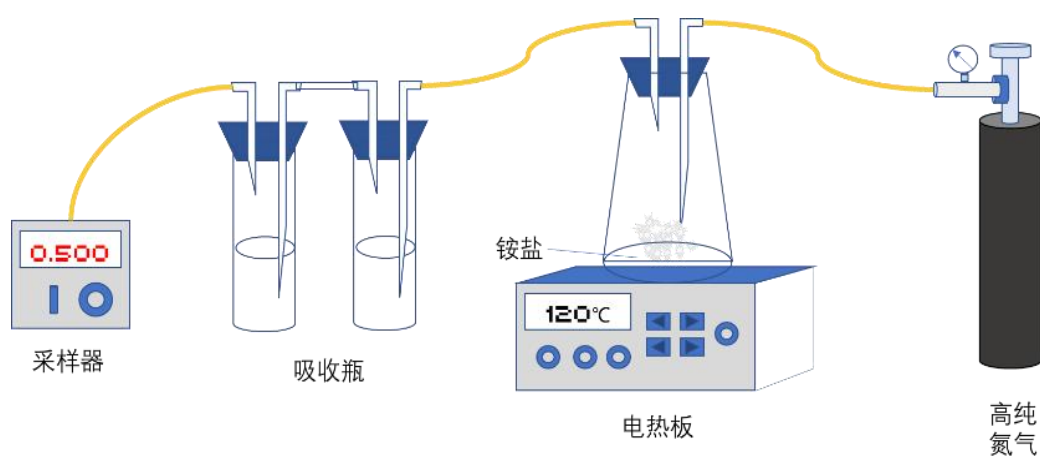
图 5-28 铵盐分解实验示意图
