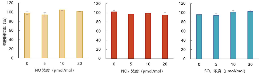
图 5-8 各干扰气体在分流采样时对氨回收率的影响 (n=3)
