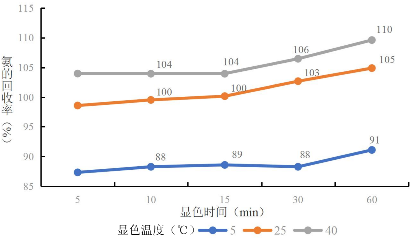
图 5-32 不同显色温度时间对氨测定的影响（ \text{HgI}_2 纳氏试剂）
