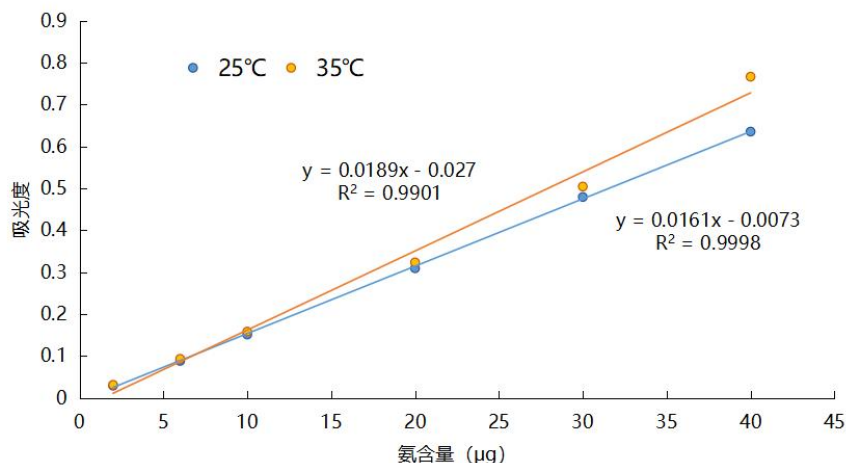
图 5-33 不同显色温度的曲线
