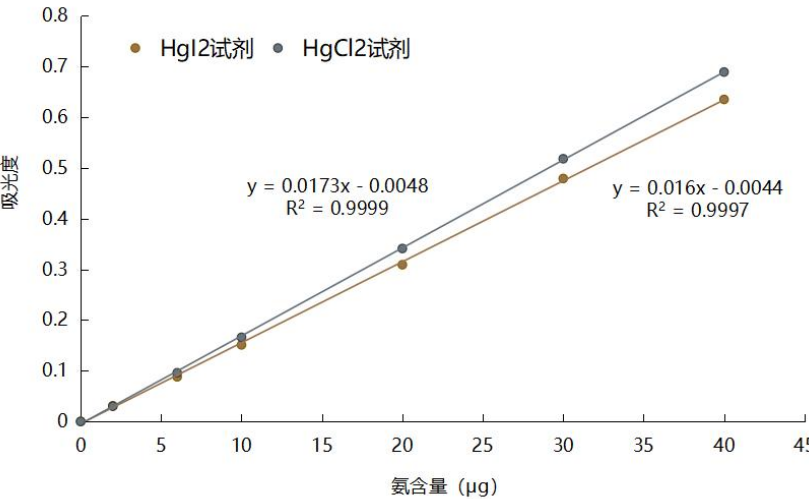
图 5-19 2 种纳氏试剂的校准曲线
