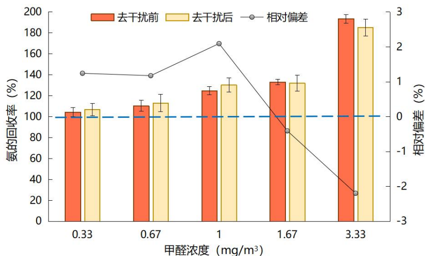
图 5-15 不同含量甲醛对氨测定的影响及去甲醛干扰效果 (n=3)
