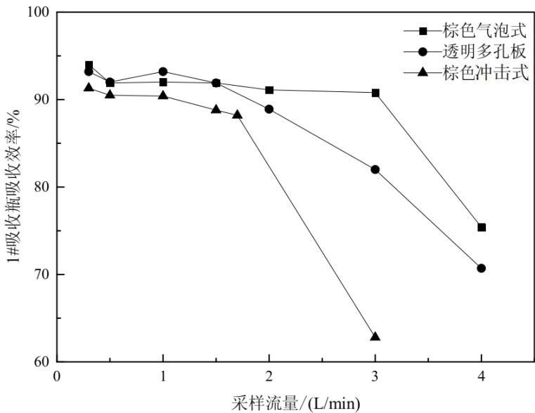
图 5-24 三种吸收瓶不同采样流量吸收效率的对比
