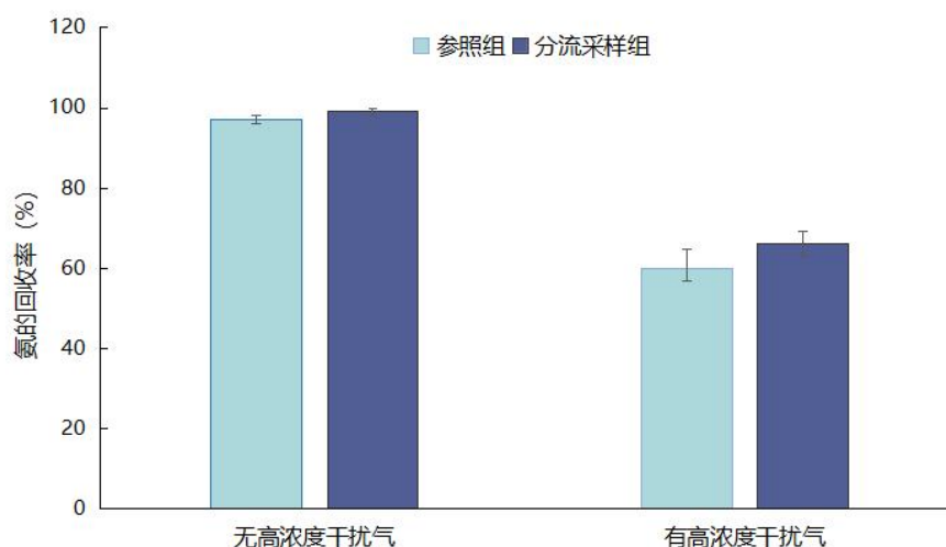
图 5-9 混合干扰气体在分流采样时对氨回收率的影响 (n=3)
