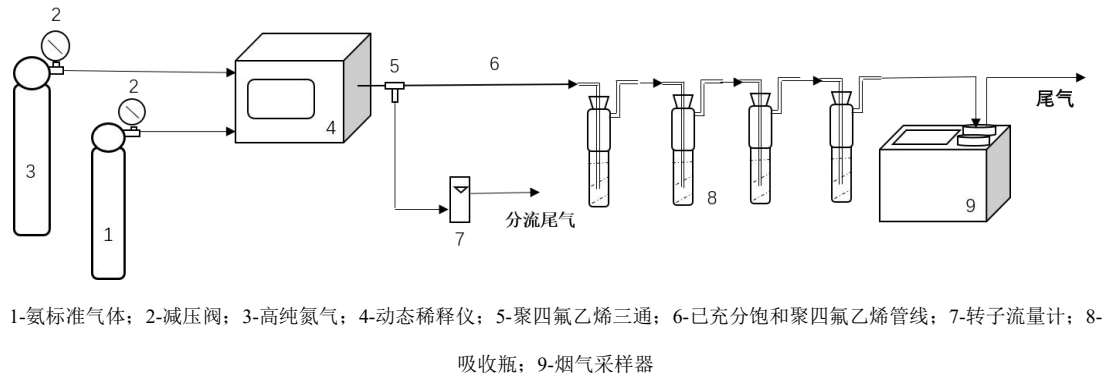
图 5-20 氨标准气体采样流程示意图
