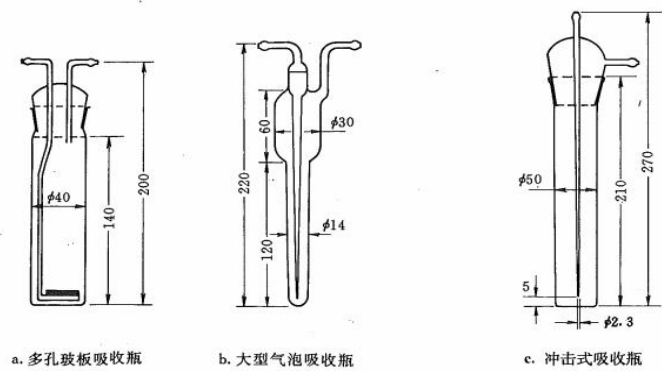
图 5-21 吸收瓶示意图
