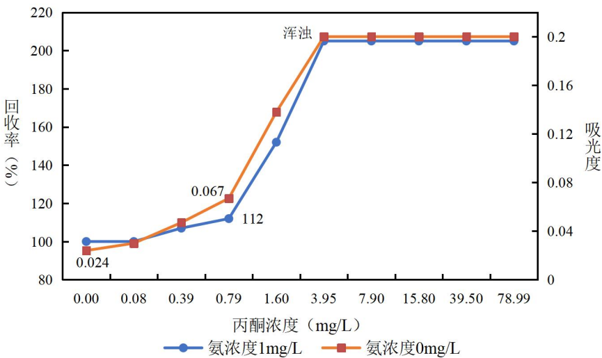
图 5-12 不同含量丙酮对氨吸收液的影响 (n=3)
