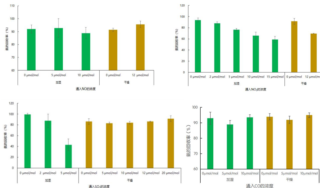
图 5-4 NO、NO 2 、SO 2 、CO 对氨回收率的影响 (n=3)
