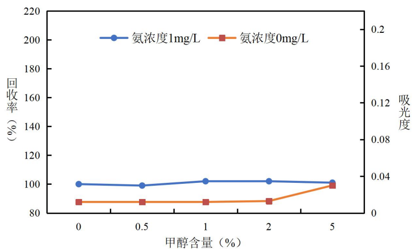
图 5-16 不同浓度的甲醇对氨吸收液的影响 (n=3)
