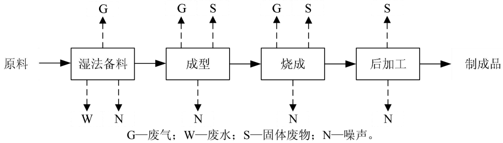
图 A.2 卫生陶瓷、日用及陈设艺术陶瓷和特种陶瓷典型生产工艺过程及污染物产生节点
