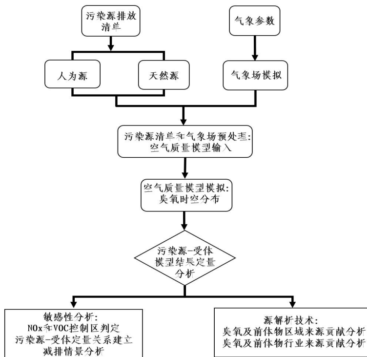
附图 2 基于空气质量模型来源解析技术流程
