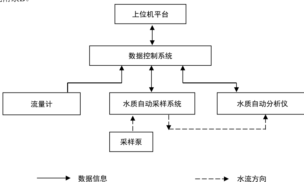
图2 数据控制系统示意图
