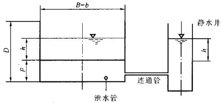
图 C.6 等宽薄壁堰构造示意图
