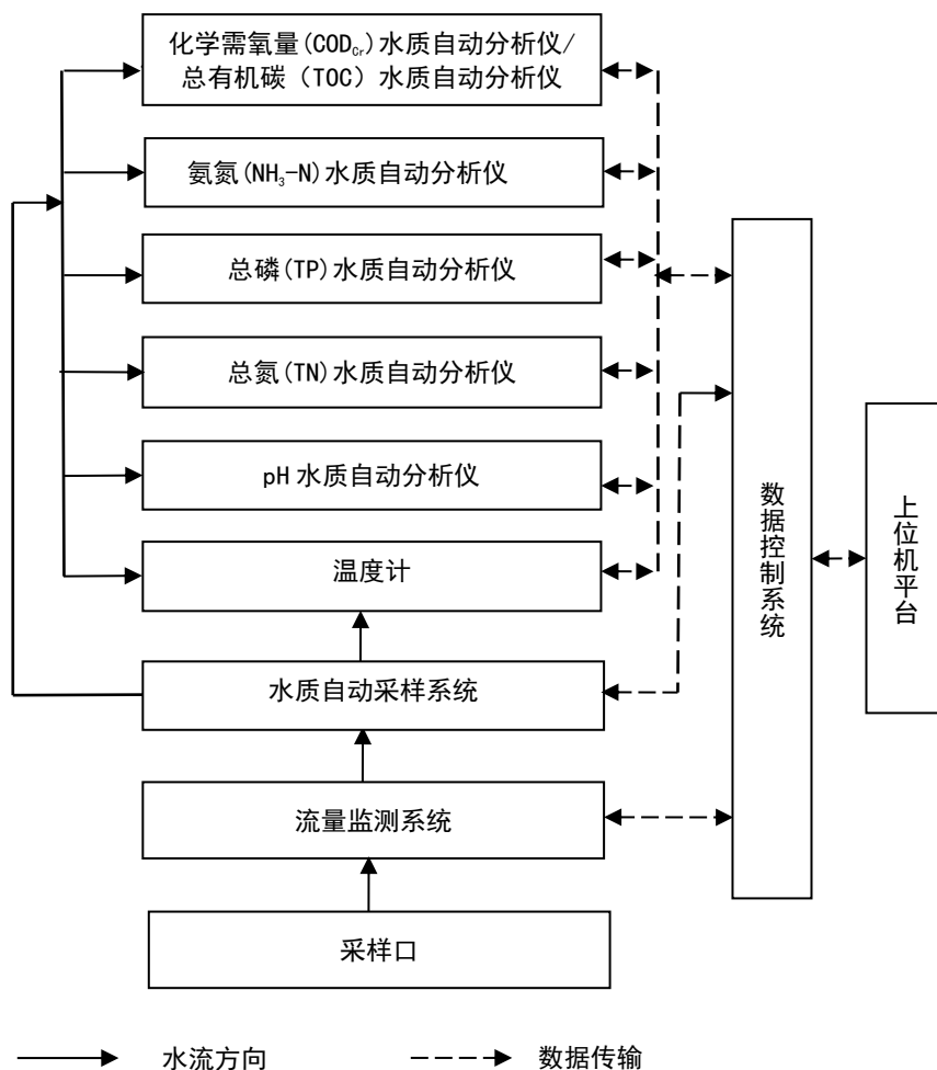
图 1 水污染源在线监测系统组成示意图
