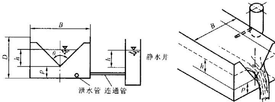
图 C. 4 三角形薄壁堰构造示意图
