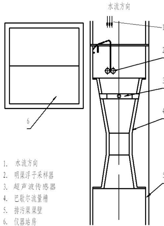
图C. 2 巴歇尔槽现场安装平面示意图
