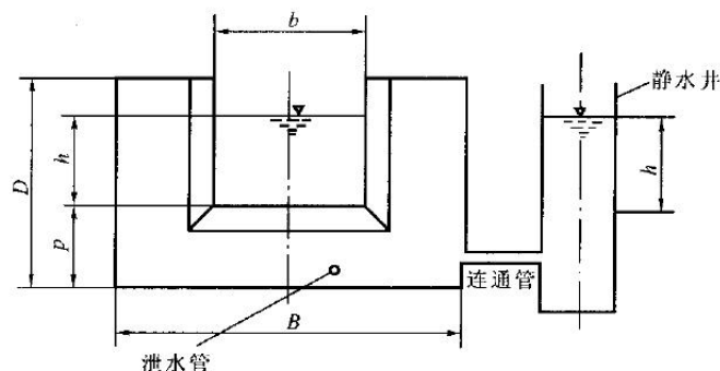
图 C. 5 矩形薄壁堰构造示意图
