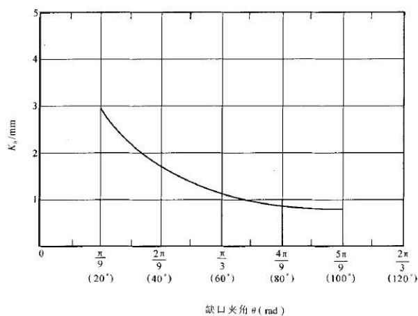
图 C.9 K_h 值和缺口夹角 \alpha 的关系曲线图
