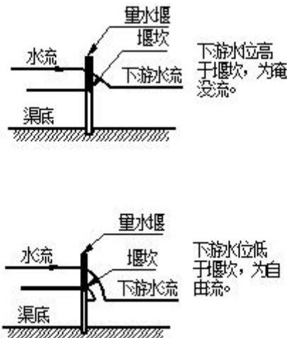
图 C. 12 自由流与淹没流
