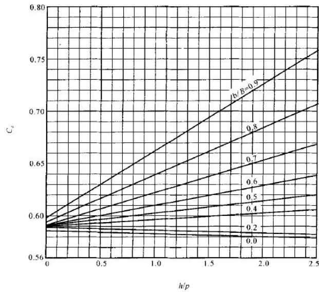
图 C.10 流量系数 C_e
