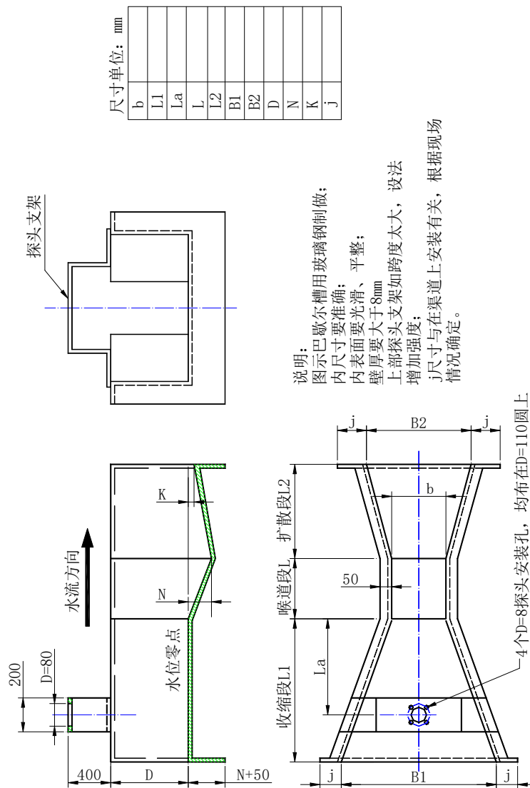
图 C.1 巴歇尔槽构造示意图
