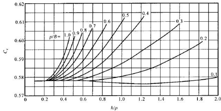
图 C.7 流量系数 C_e 图 ( \alpha=90^\circ )
