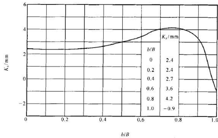
图 C.11 K_s 与 b/B 的关系曲线图
