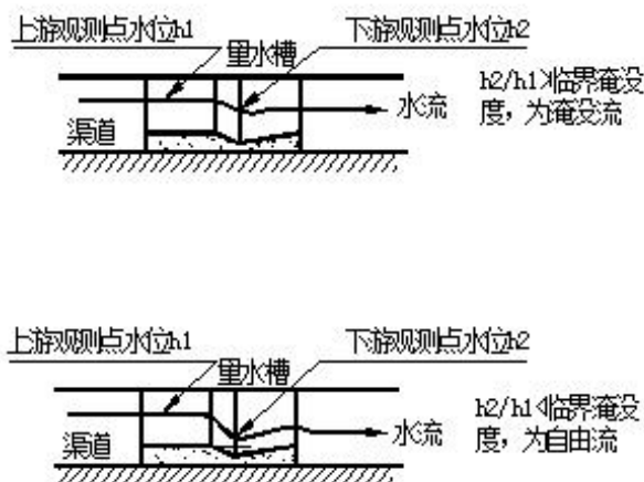
图 C. 3 自由流与淹没流
