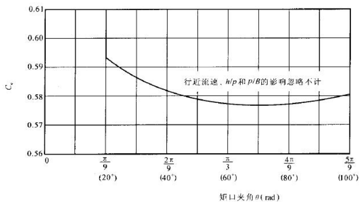
图 C.8 流量系数 C_e 和缺口夹角 \alpha 的关系曲线图
