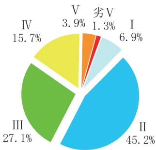
图 1-1 2026 年 6 月全国地表水水质类别比例
