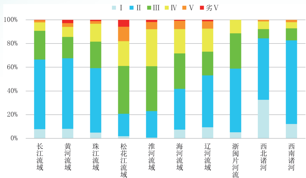
图 1-5 2026 年 6 月十大流域主要江河水质类别比例
