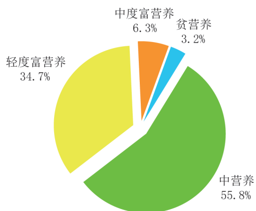
图 1-8 2026 年 6 月全国重要湖库营养状态比例
