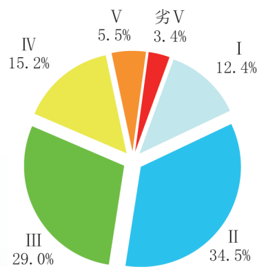
图 1-6 2026 年 6 月全国重要湖库水质类别比例
