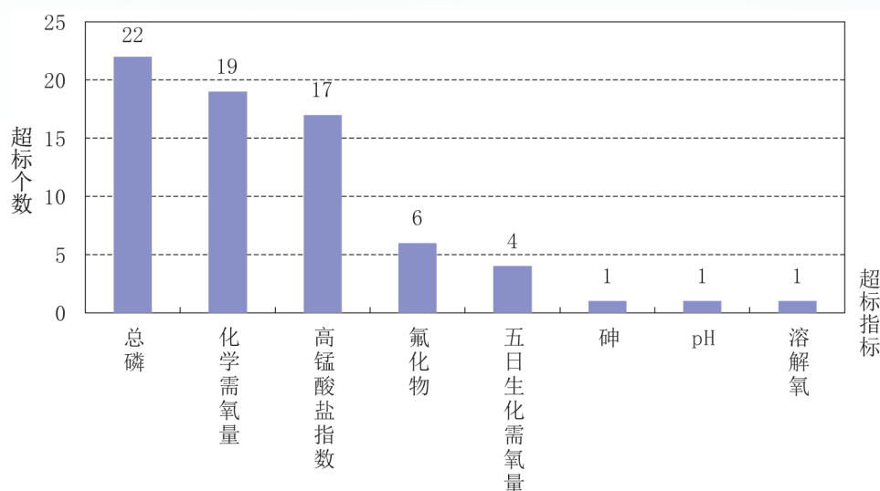
图 1-7 2026 年 6 月全国重要湖库超标指标统计
