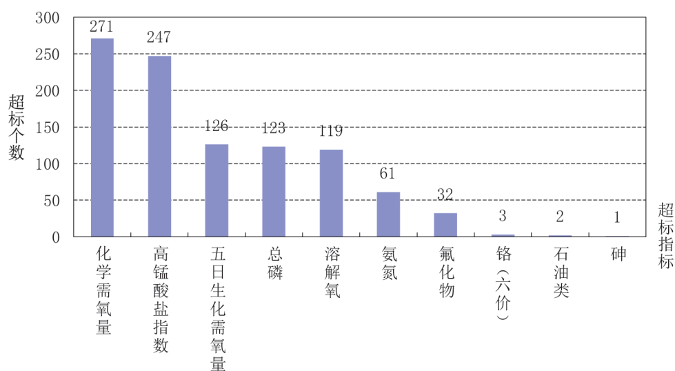
图 1-4 2026 年 6 月全国主要江河超标指标统计
