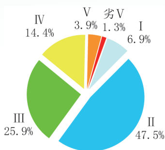
图 1-3 2026 年 6 月全国主要江河水质类别比例
