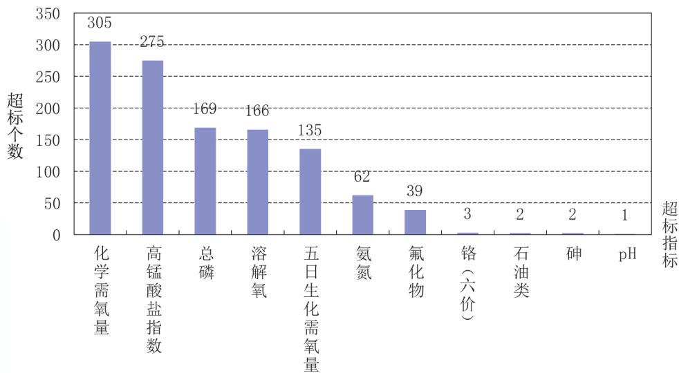
图 1-2 2026 年 6 月全国地表水超标指标统计
