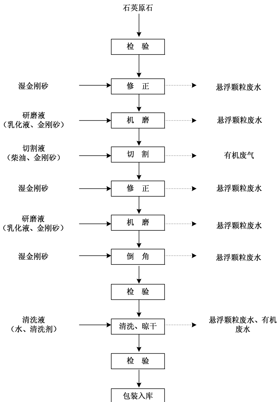
图 4-5 石英晶棒加工工艺流程及产污环节分析
