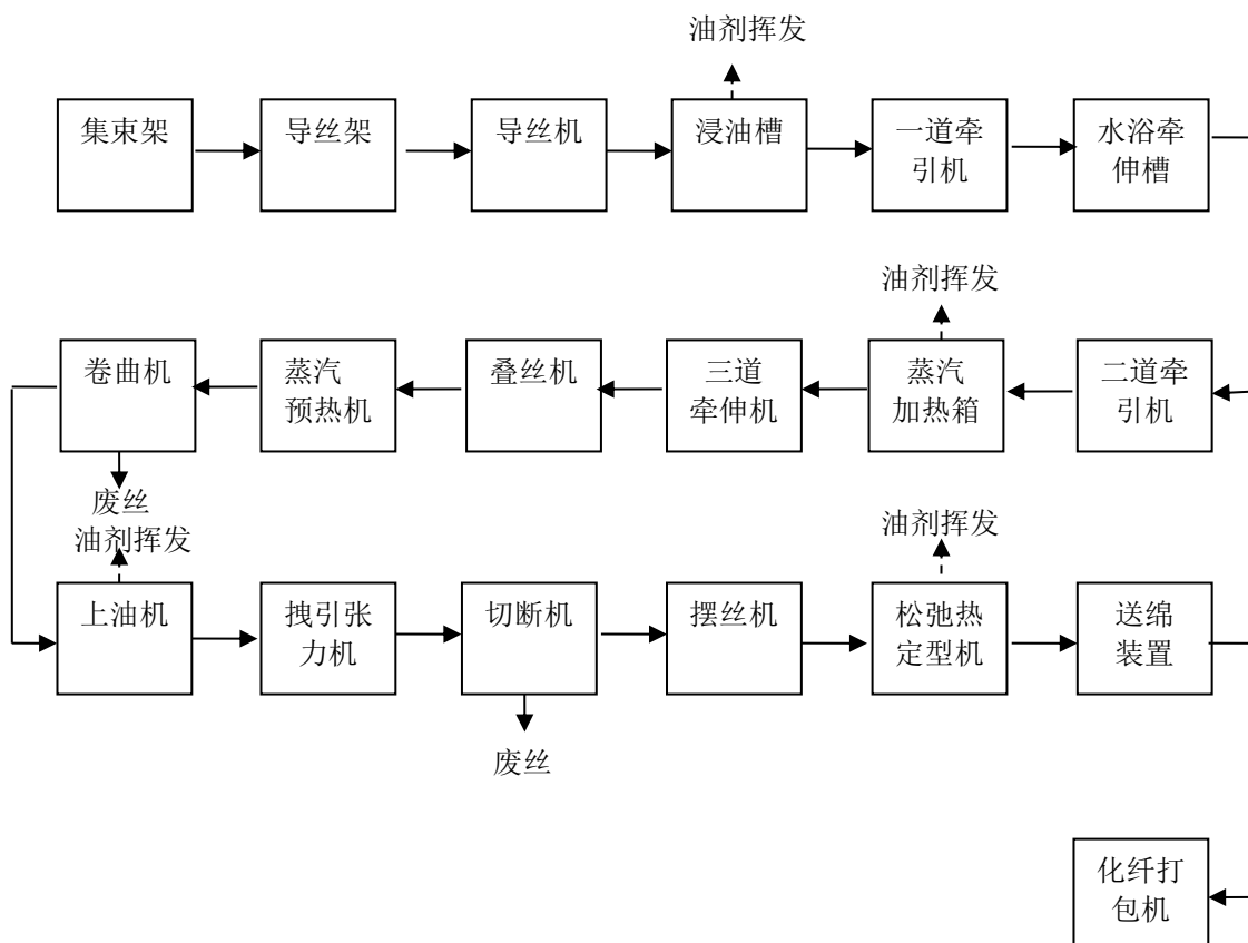
图 B.3 典型涤纶短纤维生产工艺流程示例图
