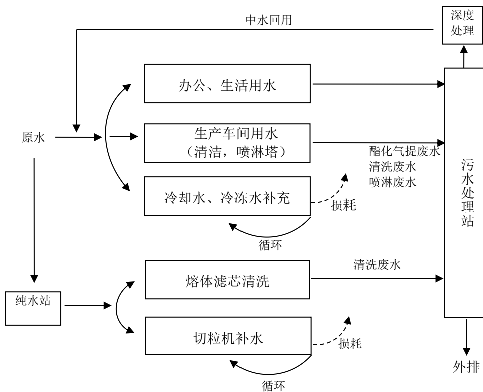
图 B.6 聚酯生产中用水、排水与水的循环使用示例图
