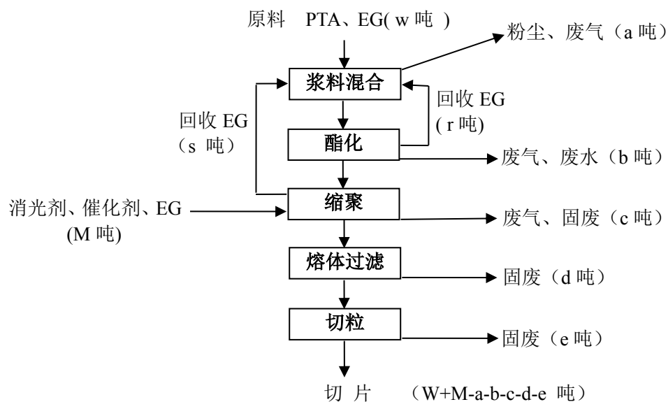
图 B.5 聚酯切片生产物料平衡示例图
