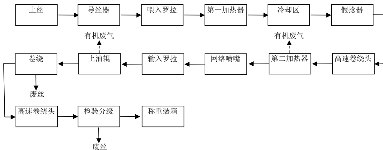
图 B.4 典型涤纶长丝生产工艺流程示例图
