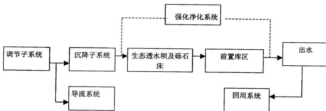
图7 平原河网地区面源污染强化净化前置库系统的结构示意图
