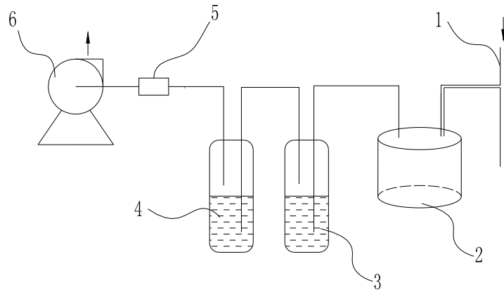
图 3-3 田间原位测定氨挥发的装置
