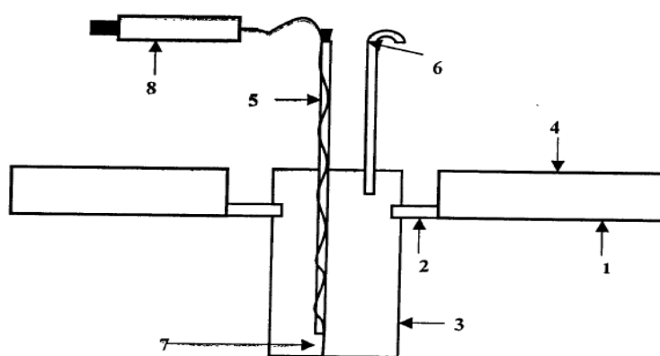
图中，1-集水槽、2-导水管、3-集水桶、4-渗水孔、5-出水管、6-通气管、7-抽水软管、8-抽气筒
