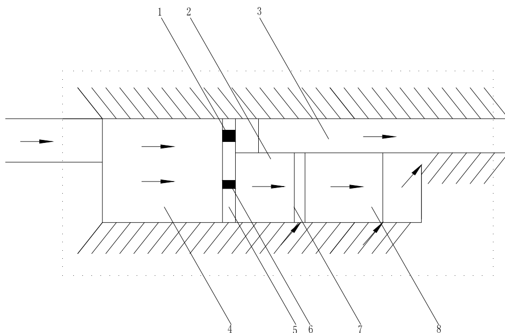
图中，1-泄洪闸、2-沉淀池、3-泄洪通道（生态沟渠）、4-径流收集与调节子系统（生态塘池）、5-拦水坝、6-控制闸、7-泄洪管、8-前置库库区
