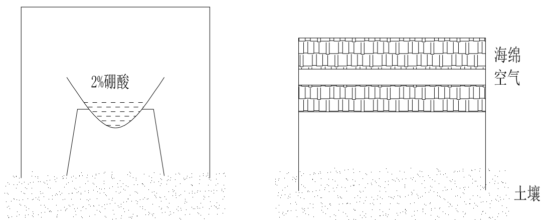
图 3-2 测定田间土壤氨挥发的密闭法 (A) 和通气法 (B) 装置
