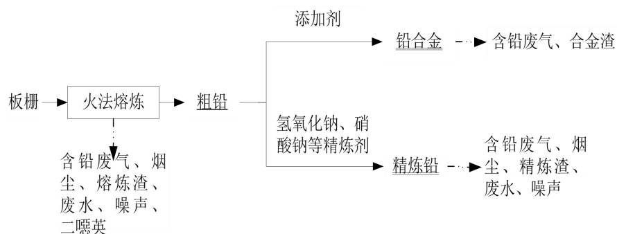
图3 预脱硫-还原熔炼-精炼工艺及产污环节——板栅熔铸、精炼
