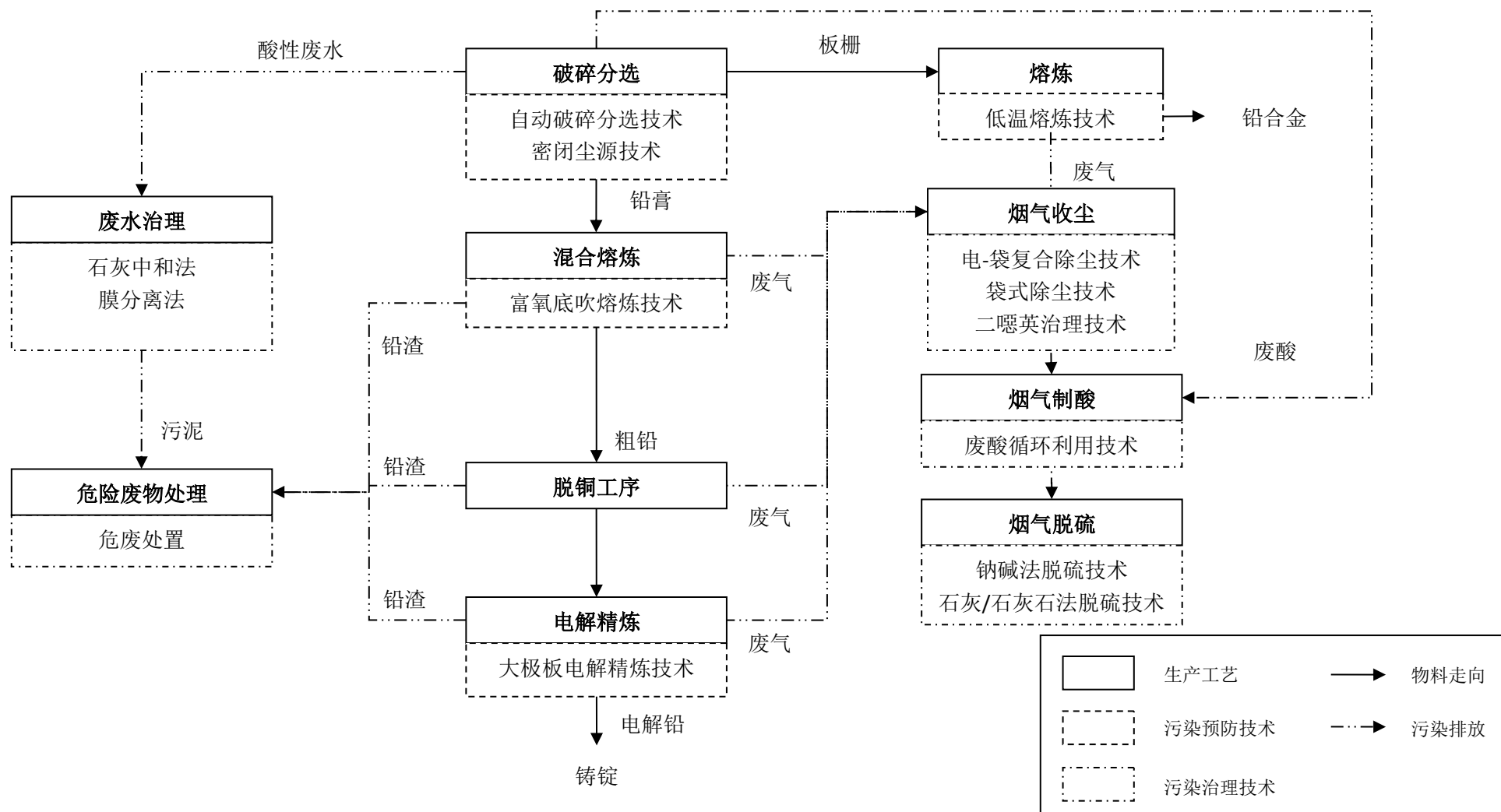
图 9 再生铅与矿产铅混合熔炼污染防治可行技术
