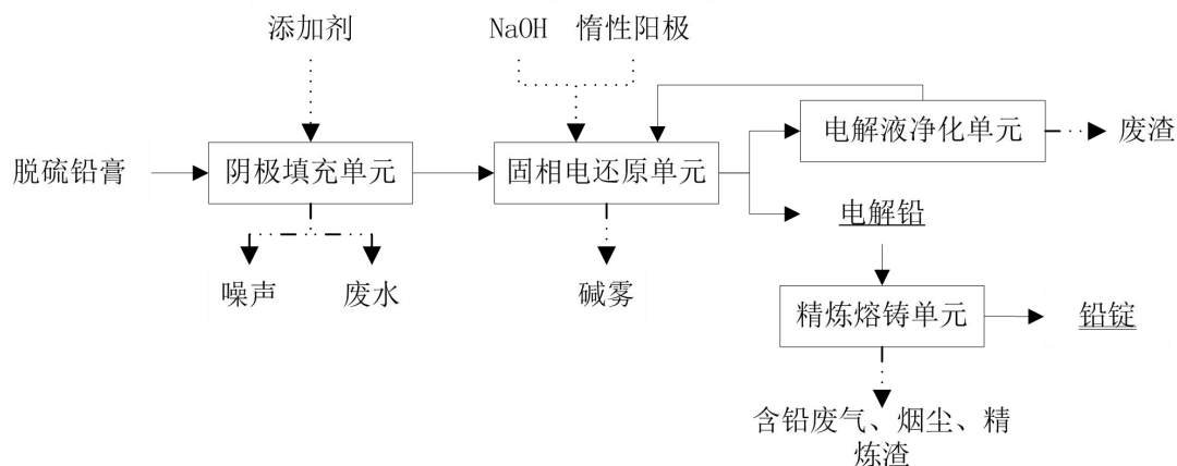
图 7 固相电还原工艺及产污环节
