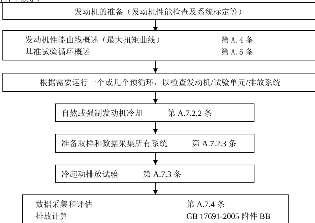
图 A.2 试验流程图
