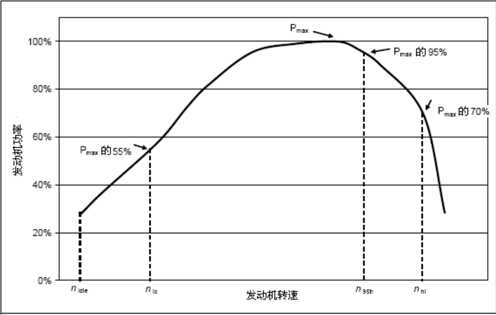
图 A.3 试验转速的定义
