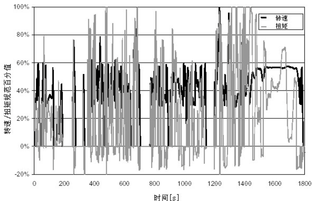
图 A.1 WHTC 试验循环
