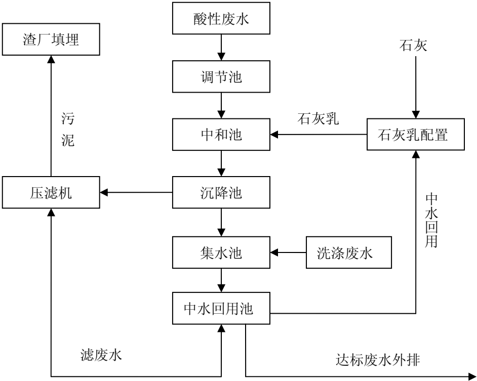
图 9 氯化法工艺生产废水处理流程图
