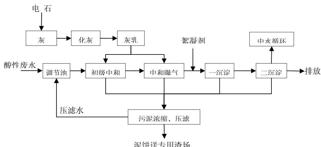
图 8 新建企业废水处理工艺流程图
