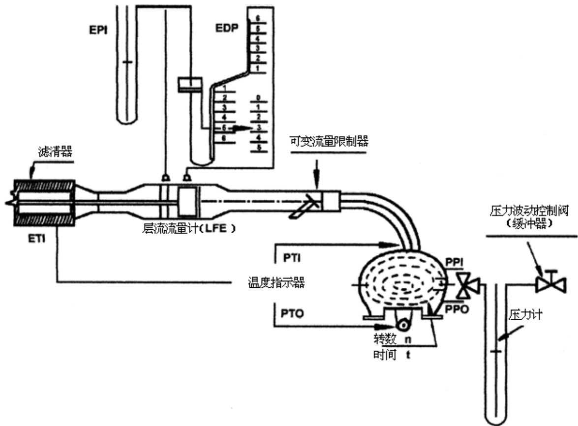
图 CC.3 PDP-CVS 标定布置图
