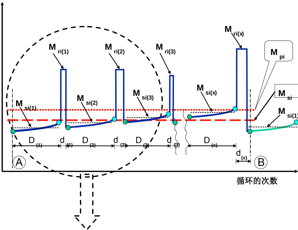
图P.2 在出现再生阶段的两循环之间以及再生时的参数测量（示意图）
