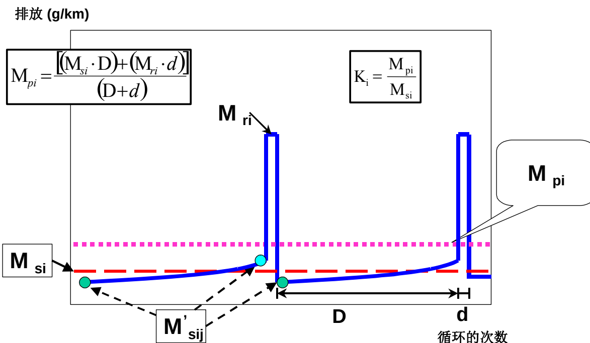
图P.1 在出现再生阶段的两循环之间以及再生时的参数测量 (示意图, “D”区间的排放可能增加或降低)
