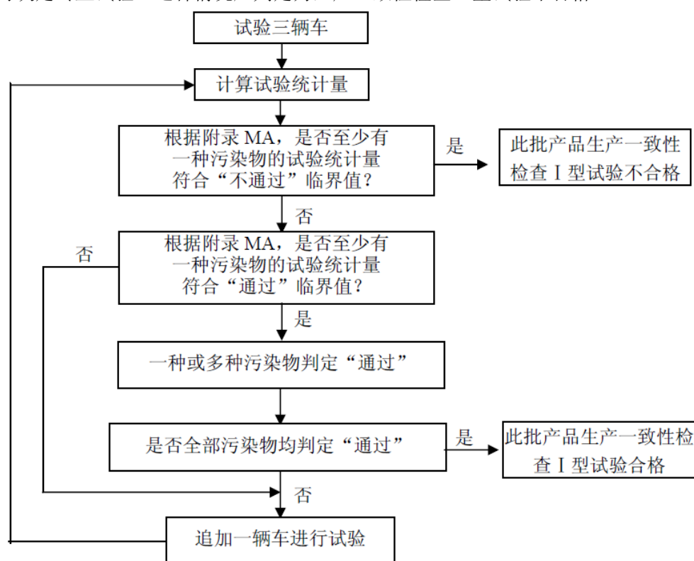
图 2 生产一致性检查 I 型试验流程图
