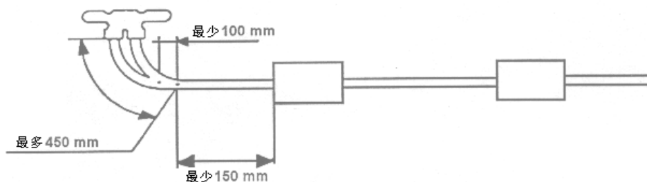
图L.2 背压 - 测量点 (2) (2)
