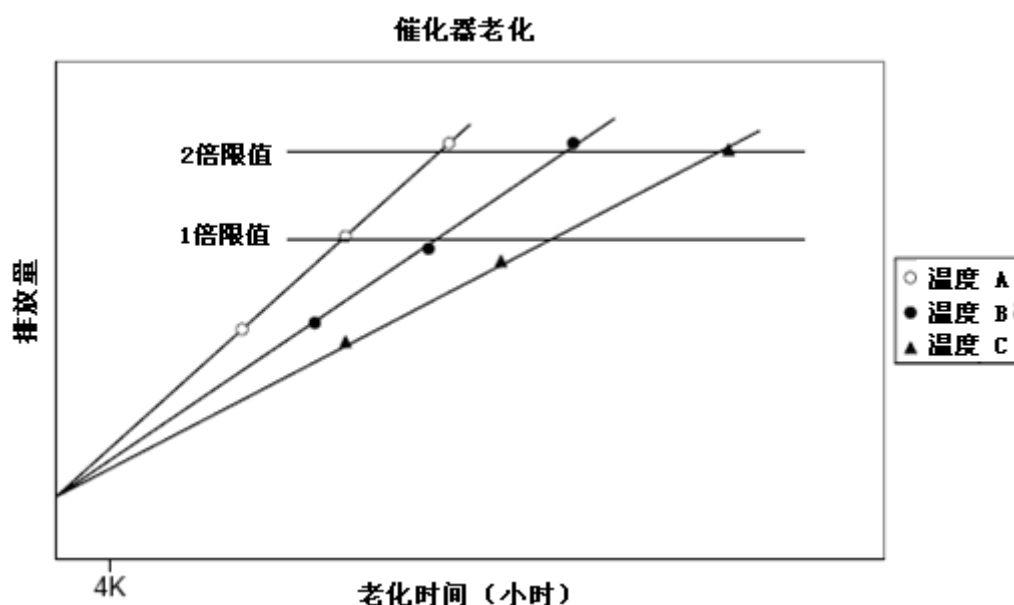
图GA.2 催化器老化与排放关系
