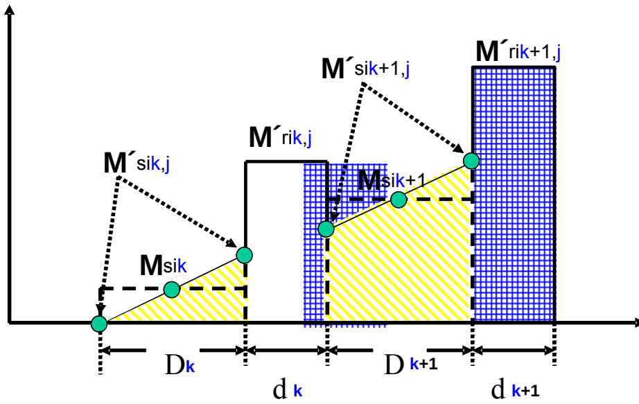
图 P.3 在出现再生阶段的两循环之间以及再生时的参数测量（示意图）
