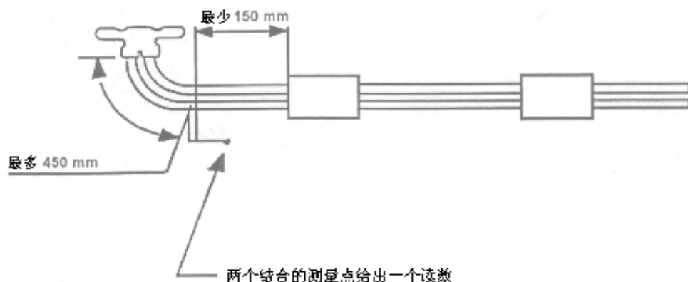
图L.3 背压 - 测量点 (3)
