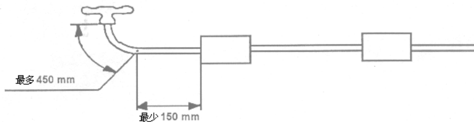
图L.1 背压 - 测量点 (1)
