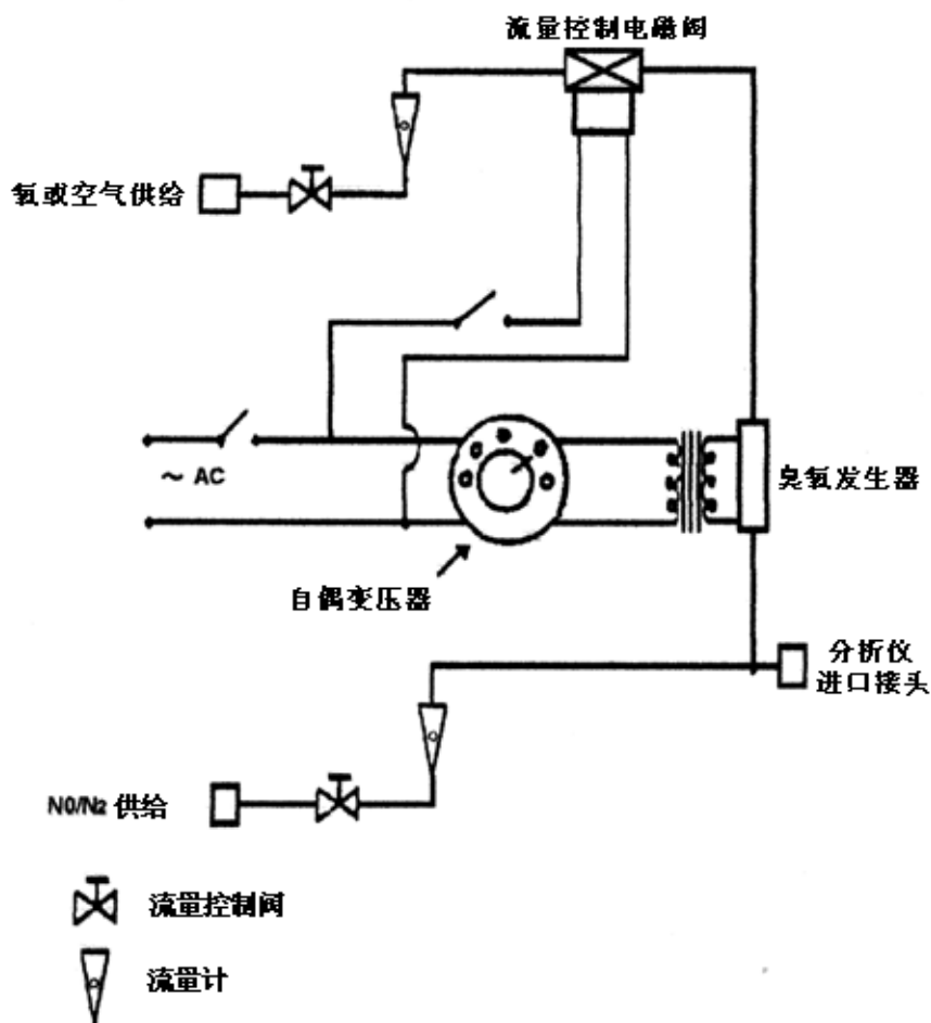
图 CD.2 NO x 转化器效率装置简图
