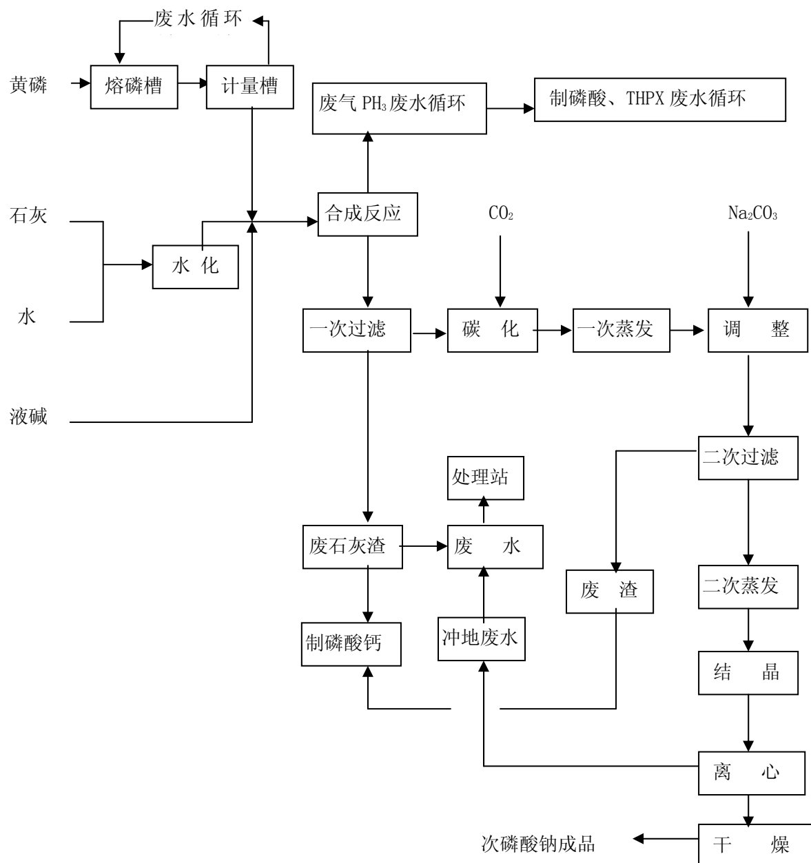
图 18 次磷酸钠生产工艺流程图示意图
