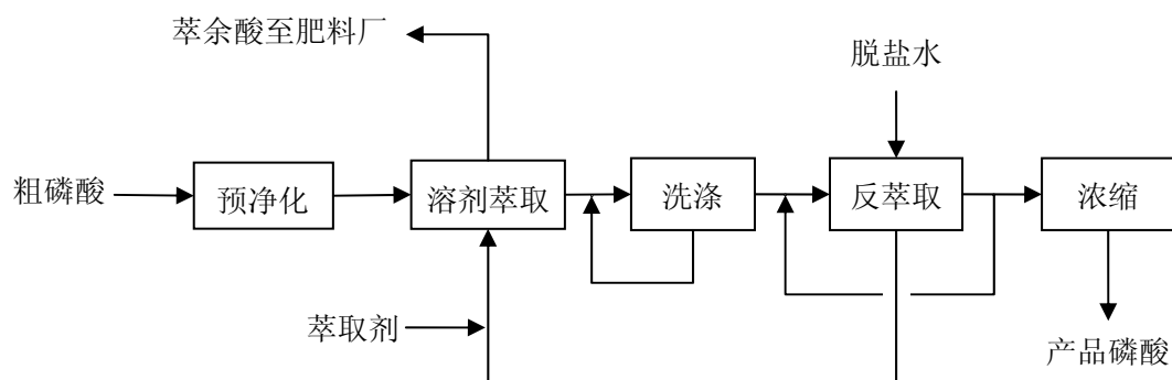
图 11 湿法磷酸精制工艺流程图
