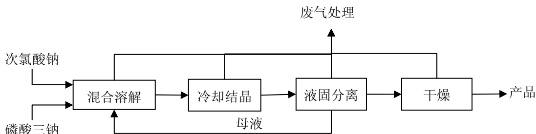
图 20 氯化磷酸三钠生产工艺流程示意图
