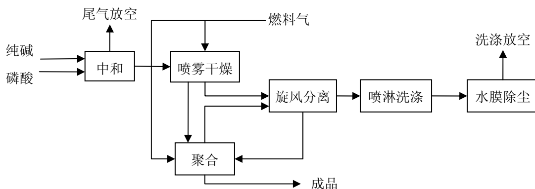
图 16 三聚磷酸钠工艺流程示意图(二步法)
