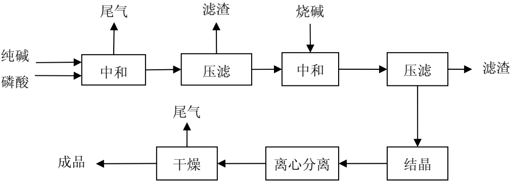
图 14 磷酸三钠生产工艺流程图
