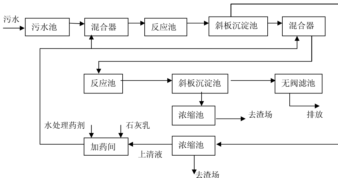
图 24 二级中和、二级沉淀加无阀过滤池处理流程
