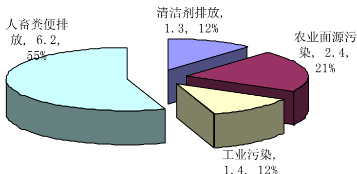
图 9 水体中磷元素来源(2000 年) (单位: 10 5 吨)
