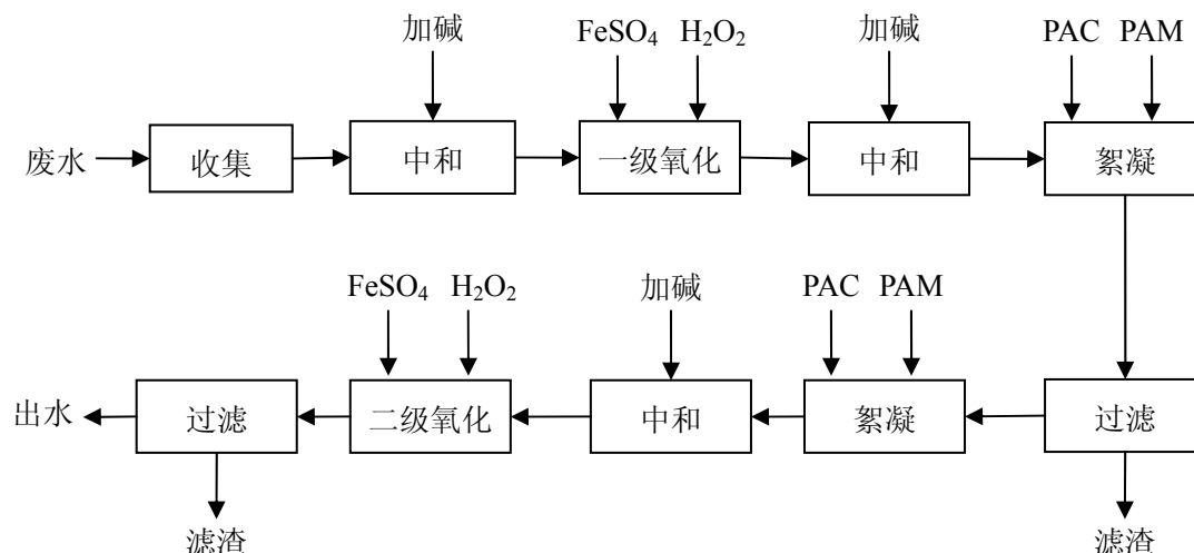
图 27 次磷酸钠废水处理流程简图
