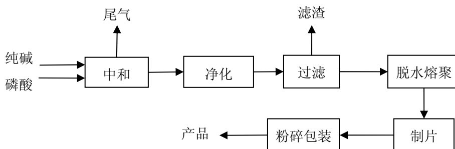
图 17 六偏磷酸钠生产工艺示意图
