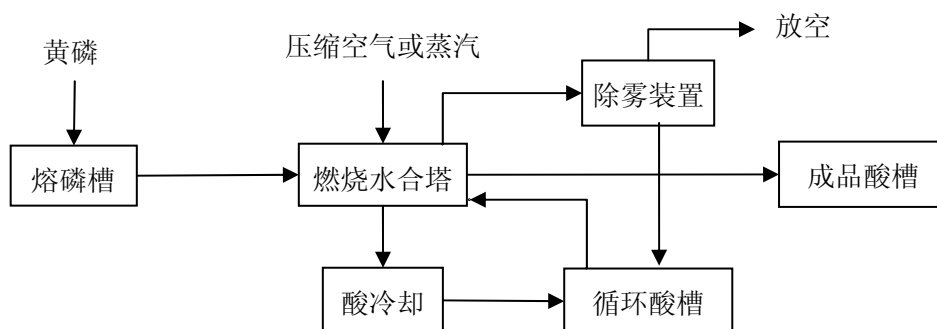
图 10 热法磷酸(一步法)生产工艺流程及产污节点图
