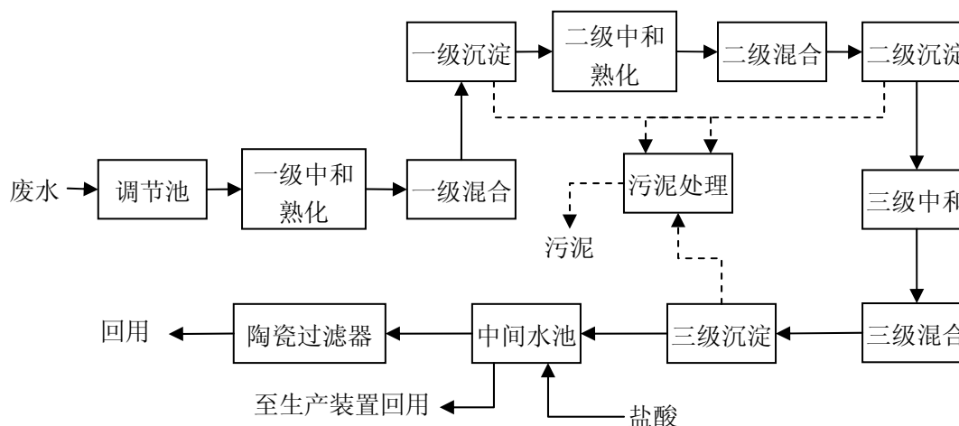
图 26 三级中和、三级沉淀、一级过滤废水处理流程简图
