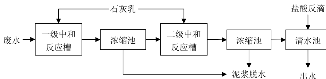
图 25 二级石灰乳过量—盐酸反滴法废水处理流程简图
