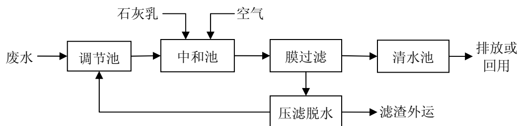
图 23 一级中和加一级膜过滤处理磷酸废水流程
