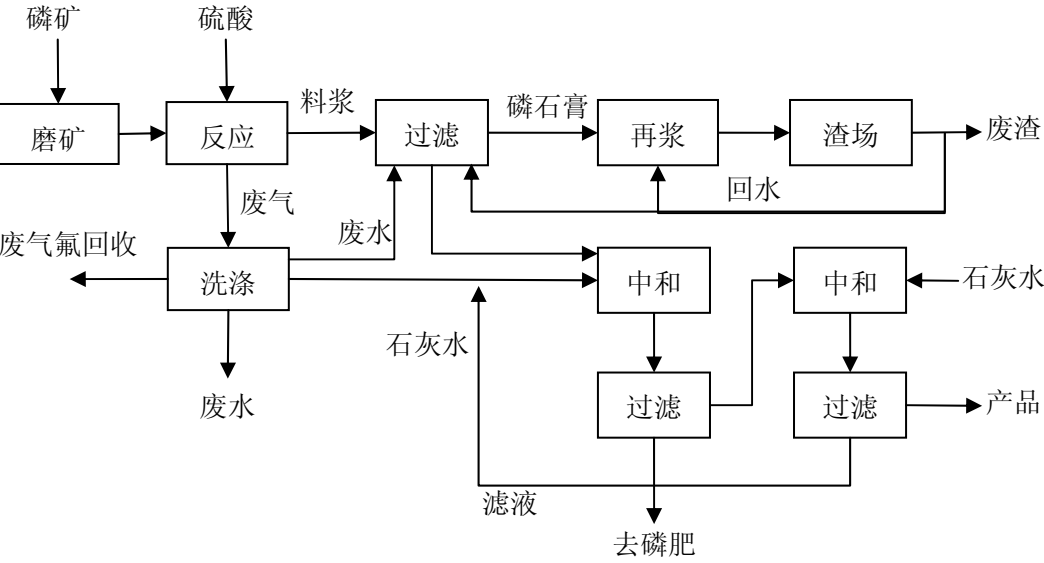
图 15 饲料磷酸氢钙工艺流程示意图
