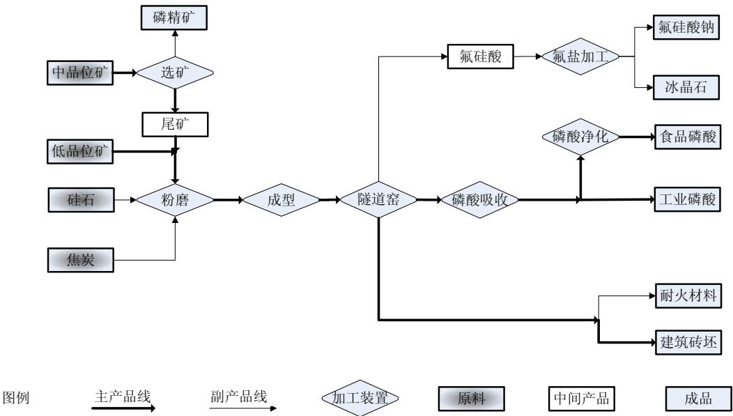
图 12 隧道窑法磷酸生产工艺示意图
