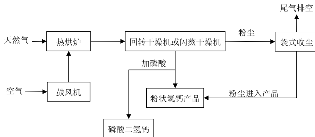
图 28 饲料磷酸钙产品烘干粉尘处理流程简图
