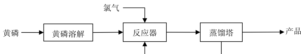
图 22 三氯化磷生产工艺简图
