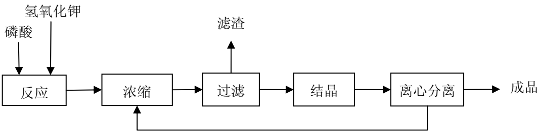
图 13 磷酸二氢钾生产工艺流程图（中和法）
