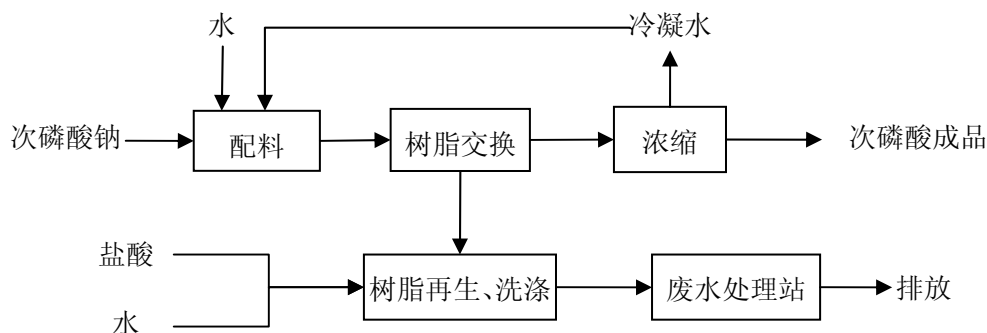
图 19 次磷酸生产工艺流程及产污节点图
