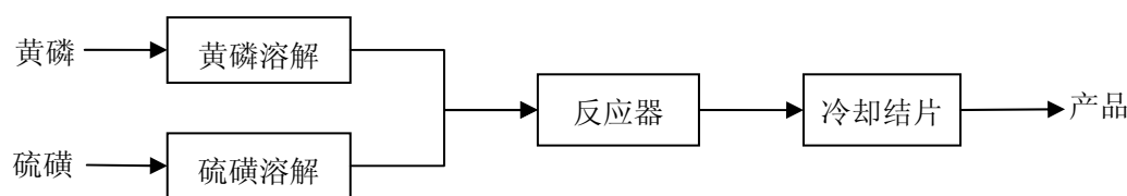
图 21 五硫化二磷生产工艺简图
