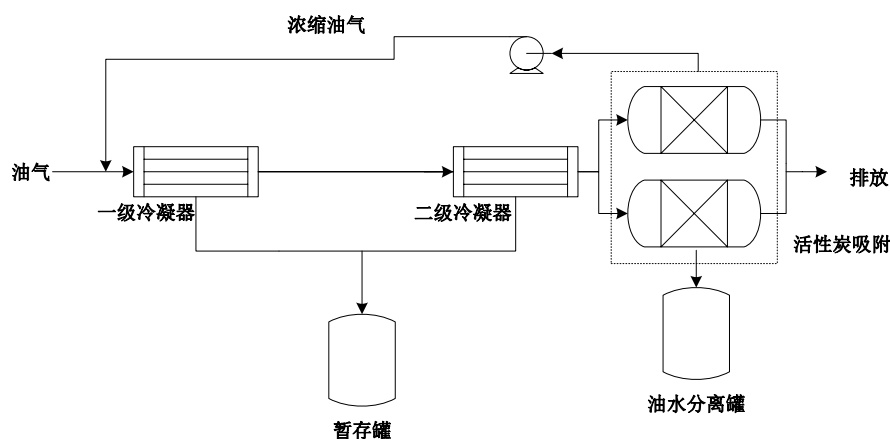
图 9.1-5 油气回收流程示意图
