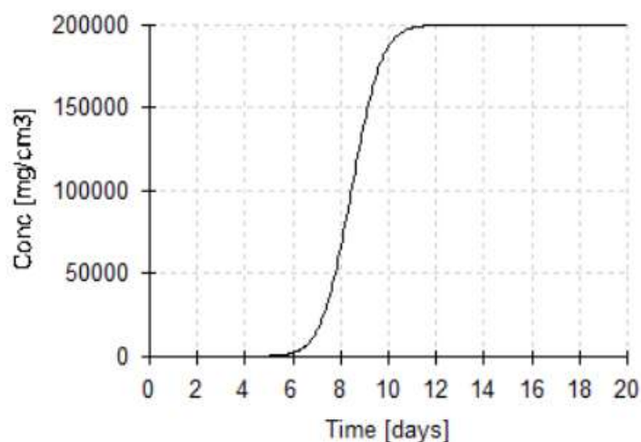
图 7.5-2 模型下边界（潜水面处）氨氮浓度变化曲线
