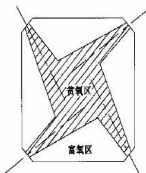
图 9.1-2 径向分级燃烧示意图
