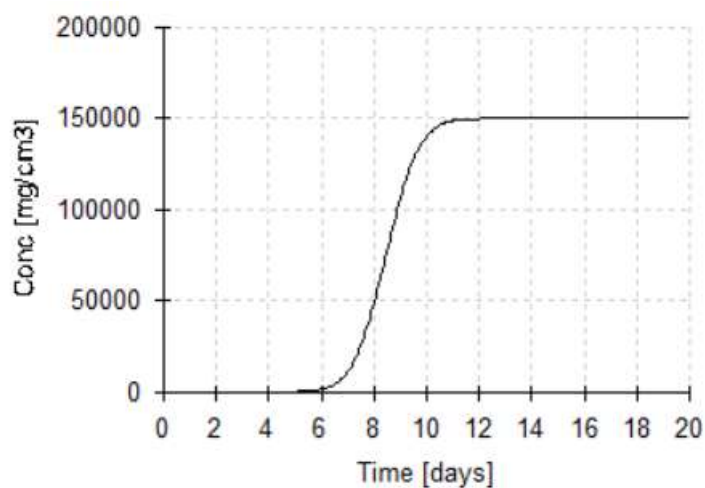
图 7.5-6 模型下边界（潜水面处）石油类浓度变化曲线
