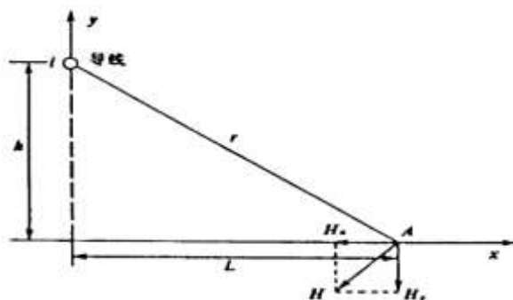
图 7.8-1 磁场向量图
