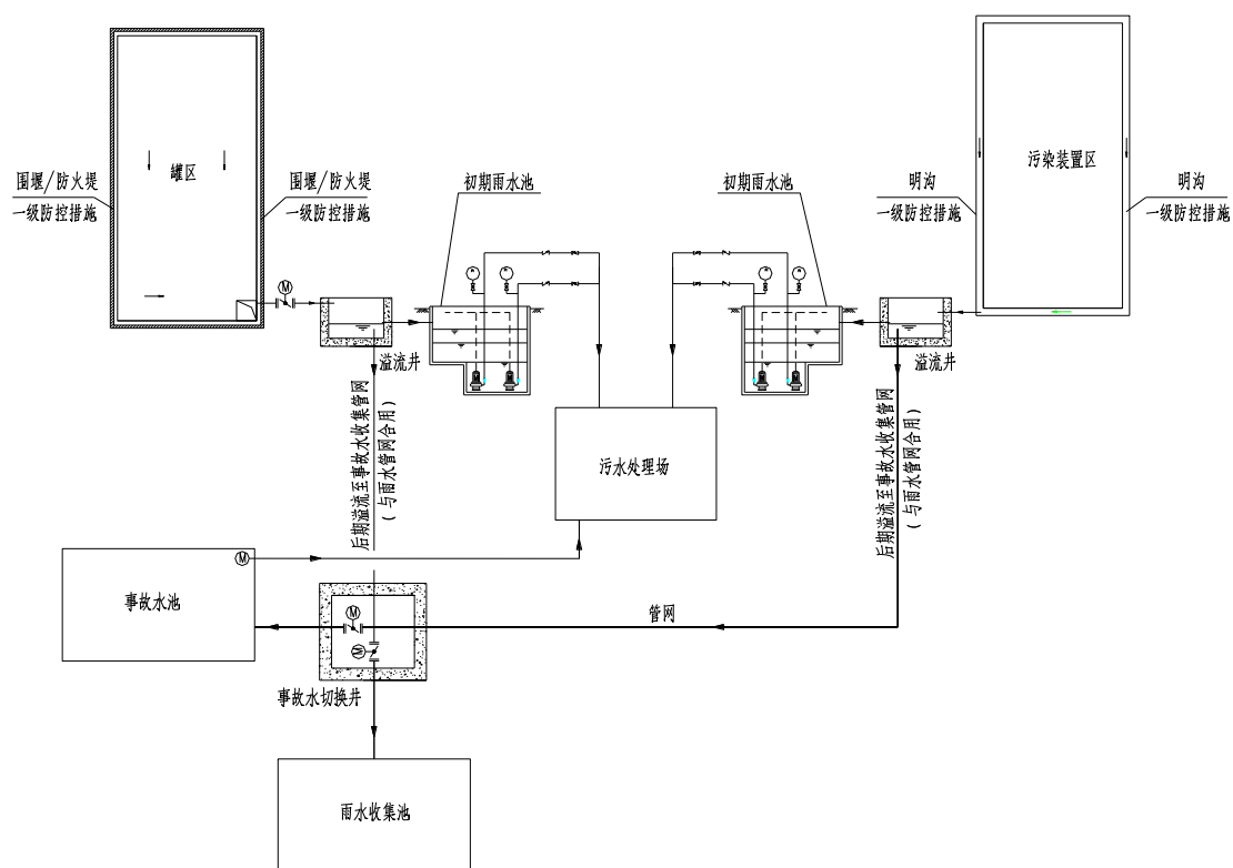
图 8.7-1 消防事故废水三级防控措施典型图
