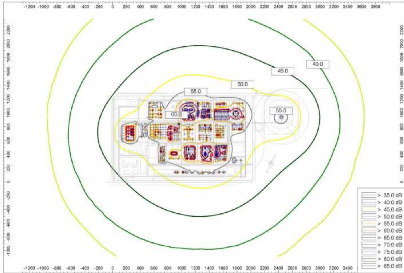
图 7.2-2 拟建工程非正常工况噪声分布图
