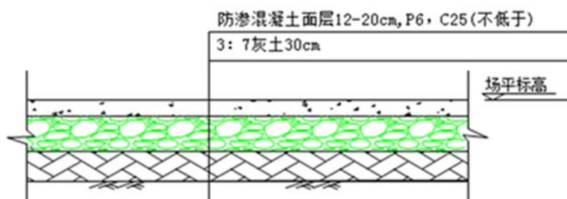
图 9.3-2 一般污染防治区典型防渗结构典型图
