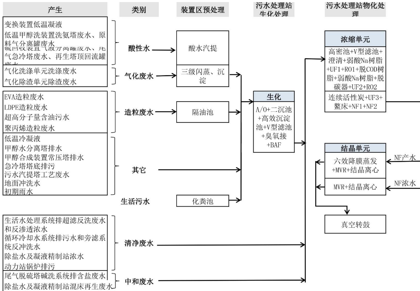
图 9.2-1 污水处理系统流程图
