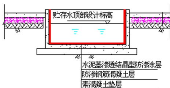
图 9.3-7 污水池、污水井防渗层结构图
