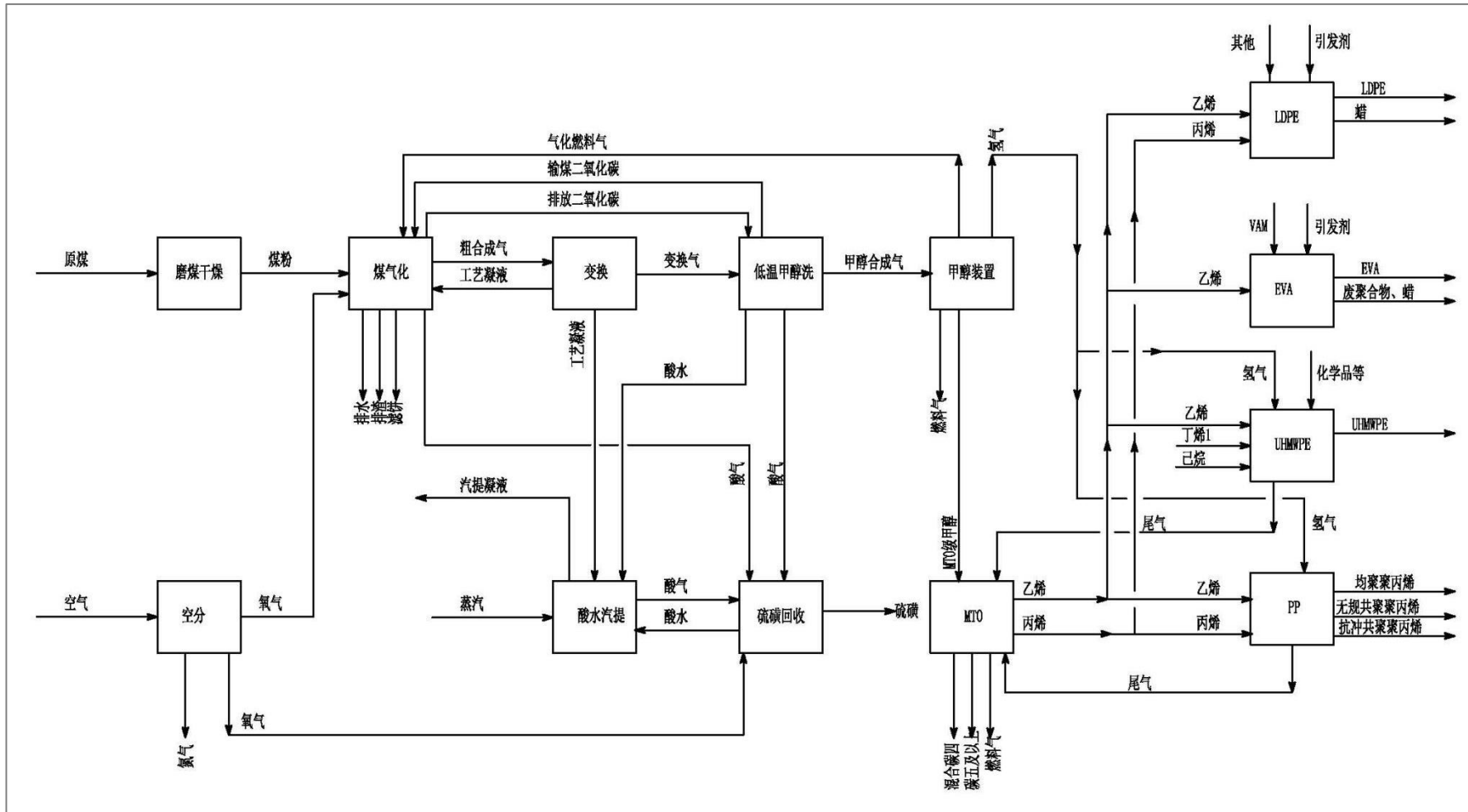
图 3.1-2 全厂工艺流程图
