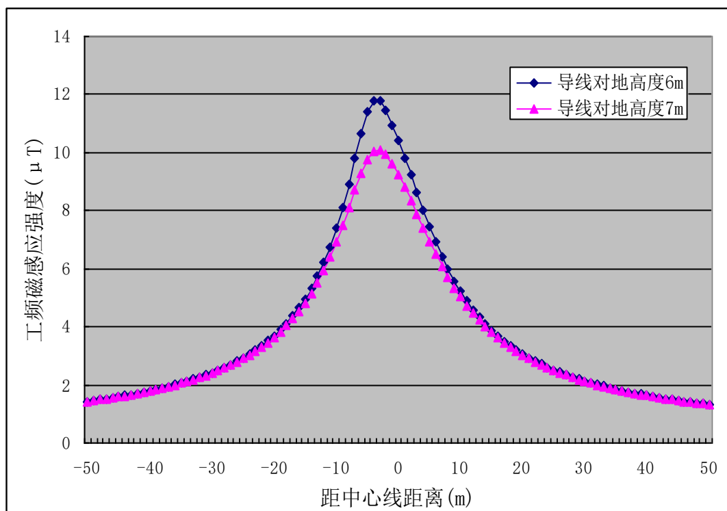
图 7.8-3 110kV 输电线路单回段工频磁感应强度走势图
