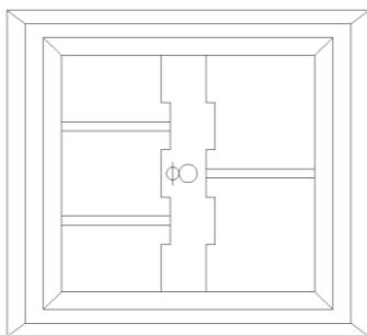
图 9.1-3 水平浓淡快速着火煤粉喷嘴
