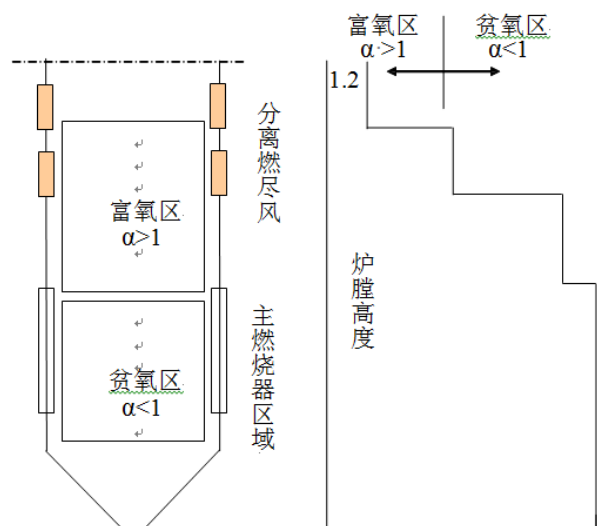
图 9.1-1 沿高度方向过量空气系数的典型分布图
