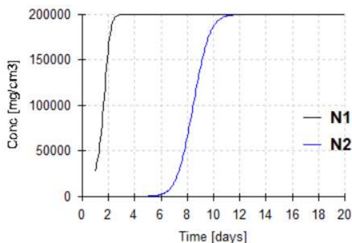
图 7.5-1 不同预测期内氨氮浓度变化曲线（N1-黄土状粉土层下边界，N2-模型下边界）
