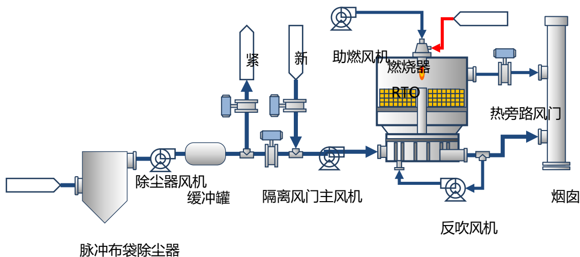
图 9.1-4 RTO 工艺流程图
