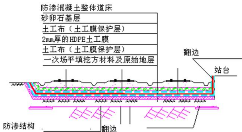
图 9.3-6 铁路、汽车液体产品装卸区路基防渗层结构典型图
