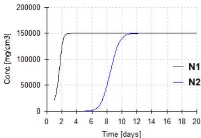
图 7.5-5 不同预测期内石油类浓度变化曲线（N1-黄土状粉土层下边界，N2-模型下边界）
