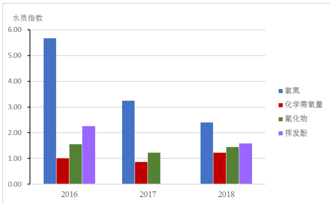
图 4.4-10 大河子沟入东沟断面污染因子水质指数变化图
