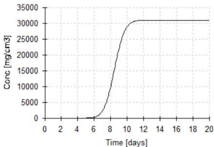
图 7.5-7 不同预测期内氨氮浓度变化曲线（N1-黄土状粉土层下边界，N2-模型下边界）
