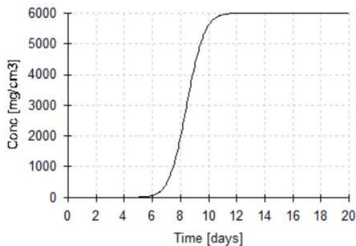
图 7.5-3 不同预测期内氰化物浓度变化曲线（N1-黄土状粉土层下边界，N2-模型下边界）
