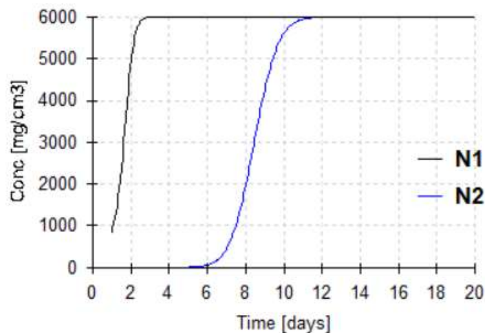
图 7.5-3 不同预测期内氰化物浓度变化曲线（N1-黄土状粉土层下边界，N2-模型下边界）
