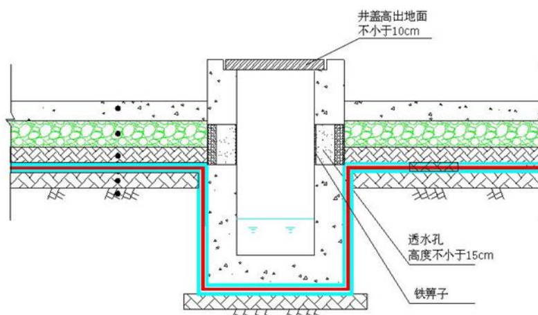
图 9.3-8 渗漏液收集井典型结构
