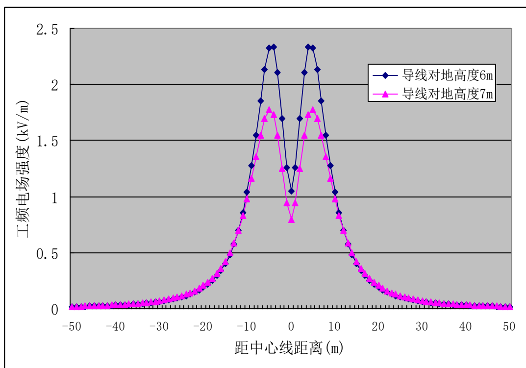
图 7.8-2 110kV 输电线路单回路工频电场强度走势图
