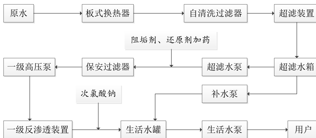
图 3.4-1 生活水处理系统工艺流程方框图
