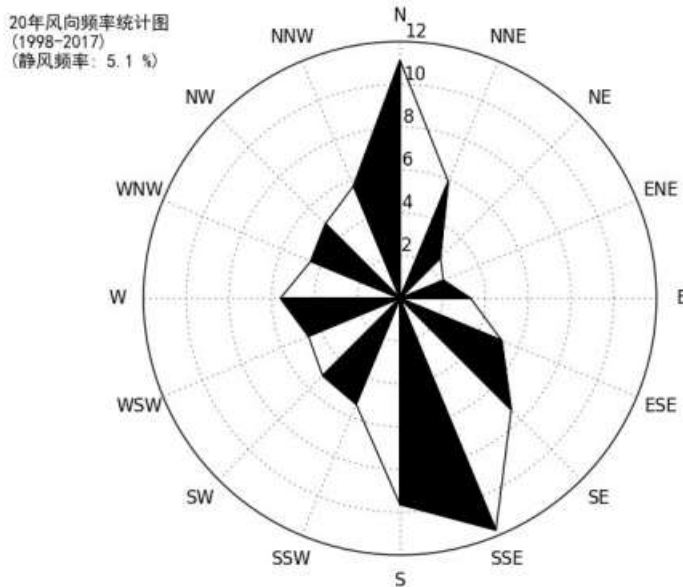
图 7.1-1 灵武站多年风向玫瑰图
