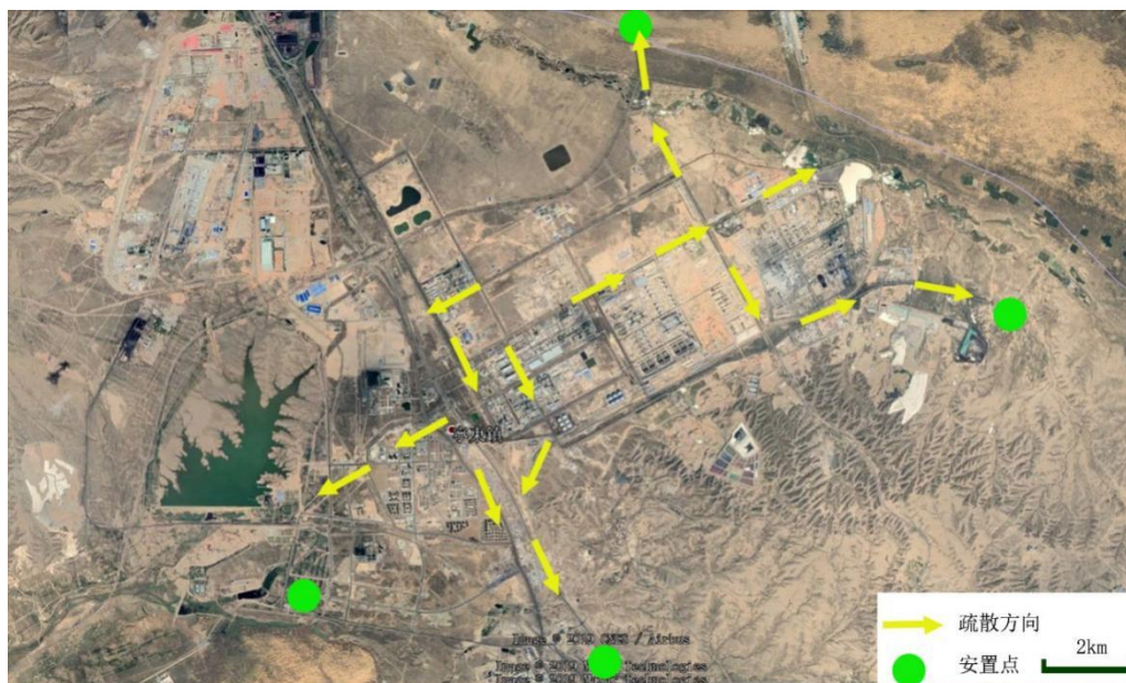
图 8.7-7 应急疏散路线示意图
