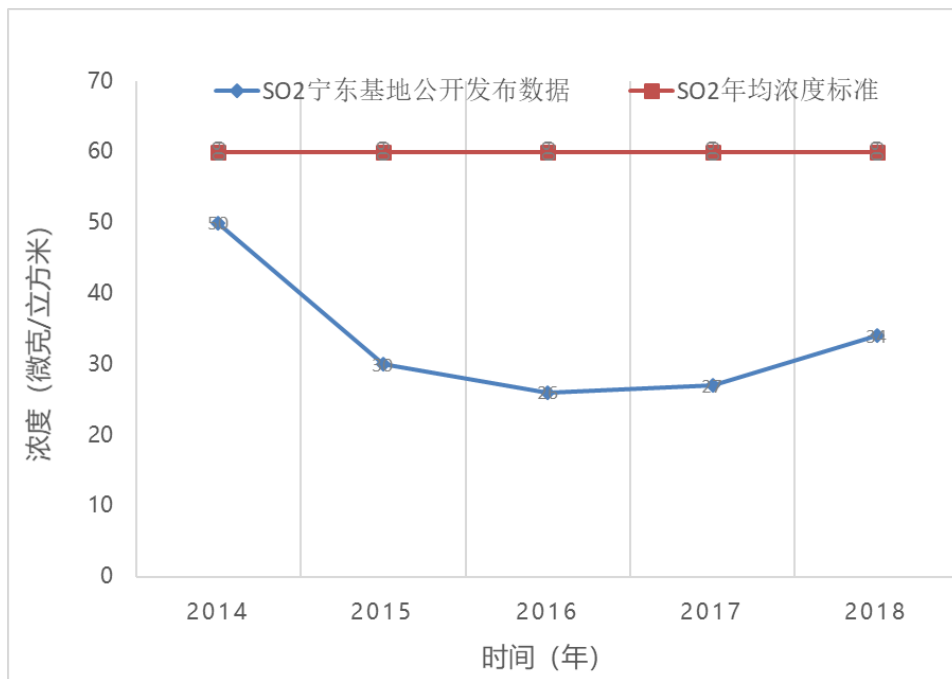
图 4.4-4 区域 SO 2 变化趋势图
