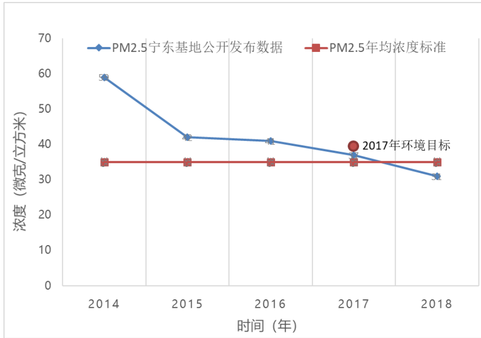
图 4.4-3 区域 PM 2.5 变化趋势图
