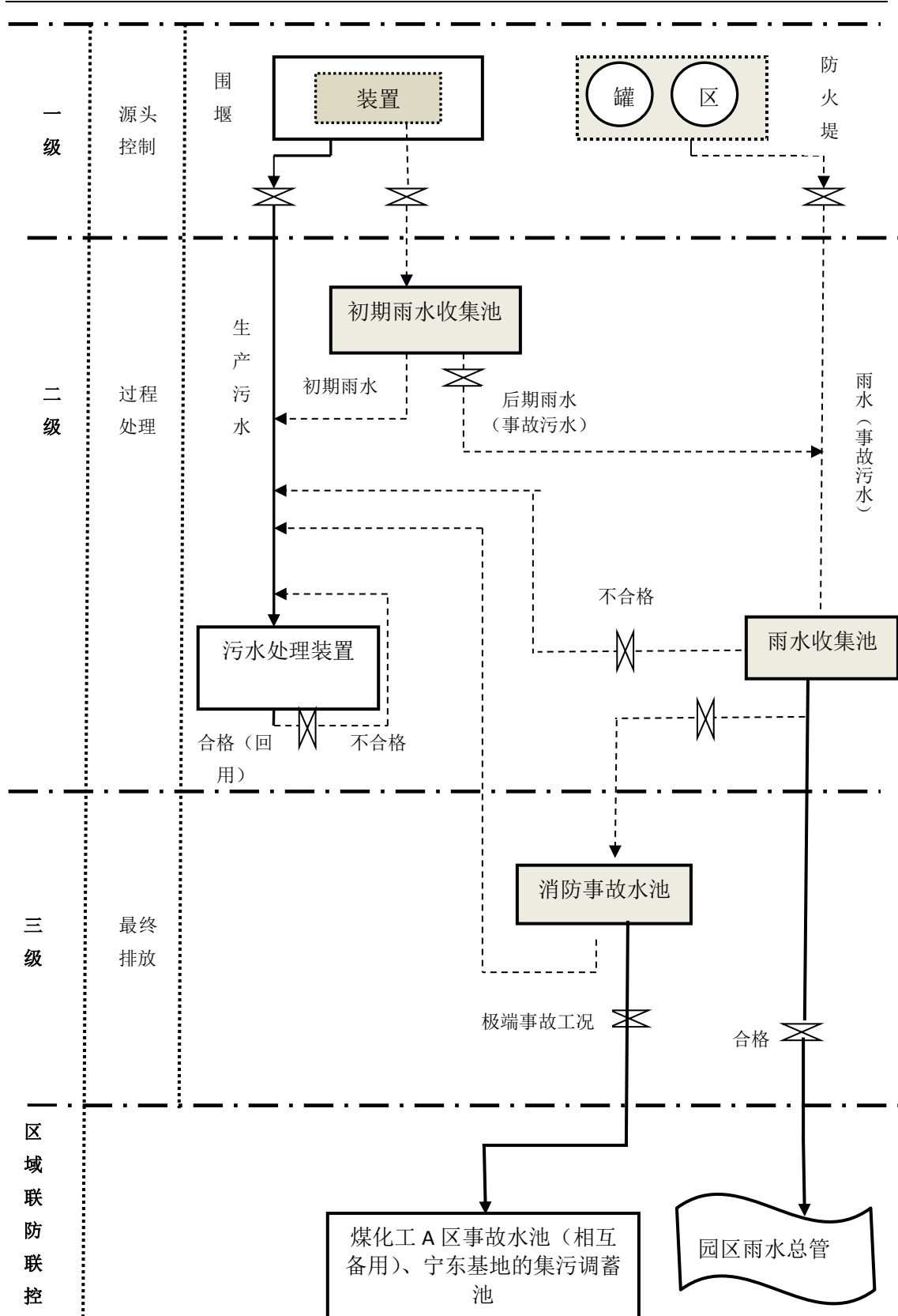
图 8.7-3 事故废水三级防控系统示意图
