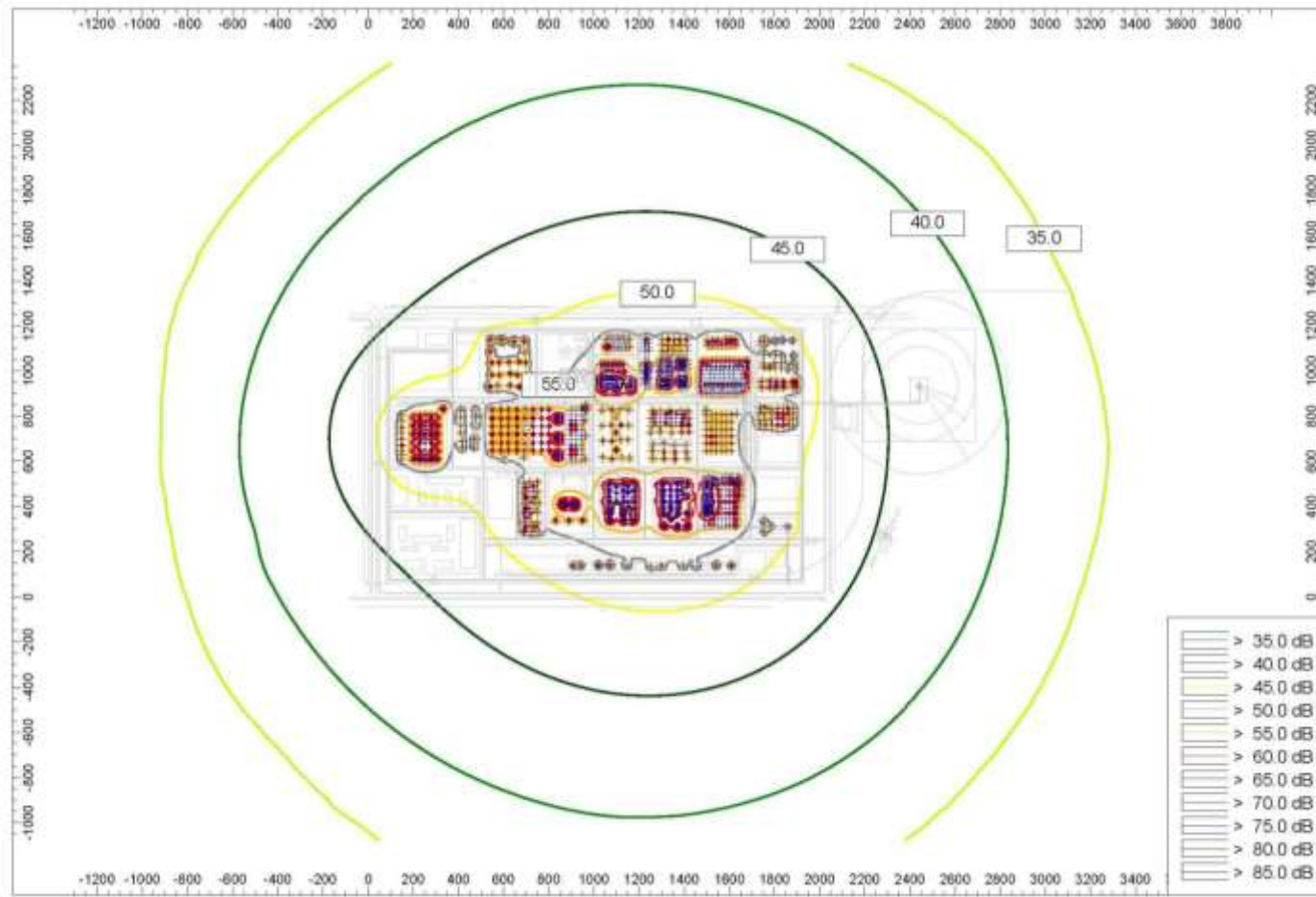
图 7.2-1 拟建工程正常工况噪声贡献值分布图
