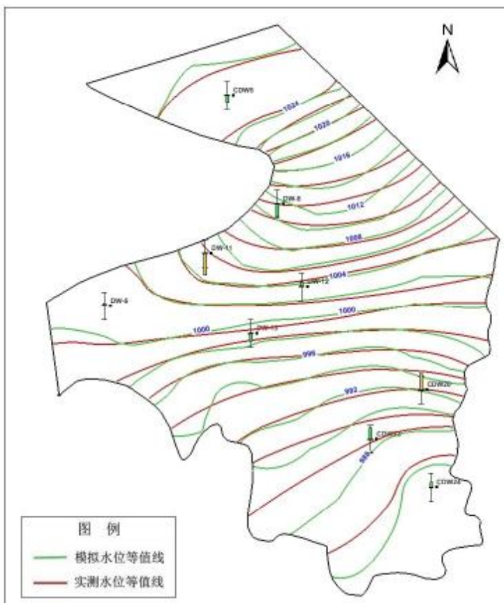
图 6.4-32 承压水流场拟合图
