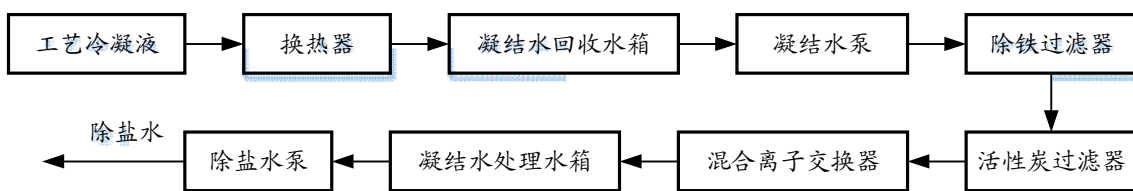
图 4.4-3 工艺凝结水制除盐水流程图
