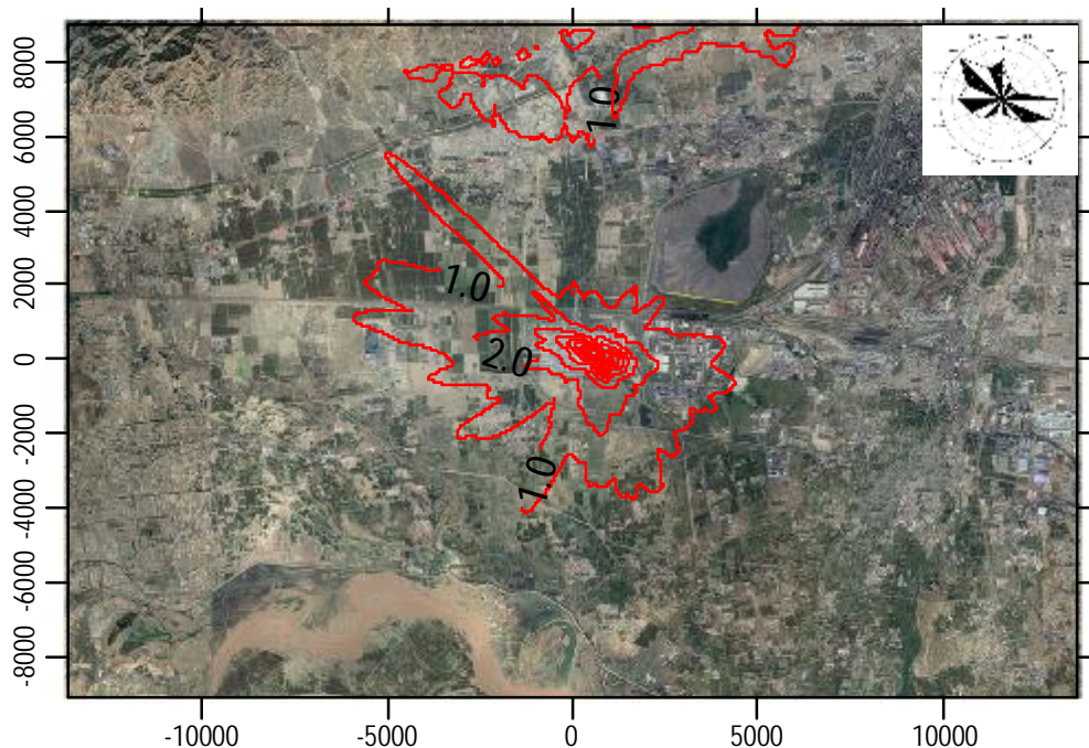
图 6.2-15 \text{PM}_{10} 最大日均浓度等值线分布图 (单位: \mu\text{g}/\text{m}^3 )
