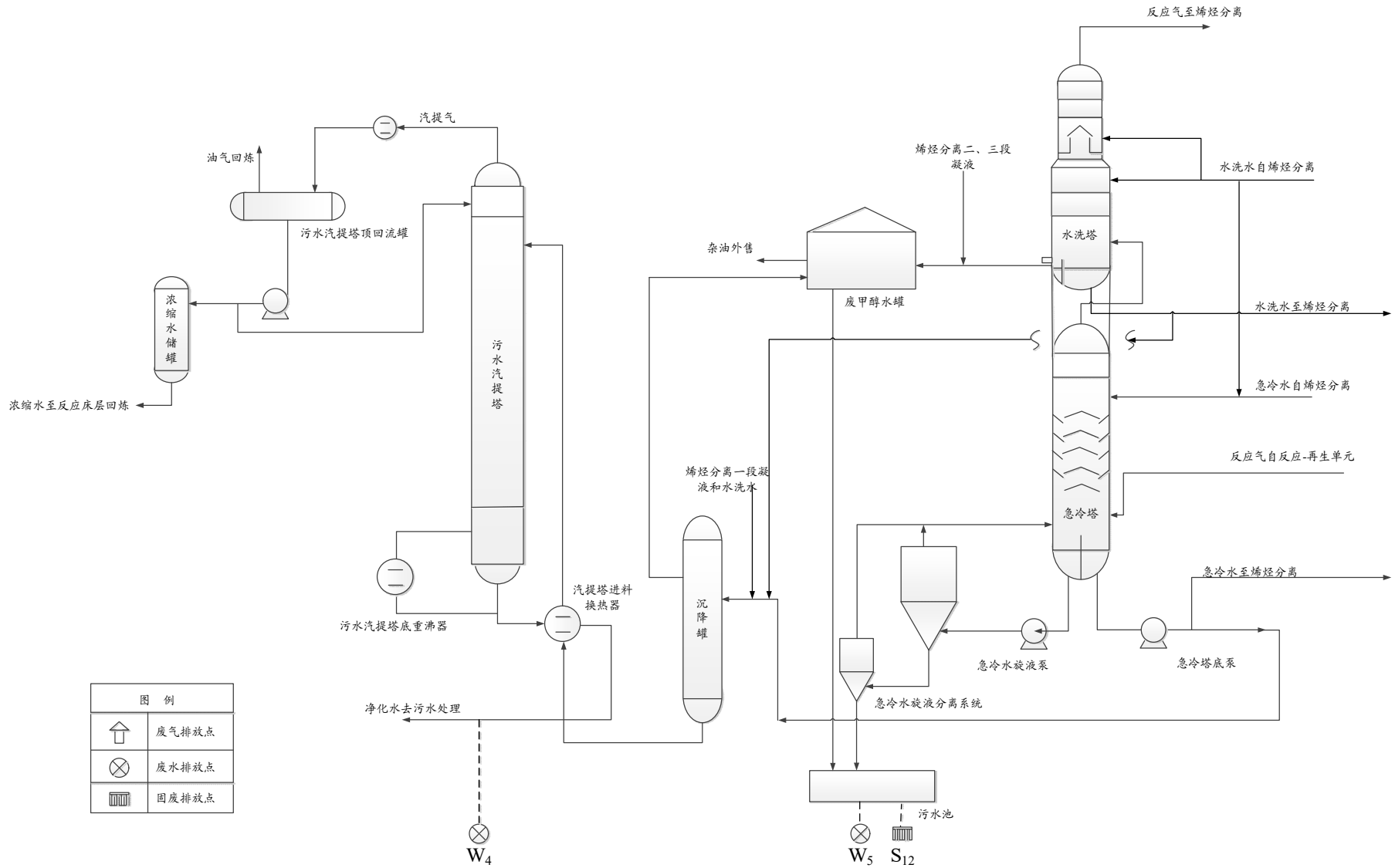
图 3.2-9 MTO 装置产排污节点图 (c)
