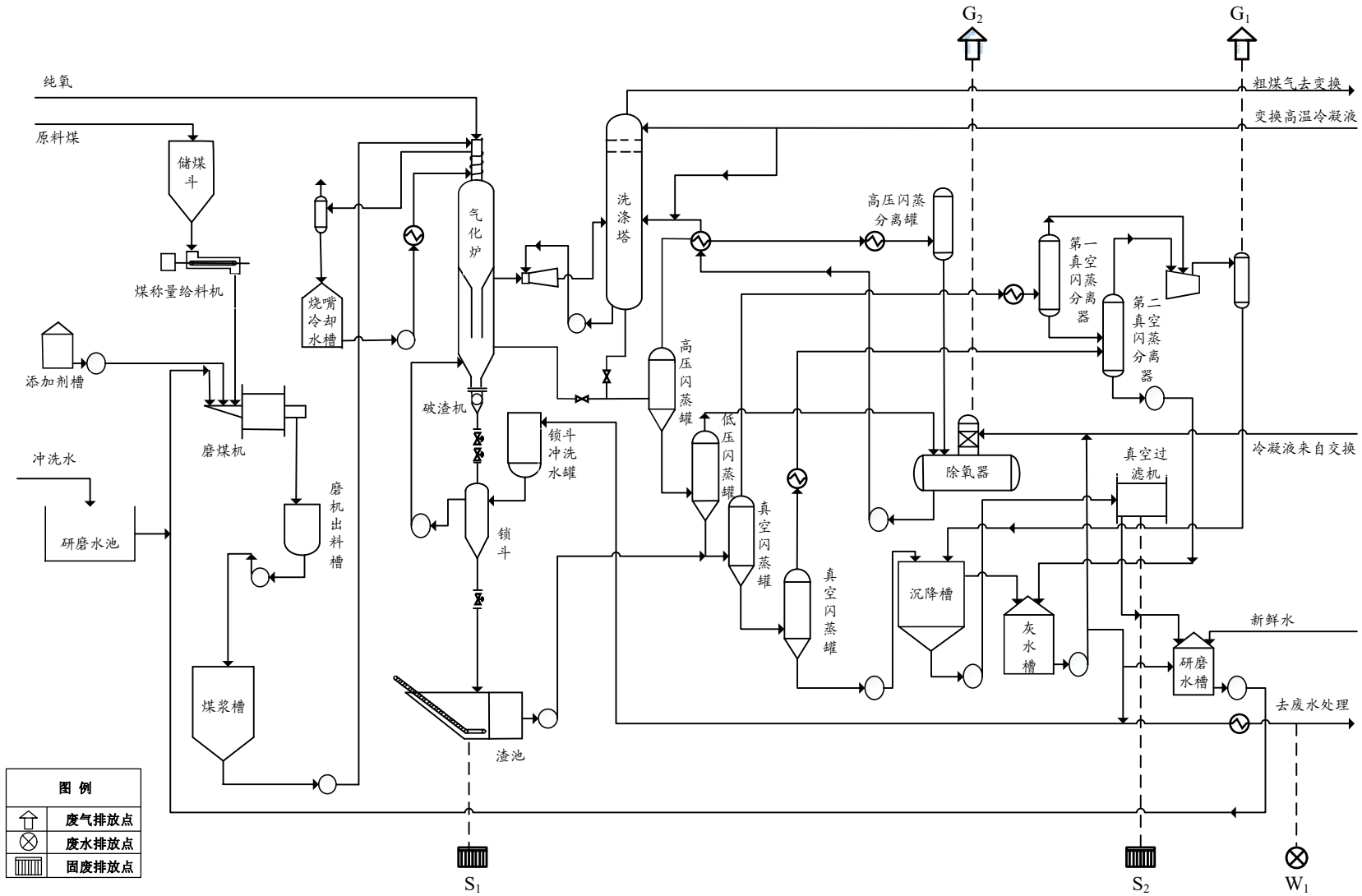
图 3.2-2 气化装置产排污节点图
