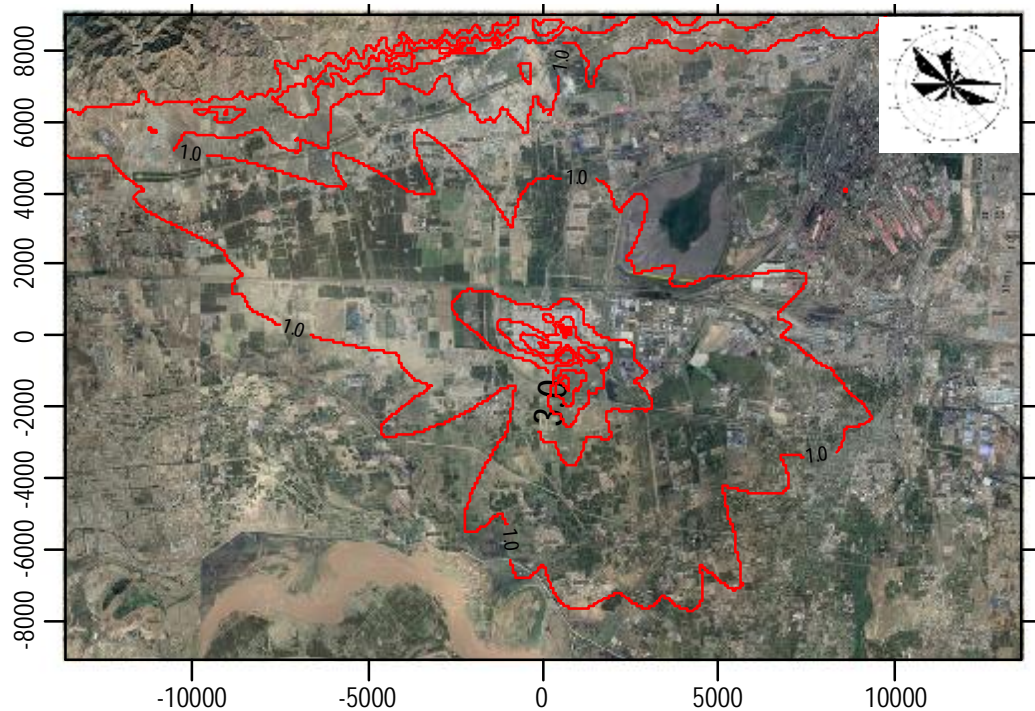
图 6.2-11 NO 2 最大日均浓度等值线分布图 (单位: \mu\text{g}/\text{m}^3 )
