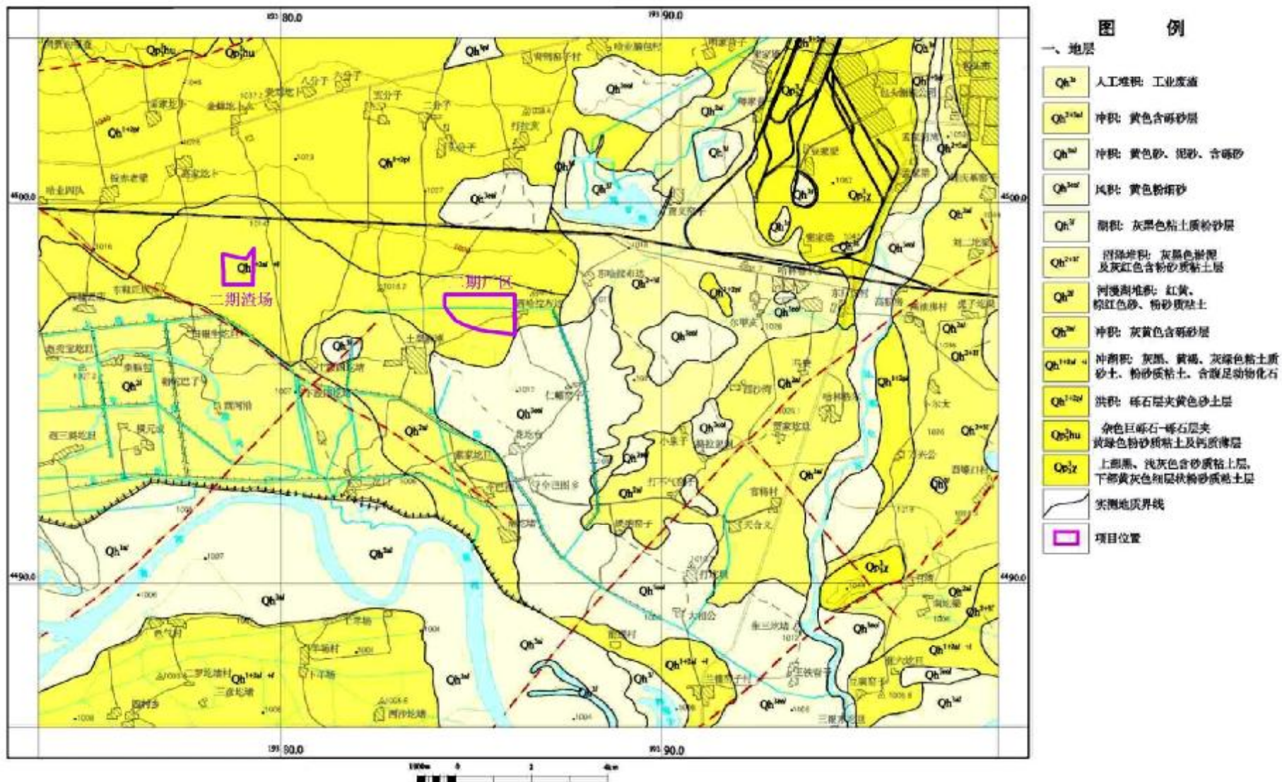
图 5.1-2 区域地质图
