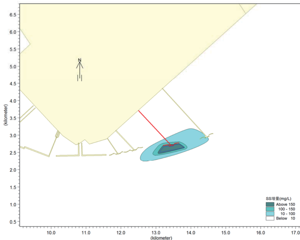
图 5.3-3 疏浚施工悬浮物影响范围包络线
