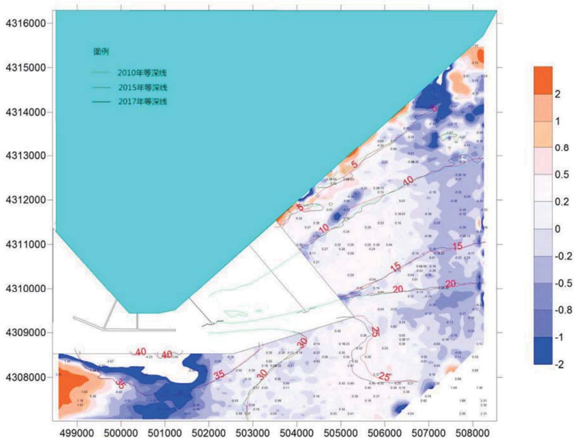
图 4.3-2 曹妃甸海域地形冲淤变化 (2010.9~2017.8)
