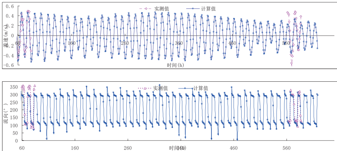
图 5.1-5 V1 站流速、流向验证
