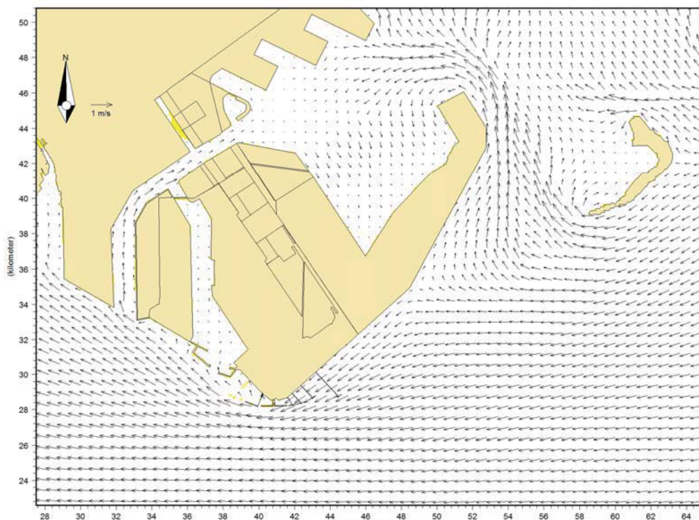
图 5.1-15 现状涨急局部流场（小潮）
