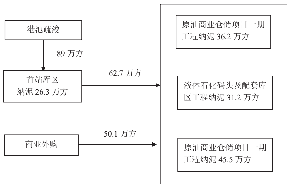
图 3.9-4 项目土方平衡图
