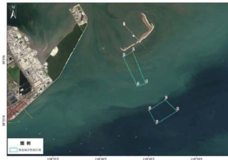
图 5.8-1 模型模拟区范围边界图
