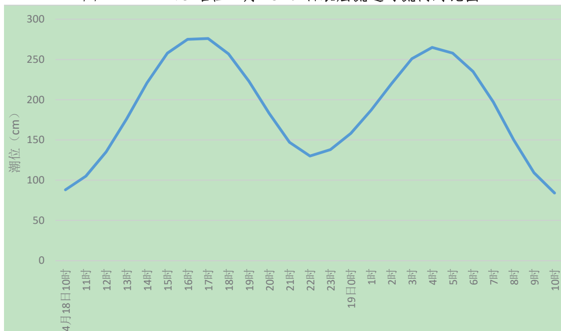
图 4.2-3 曹妃甸海洋站 4 月 18-19 日潮位变化曲线
