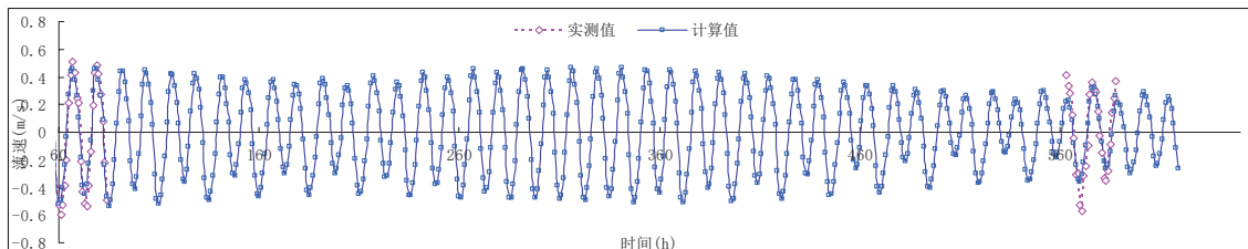
图 5.1-5 V1 站流速、流向验证
