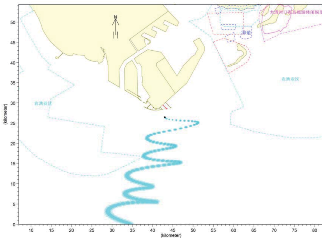
图 7.5-8 港池和航道交汇处冬季风工况下落潮溢油事故发生 72 小时影响范围
