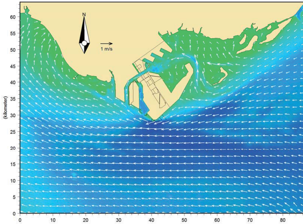
图 5.1-11 现状涨急流场（大范围）
