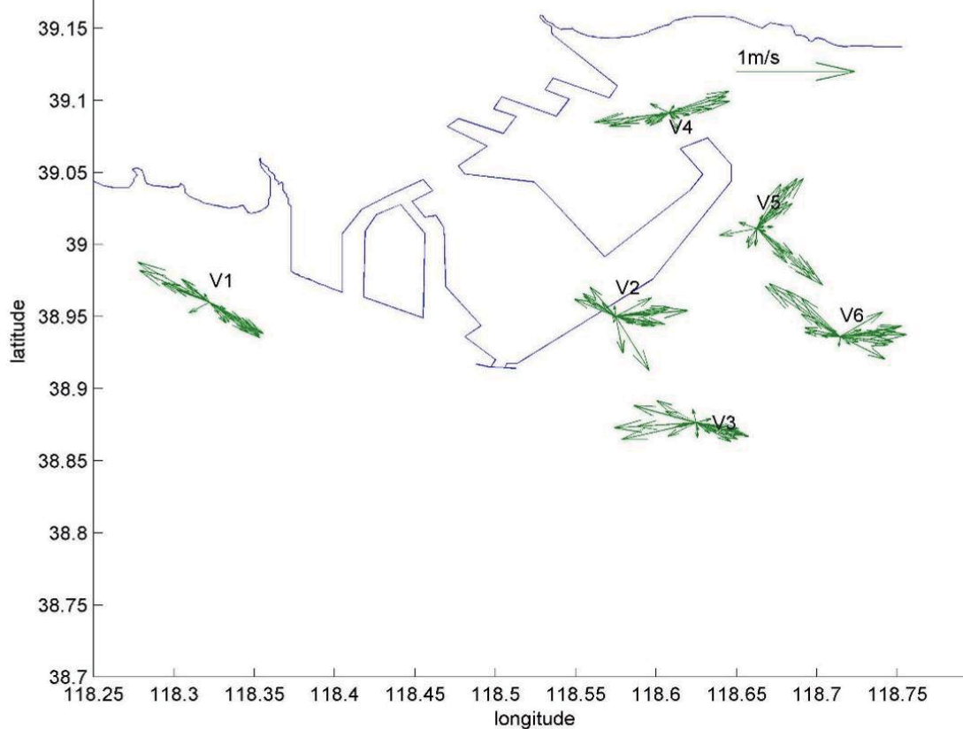
图 4.2-8 小潮期（5月 9-10 日）观测站位表层海流矢量图
