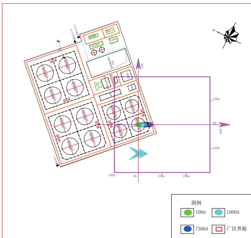
图 6.3-5 油储罐爆炸石油类影响范围预测图
