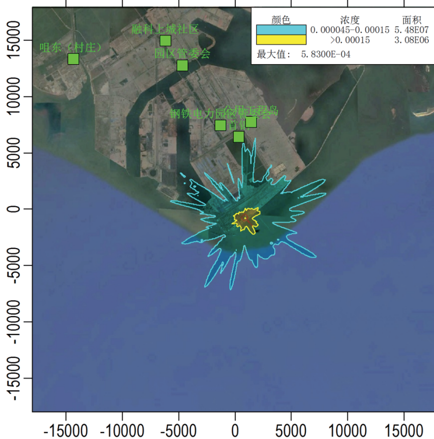
图 6.1-6 SO 2 新增污染源最大日平均质量浓度分布图
