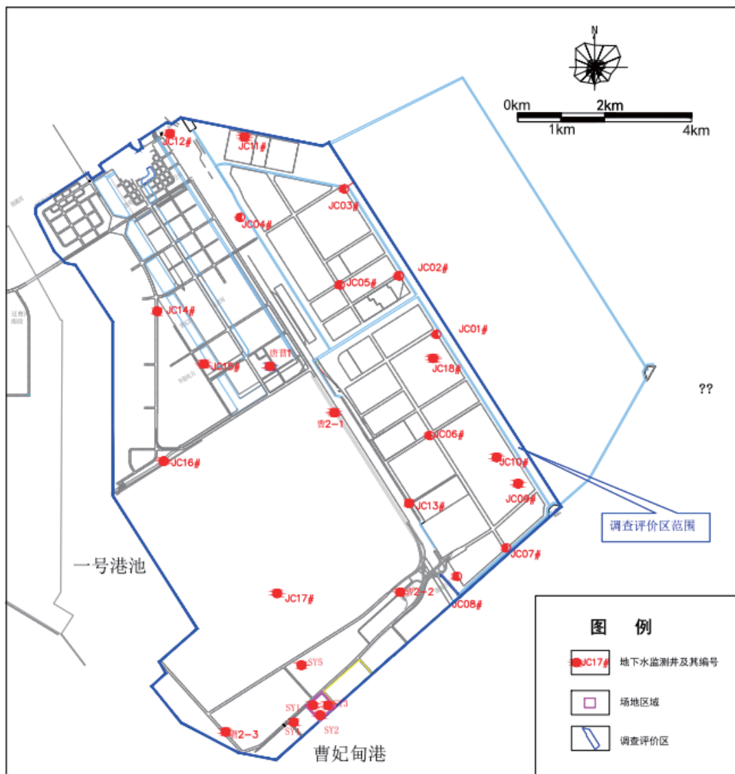
图 4.11-10 调查评价区内地下水监测点布置图
