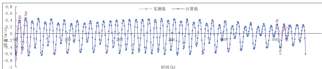
图 5.1-7 V3 站流速、流向验证
