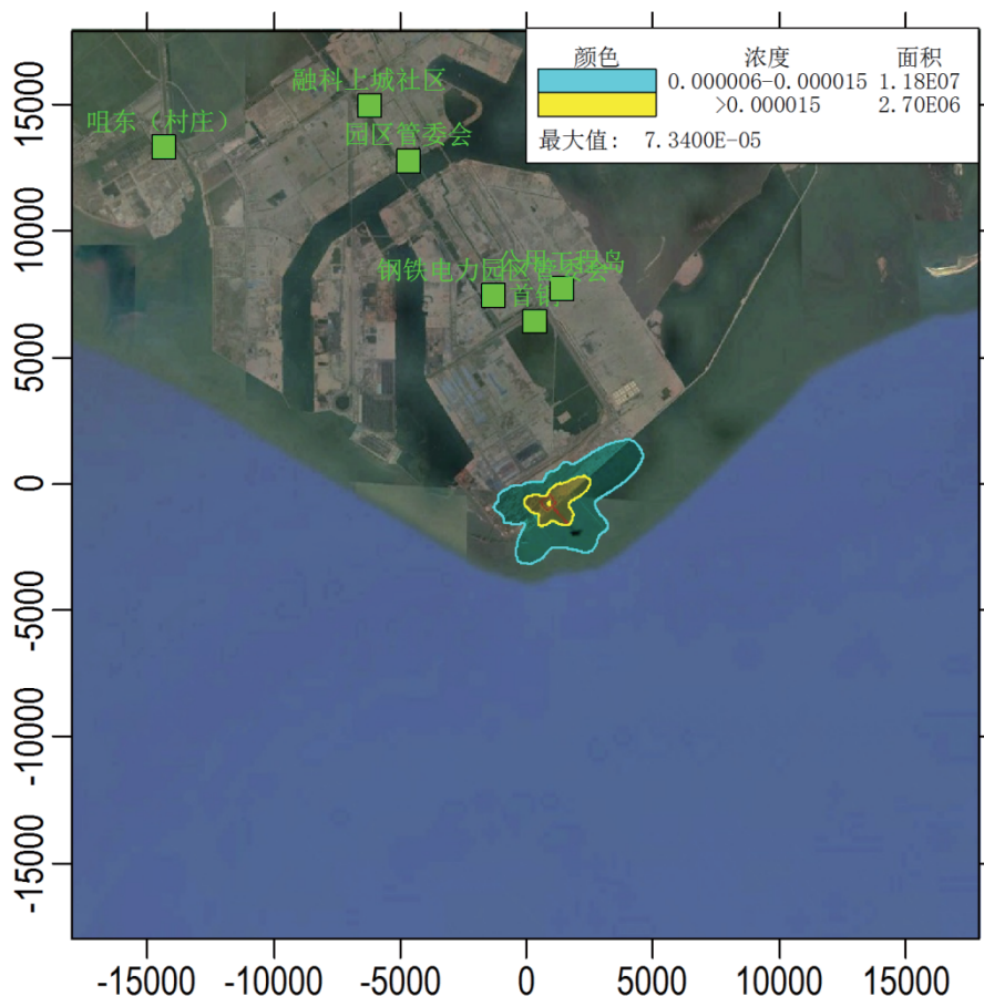
图 6.1-7 SO 2 新增污染源年均质量浓度分布图
