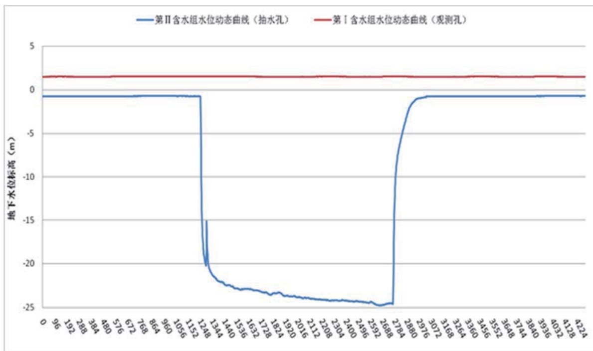
图 4.11-1 调查评价区内第 II 含水组抽水试验地下水水位动态历时曲线
