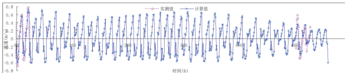
图 5.1-8 V4 站流速、流向验证
