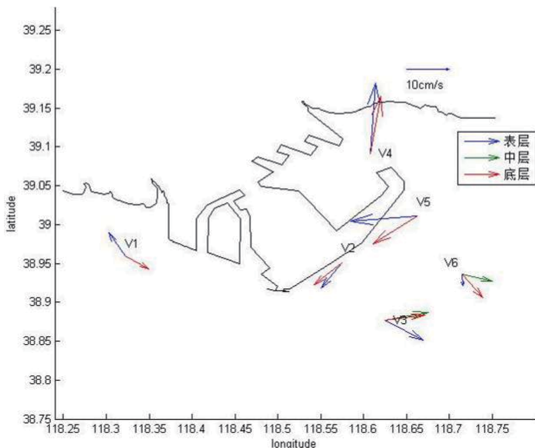
图 4.2-11 曹妃甸附近海域观测站位小潮各层余流矢量图
