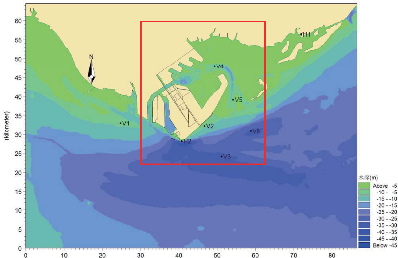
图 5.1-2 模型计算区域、嵌套范围以及水文站位示意图
