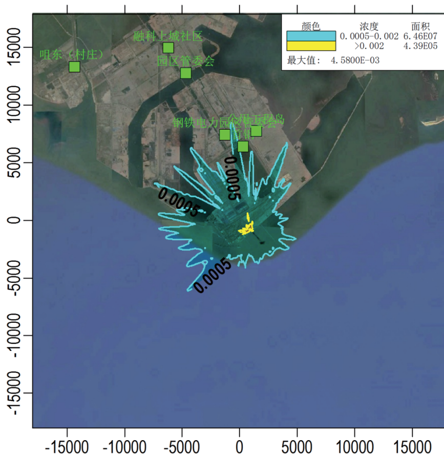
图 6.1-5 SO 2 新增污染源最大小时质量浓度分布图
