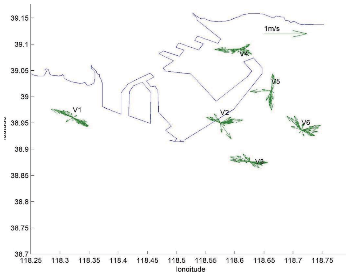
图 4.2-9 小潮期 (5 月 9-10 日) 观测站位底层海流矢量图
