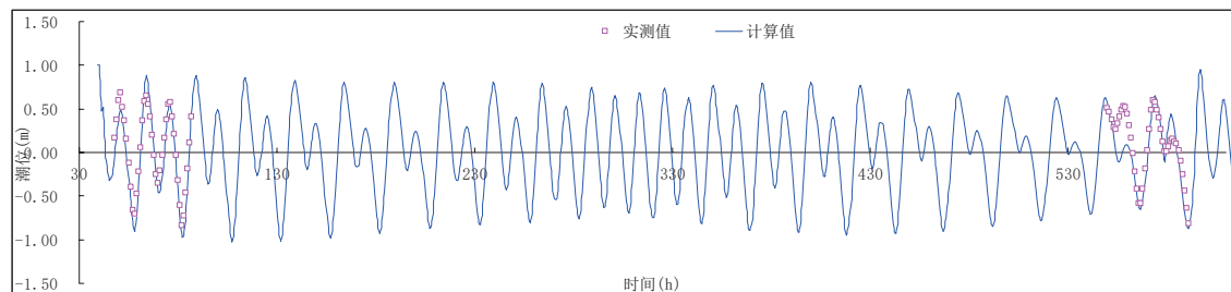
图 5.1-3 三岛 H1 潮位验证过程线
