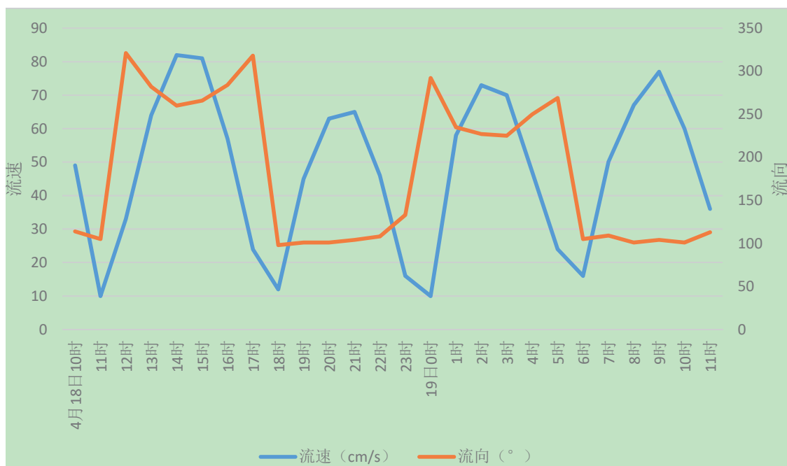
图 4.2-2 V3 站位 4 月 18-19 日表层流速与流向对比图
