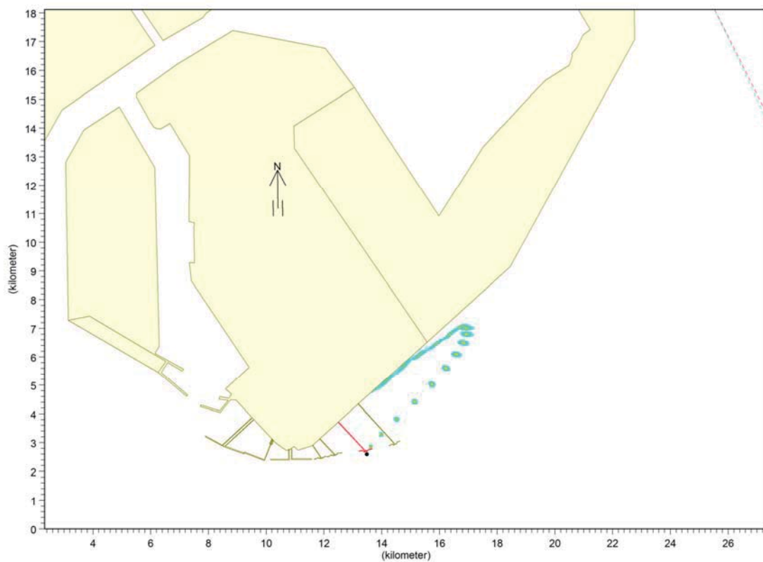
图 7.5-2 码头前沿处落潮期夏季风风况下溢油事故发生 72 小时影响范围
