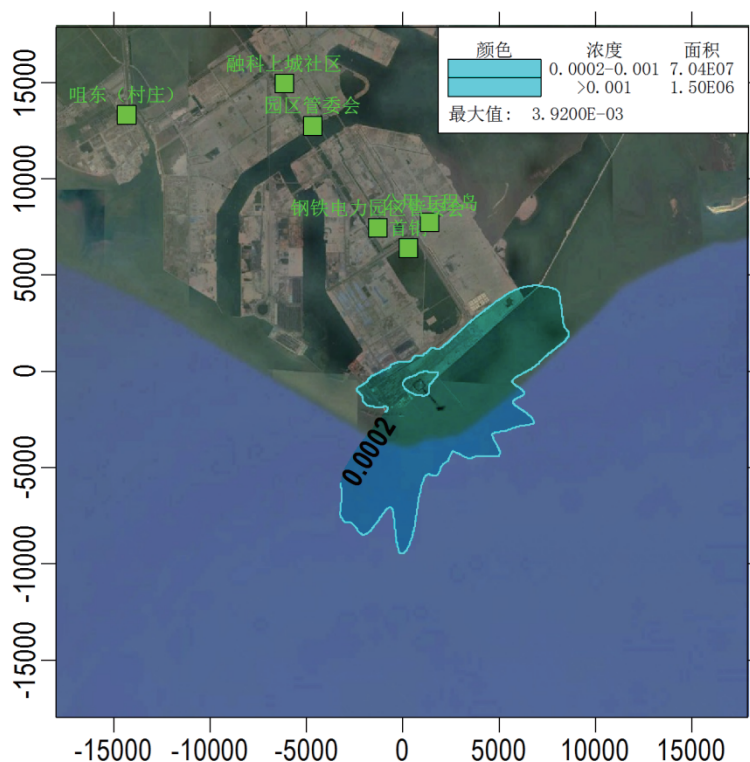
图 6.1-13 NMHC 新增污染源年均质量浓度分布图
