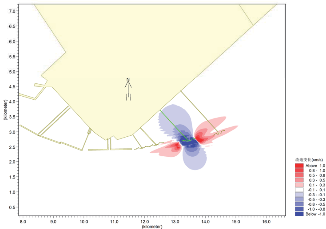
图 5.1-21 工程前后平均流速大小变化图
