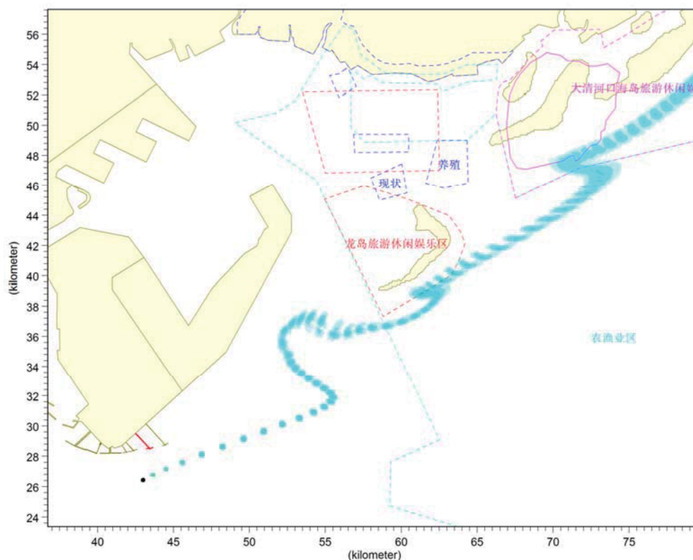
图 7.5-11 港池和航道交汇处 SSW 风不利风况下落潮期溢油事故发生 72 小时影响范围
