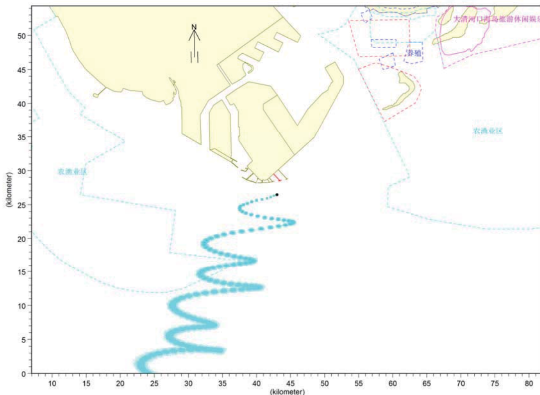
图 7.5-7 港池和航道交汇处冬季风工况下涨潮溢油事故发生 72 小时影响范围
