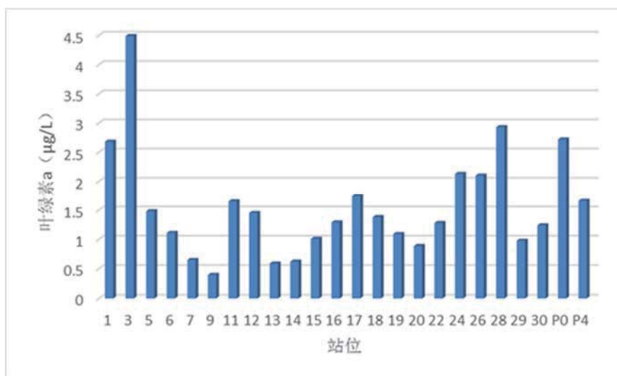
图 4.7-10 调查海区叶绿素 a 含量 ( \text{mg/m}^3 )
