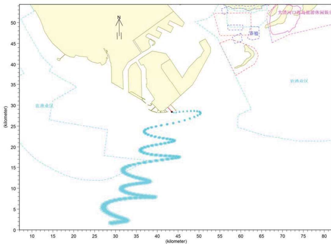
图 7.5-4 码头前沿处冬季风工况下落潮溢油事故发生 72 小时影响范围
