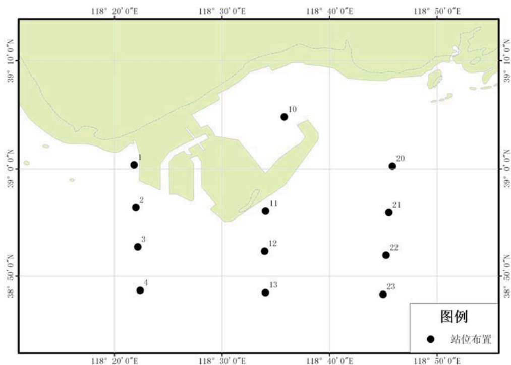
图 4.8-1 渔业资源调查站位
