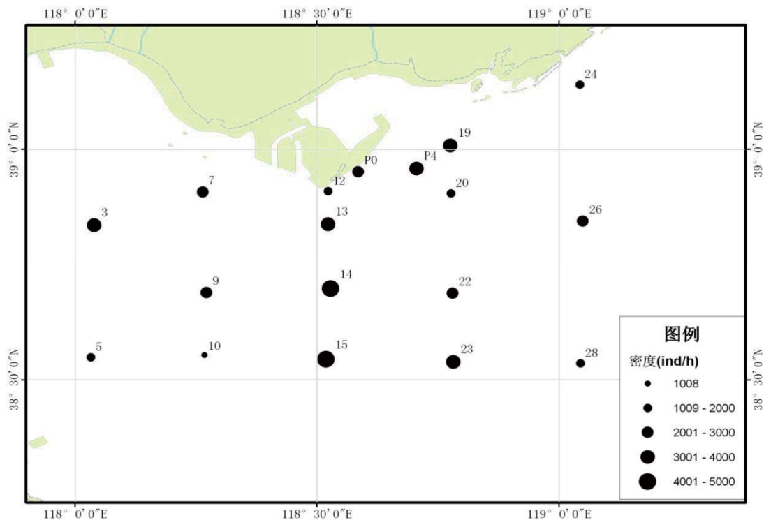
图 4.8-5 生物密度分布
