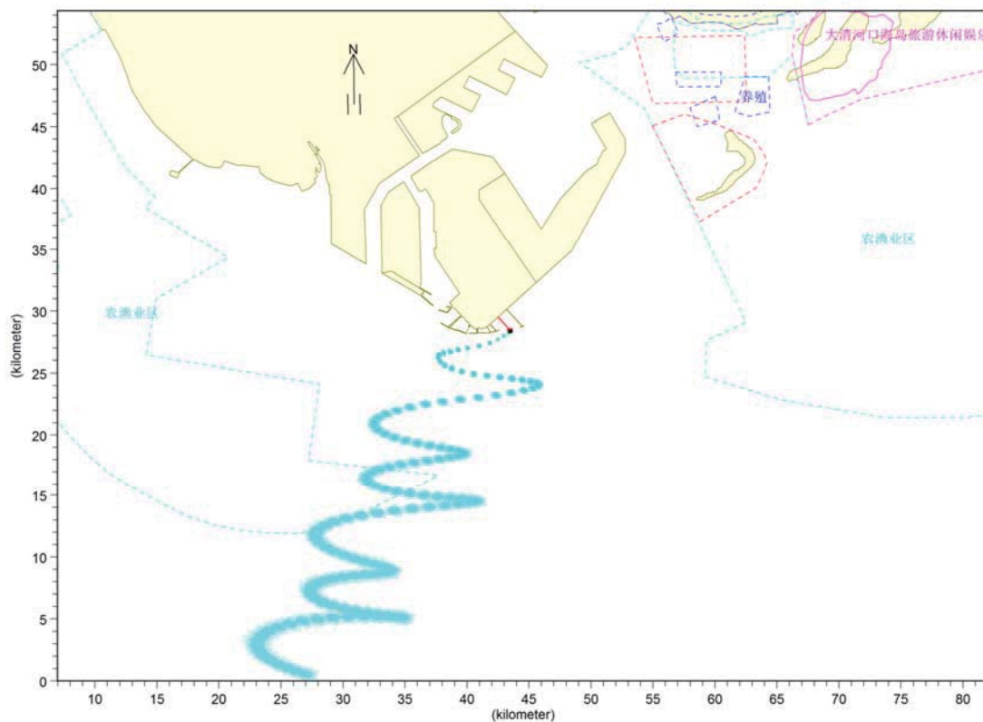
图 7.5-3 码头前沿处冬季风工况下涨潮溢油事故发生 72 小时影响范围
