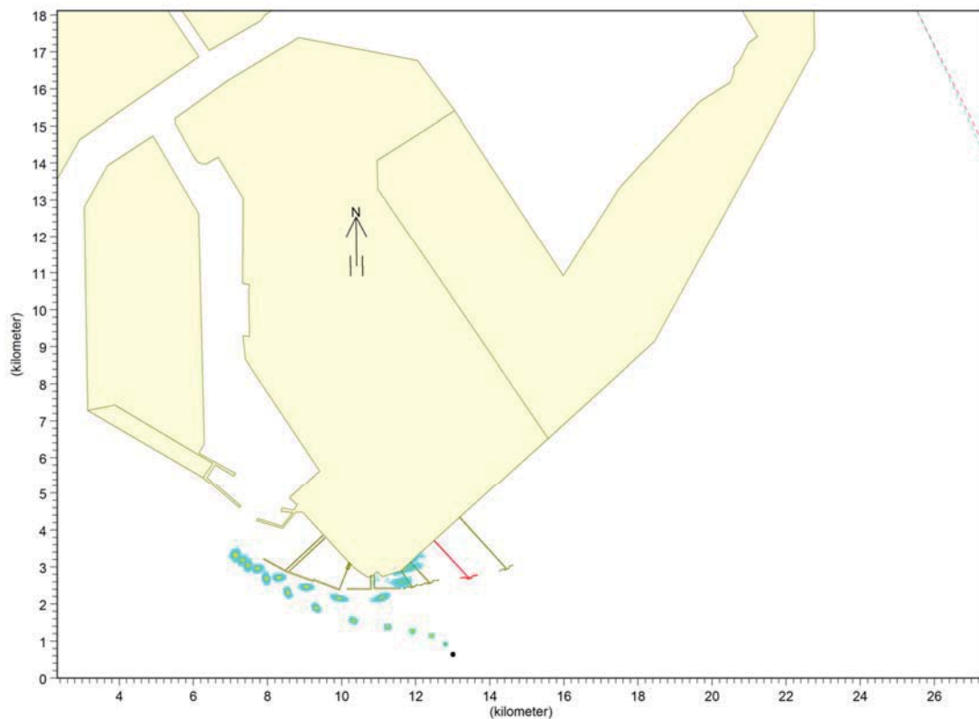
图 7.5-5 港池和航道交汇处涨潮期夏季风风况下溢油事故发生 72 小时影响范围
