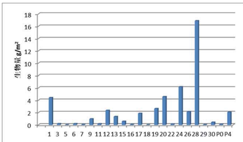
图 4.7-17 调查海域大型底栖生物生物量分布 (g/m 2 )
