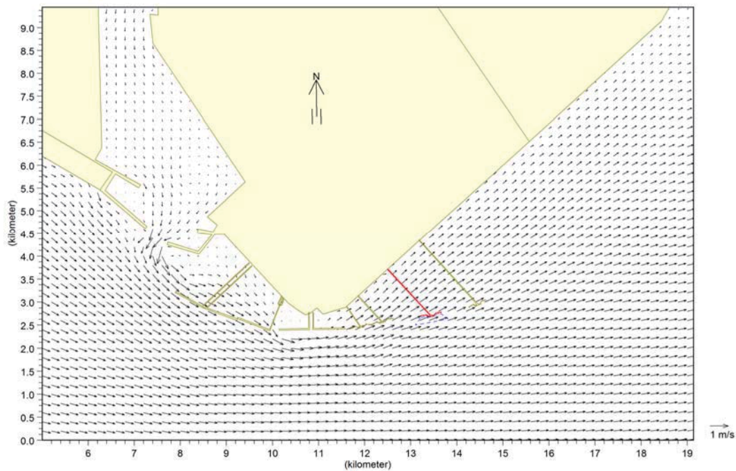
图 5.1-20 工程后落急时刻潮流矢量图
