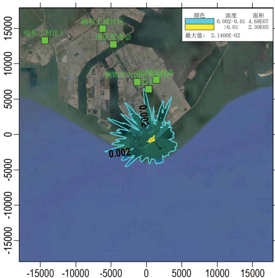
图 6.1-8 NO 2 新增污染源最大小时质量浓度分布图
