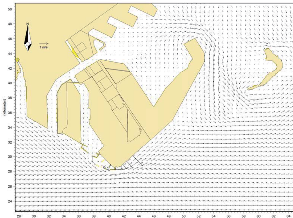
图 5.1-14 现状落急局部流场（大潮）
