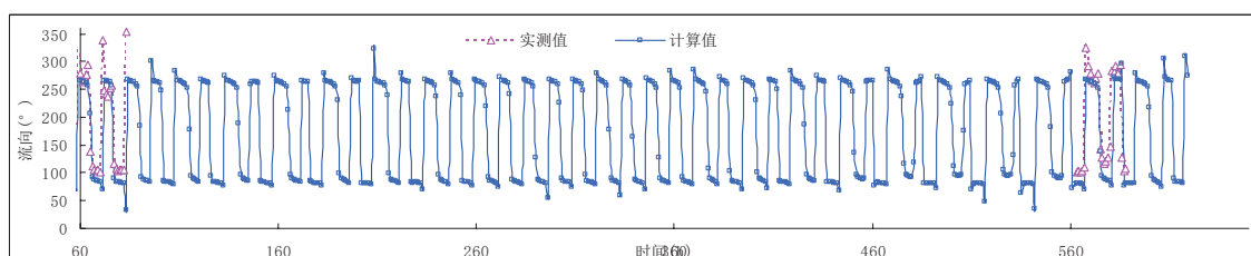
图 5.1-7 V3 站流速、流向验证
