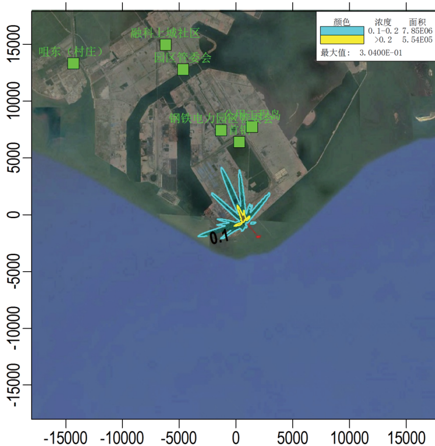
图 6.1-11 NMHC 新增污染源最大小时质量浓度分布图
