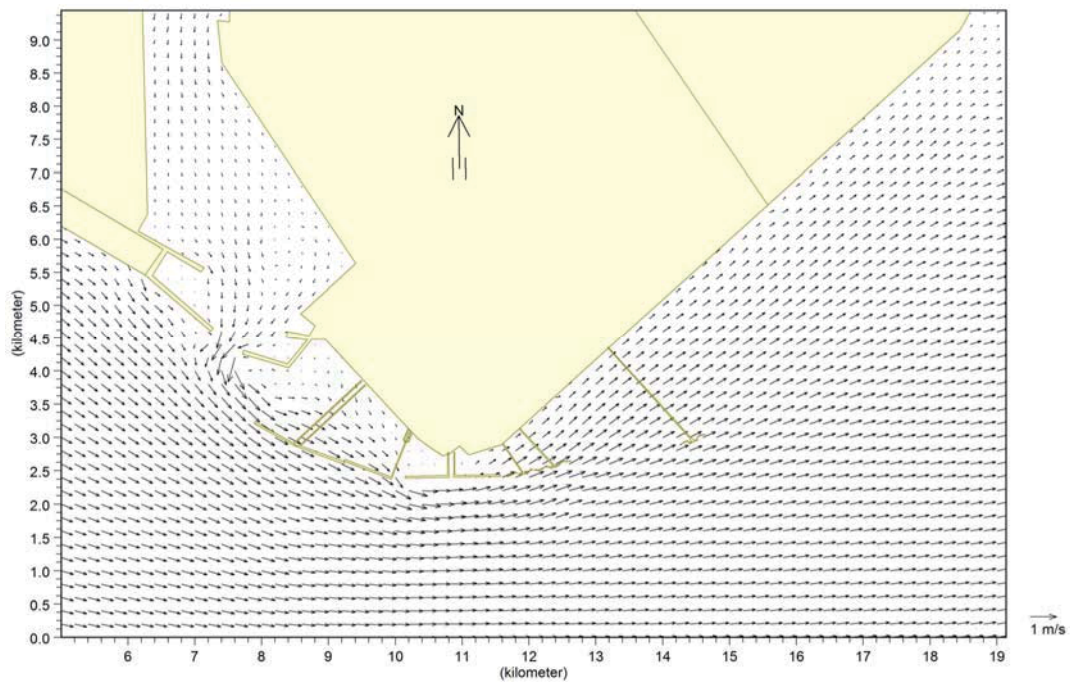
图 5.1-18 工程前落急时刻潮流矢量图
