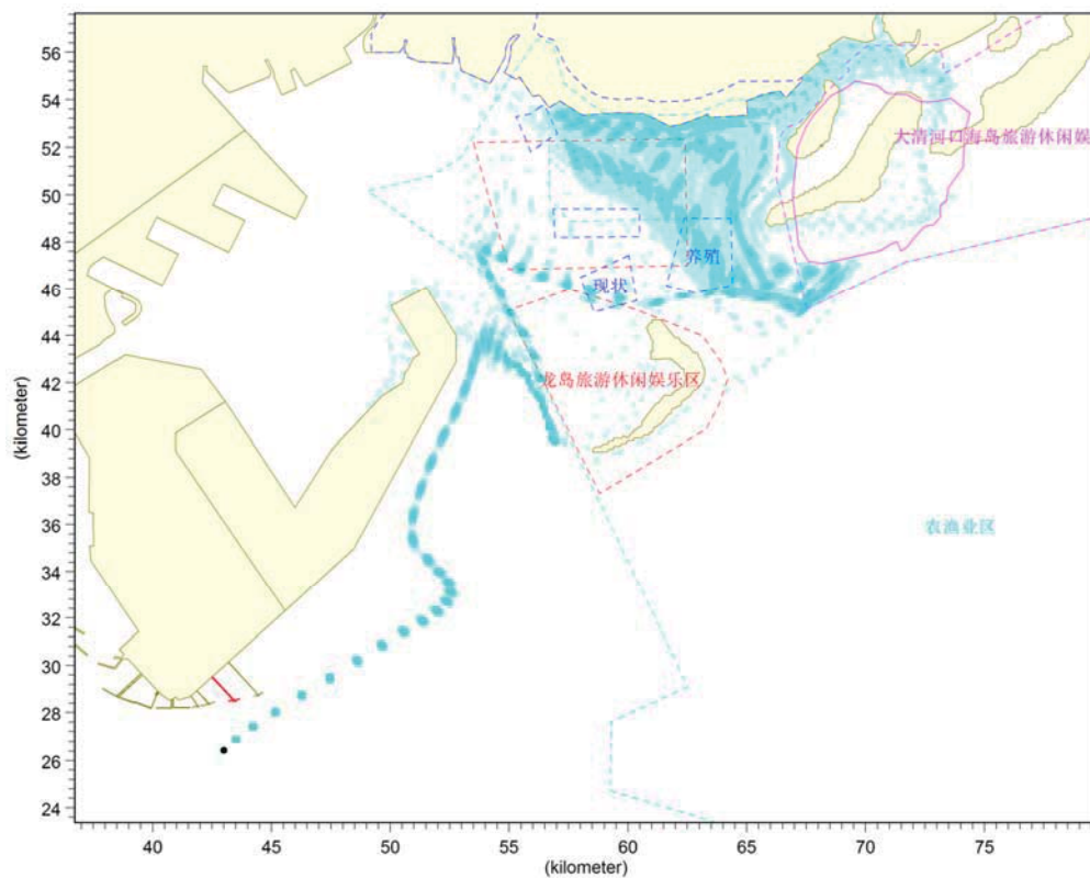
图 7.5-10 港池和航道交汇处 SW 风不利风况下落潮期溢油事故发生 72 小时影响范围
