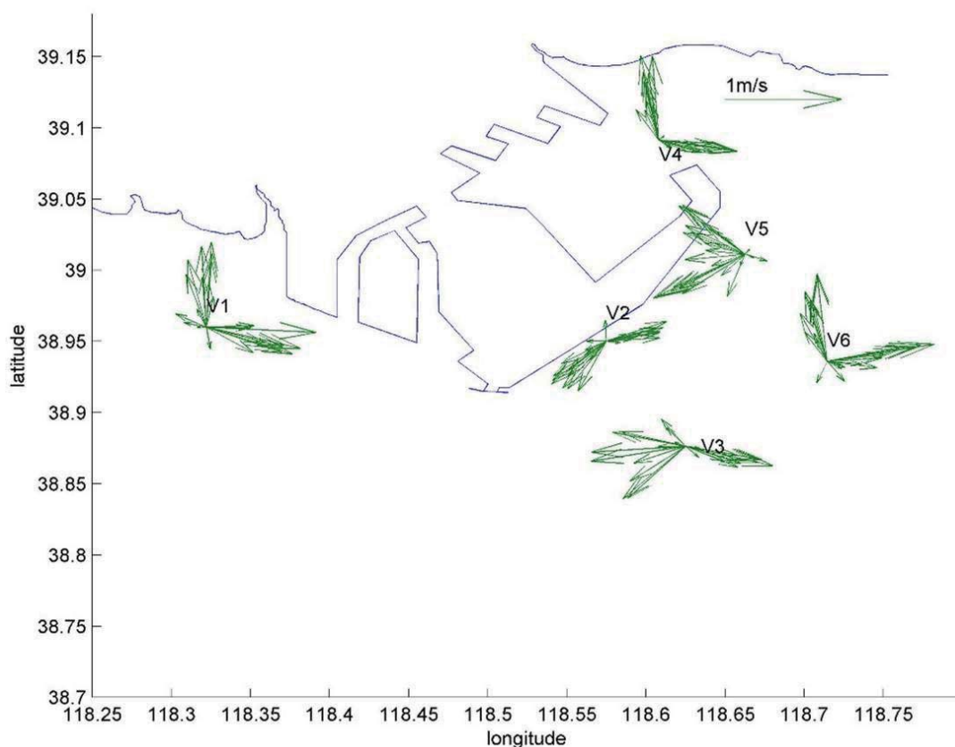
图 4.2-6 大潮期（4月 18-19 日）观测站位表层海流矢量图
