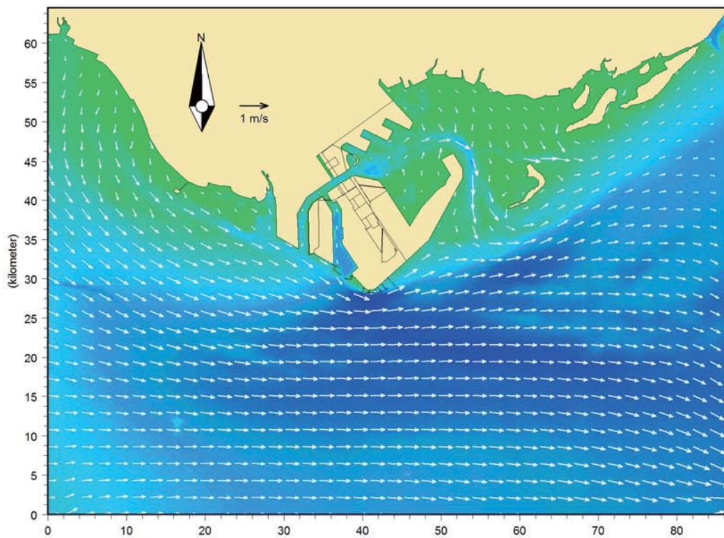
图 5.1-12 现状落急流场（大范围）
