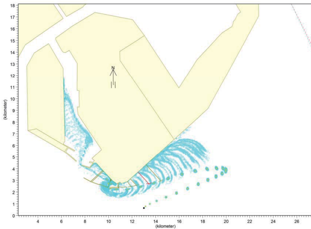
图 7.5-6 港池和航道交汇处落潮期夏季风风况下溢油事故发生 72 小时影响范围
