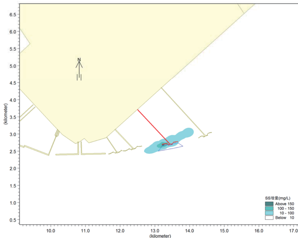
图 5.3-1 疏浚施工代表点 1 悬浮物影响范围
