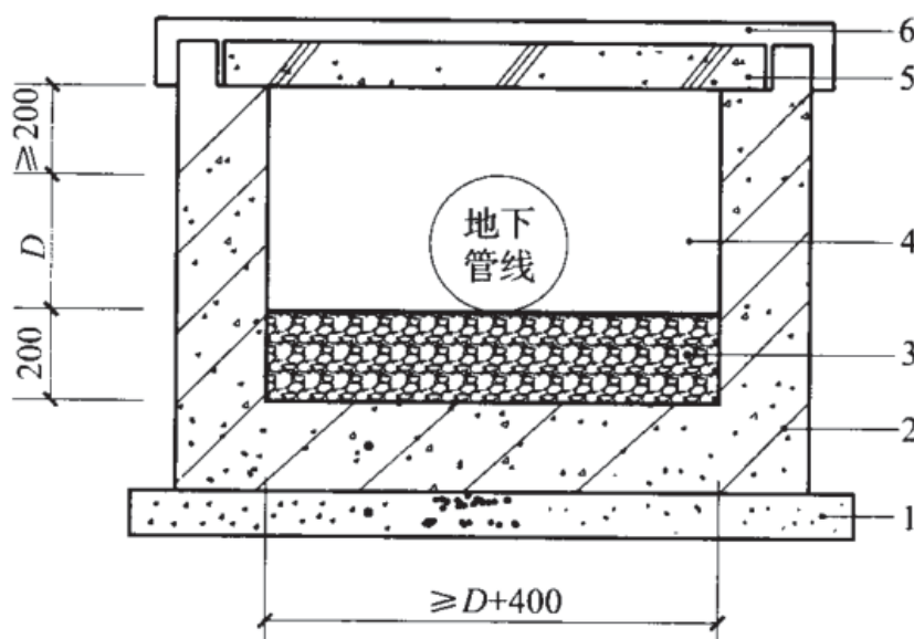
图 8.2-4 抗渗钢筋混凝土管沟防渗层示意
