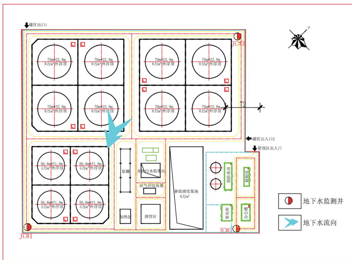
图 8.2-6 厂区地下水监控井分布图
