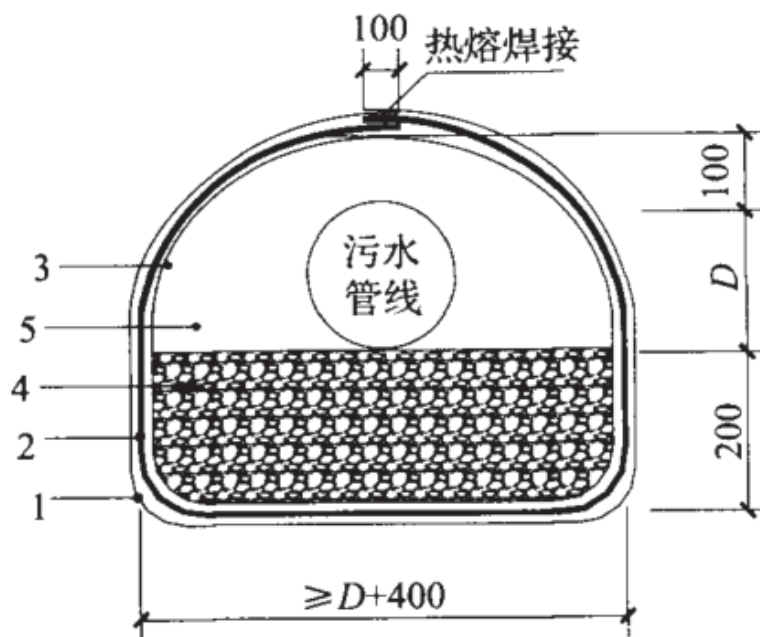
图 8.2-3 地下管道高密度聚乙烯(HDPE)膜防渗层示意
