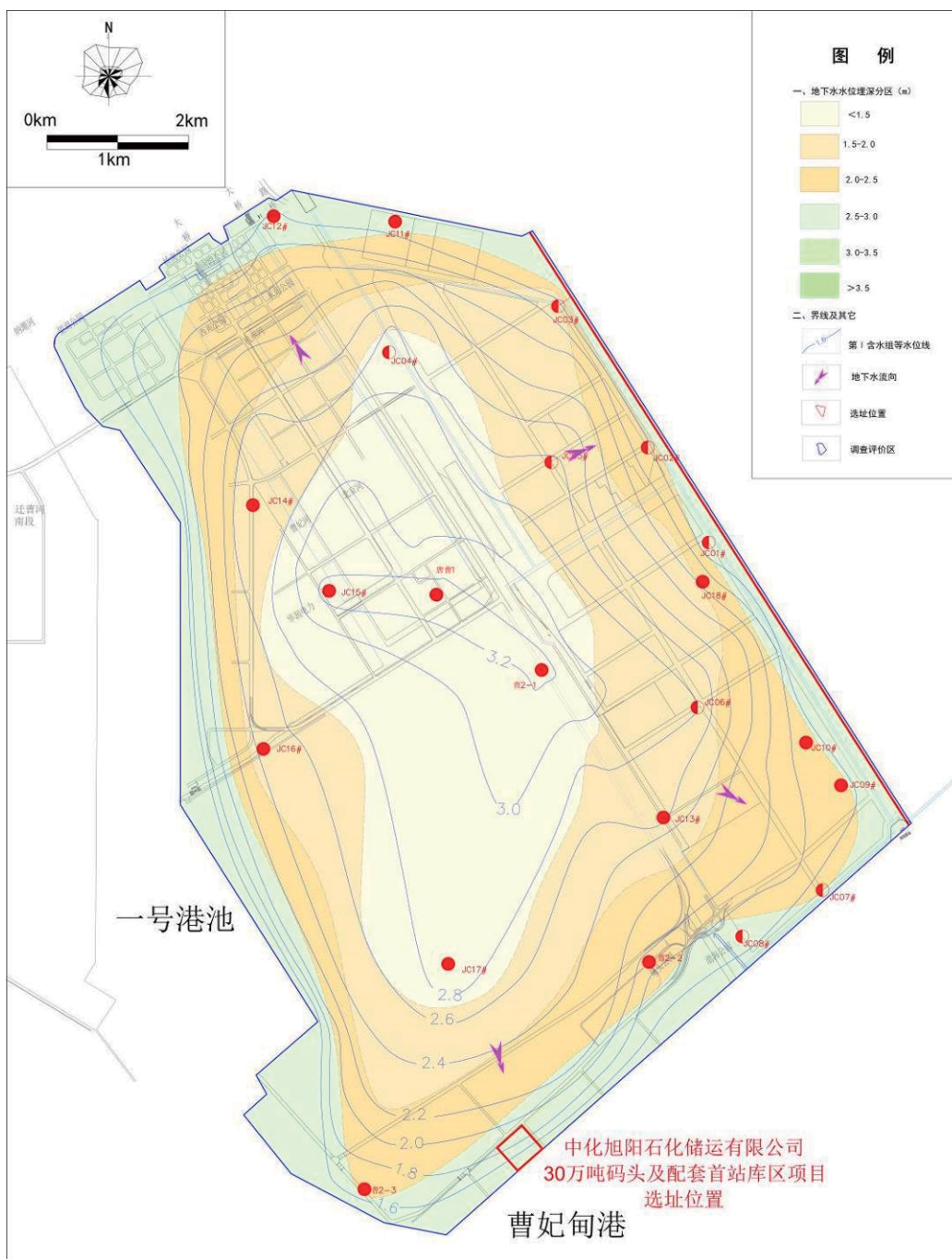
图 4.11-5 2018 年 4 月调查评价区第 I 含水组地下水流场图
