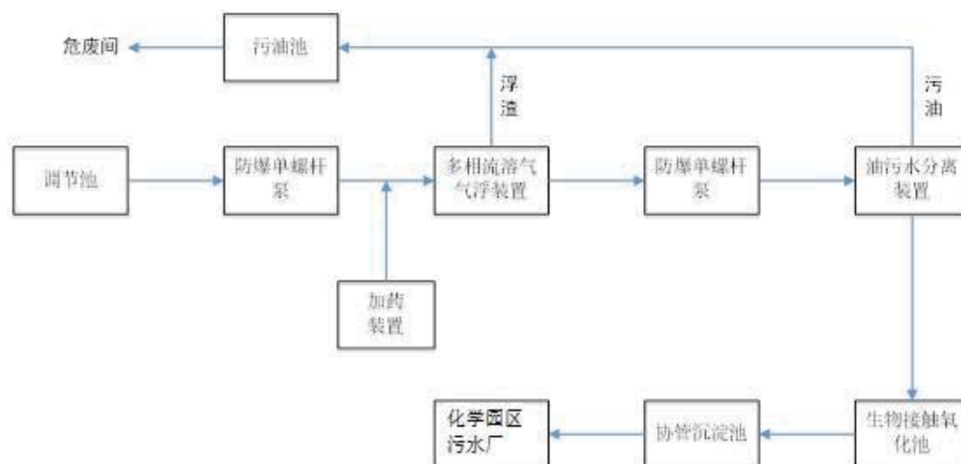
图 8.2-1 项目油污水处理工艺流程图
