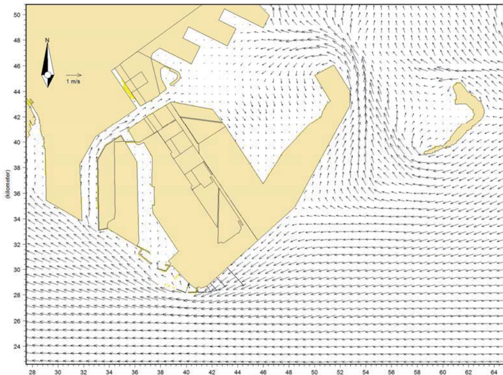
图 5.1-13 现状涨急局部流场（大潮）
