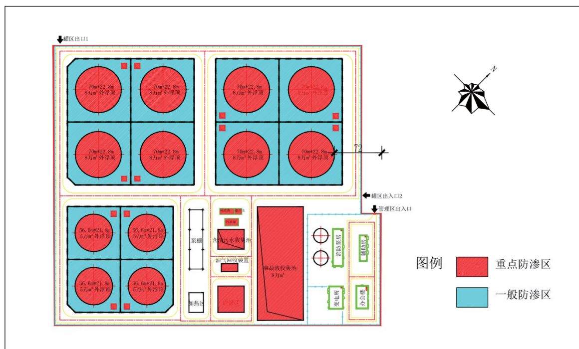
图 8.2-5 厂区防渗分区图
