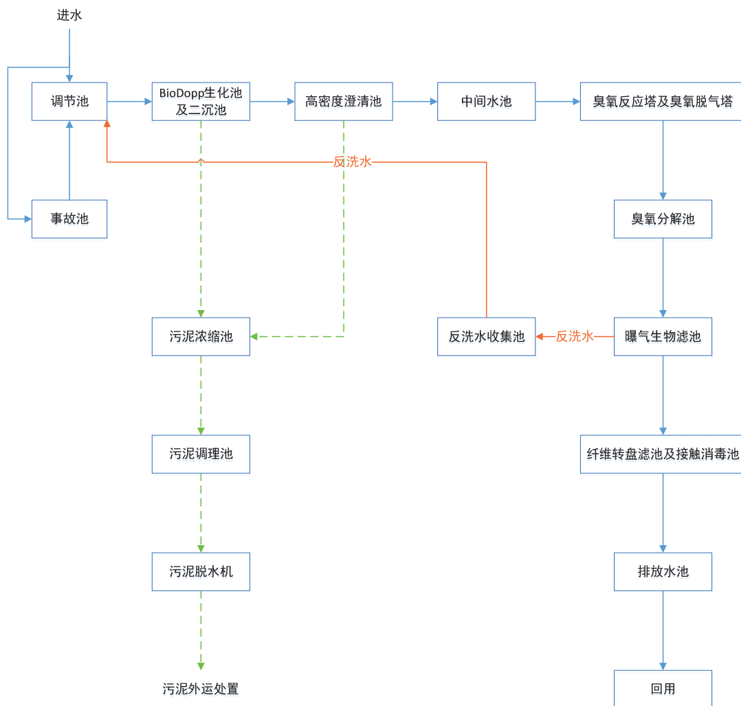
图 8.2-2 曹妃甸化学园区污水处理厂污水处理工艺流程图 化学园区污水处理厂一期工程进水水质如下：
