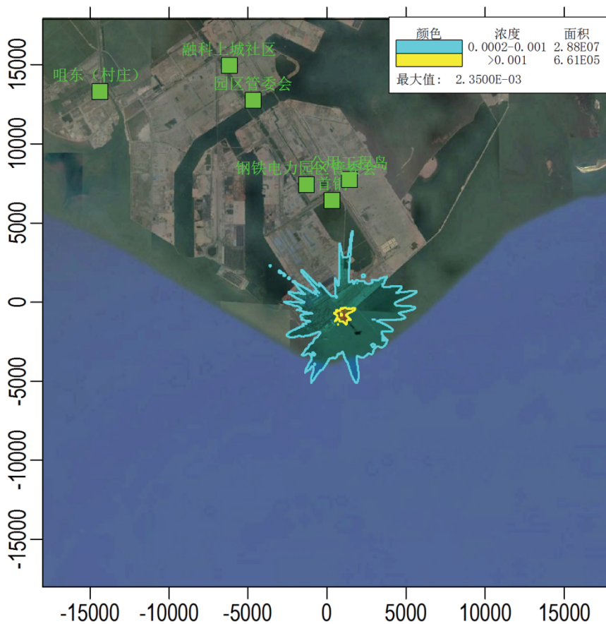
图 6.1-9 NO 2 新增污染源最大日平均质量浓度分布图
