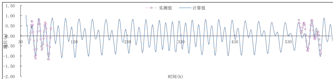
图 5.1-4 曹妃甸站 H2 潮位验证过程线
