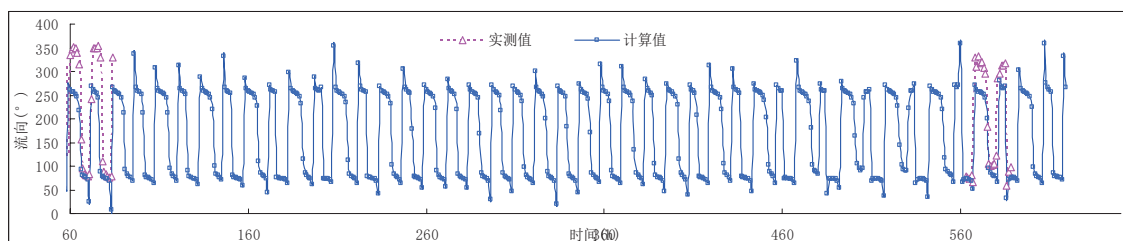
图 5.1-10 V6 站流速、流向验证
