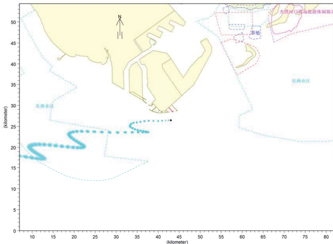
图 7.5-9 港池和航道交汇处 E 风不利风况下涨潮期溢油事故发生 72 小时影响范围
