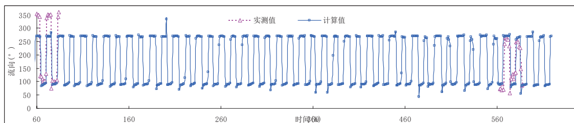
图 5.1-8 V4 站流速、流向验证
