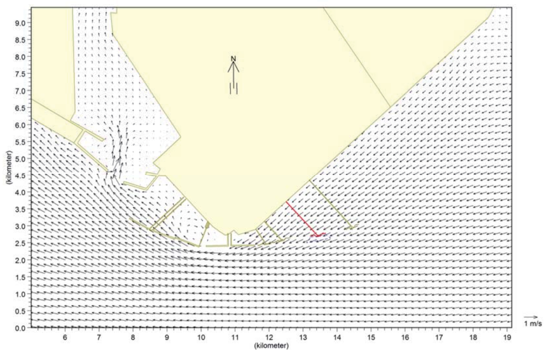
图 5.1-19 工程后涨急时刻潮流矢量图
