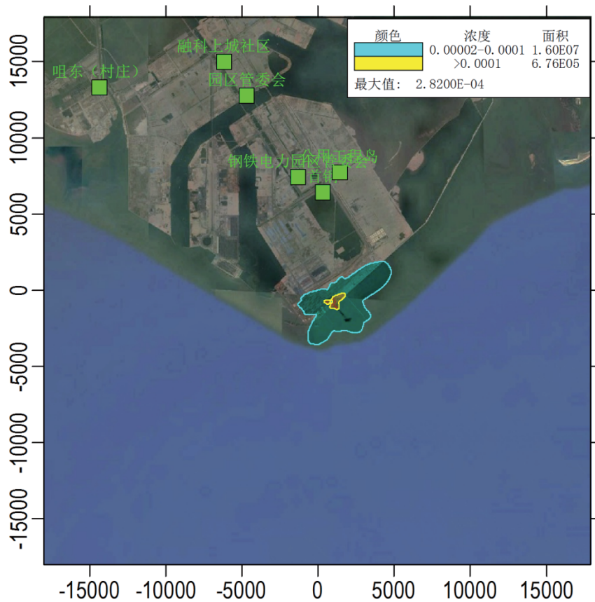
图 6.1-10 NO 2 新增污染源年均质量浓度分布图
