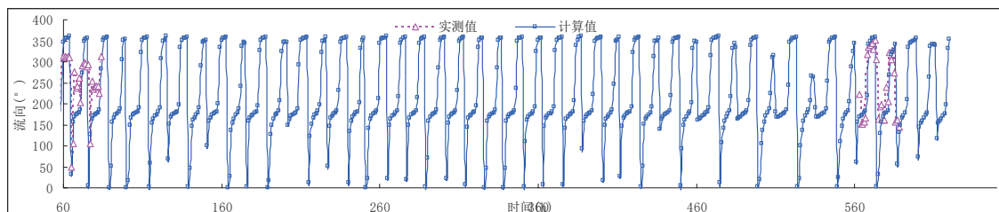
图 5.1-9 V5 站流速、流向验证
