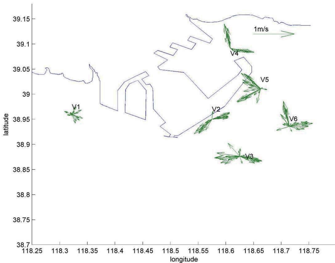
图 4.2-7 大潮期（4月 18-19 日）观测站位底层海流矢量图
