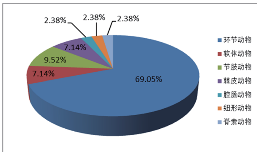
图 4.7-6 调查海域大型底栖生物种类组成与分布
