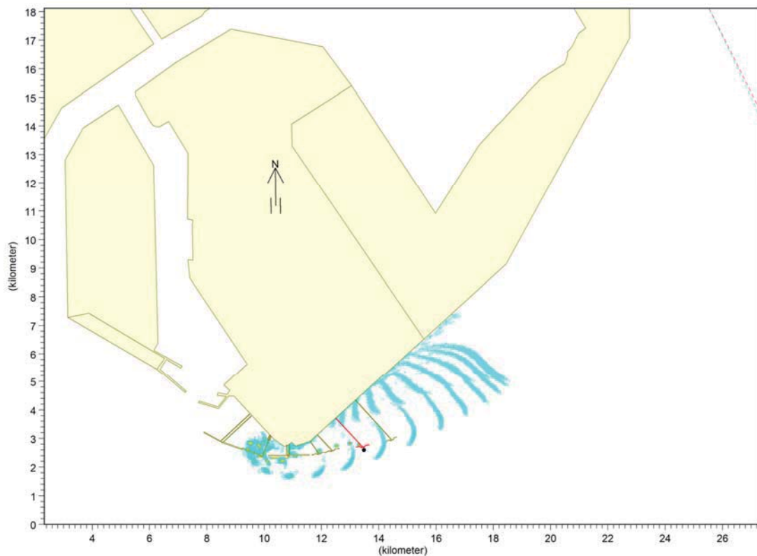
图 7.5-1 码头前沿处涨潮期夏季风风况下溢油事故发生 72 小时影响范围
