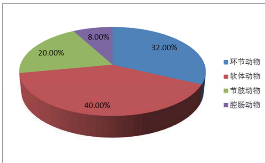
图 4.7-9 潮间带大型底栖生物种类组成与分布
