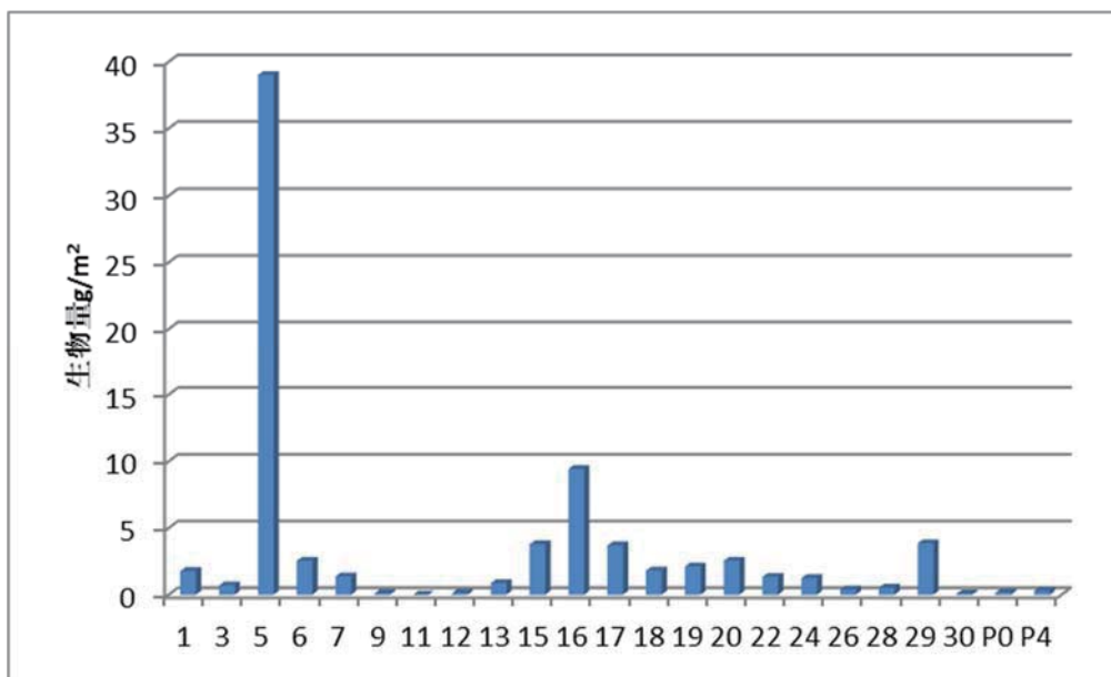
图 4.7-8 调查海域大型底栖生物生物量分布 (g/m 2 )
