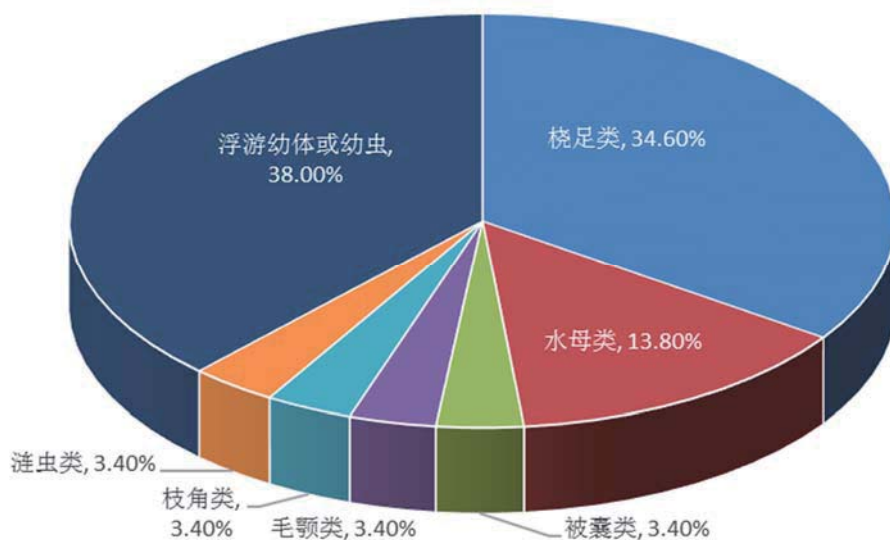
图 4.7-12 调查海域浮游动物种类组成与分布
