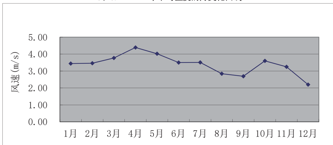
图 6.1-2 年平均风速的月变化曲线
