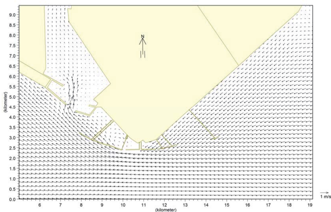
图 5.1-17 工程前涨急时刻潮流矢量图
