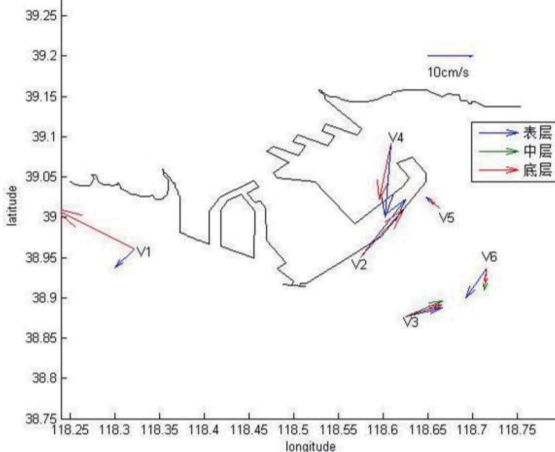
图 4.2-10 曹妃甸附近海域观测站位大潮各层余流矢量图
