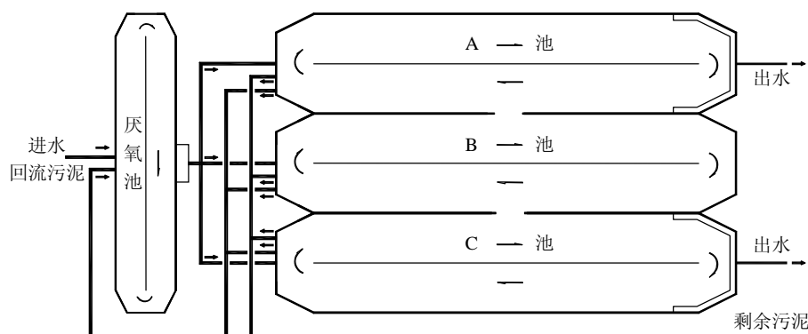
图 A.3 三槽氧化沟工艺流程
