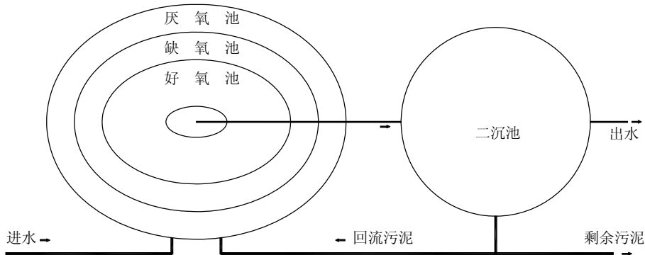
图 A.5 同心圆向心流氧化沟工艺流程
