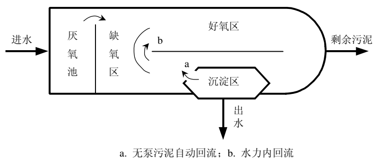
图 B.1 一体化氧化沟工艺流程
