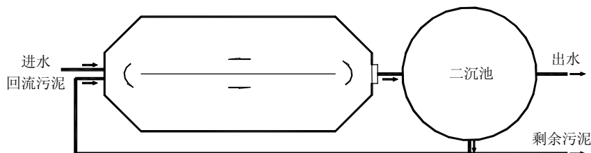
图 A.1 单槽氧化沟工艺流程
