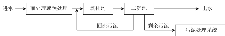
图 1 氧化沟工艺流程
