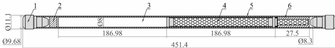
1. 外端塞；2. 垫块；3. 钴棒；4. 源芯；5. 外包壳；6. TY型源包壳 RSCOGYC 型特殊形式放射性物品结构示意图
