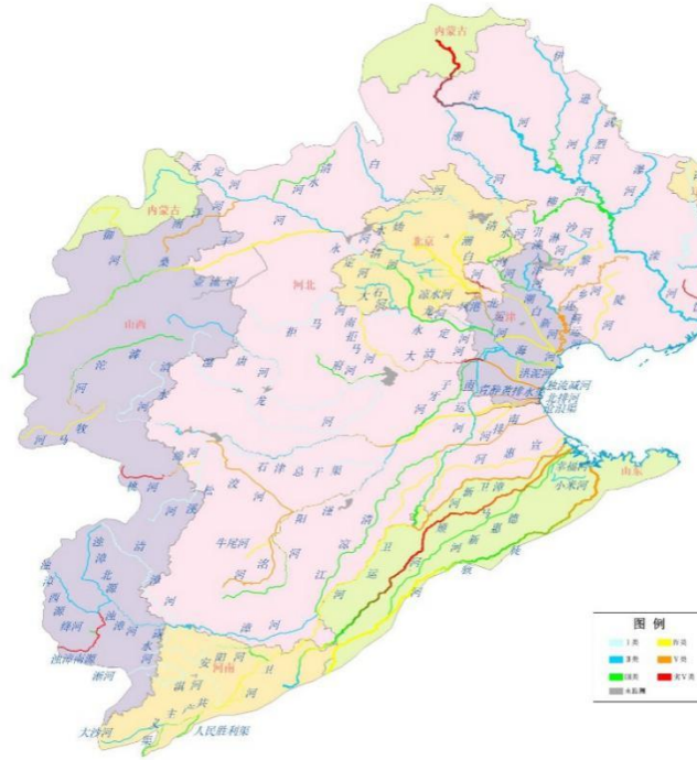
图3 海河流域主要江河水质分布示意图
