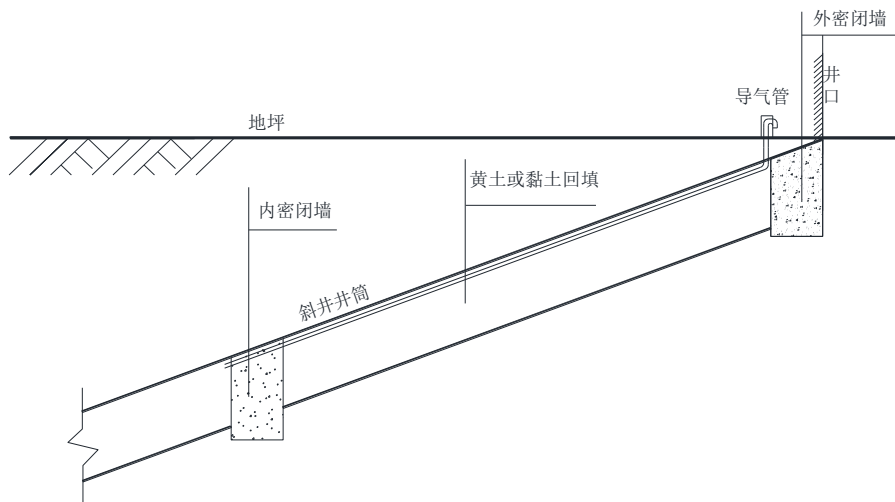
图 5-2 斜井封填示意图
