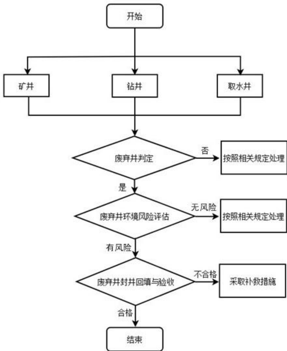
图 2-1 废弃井封井回填工作流程图
