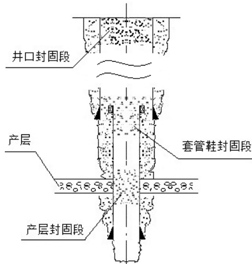
c)尾管完成井
