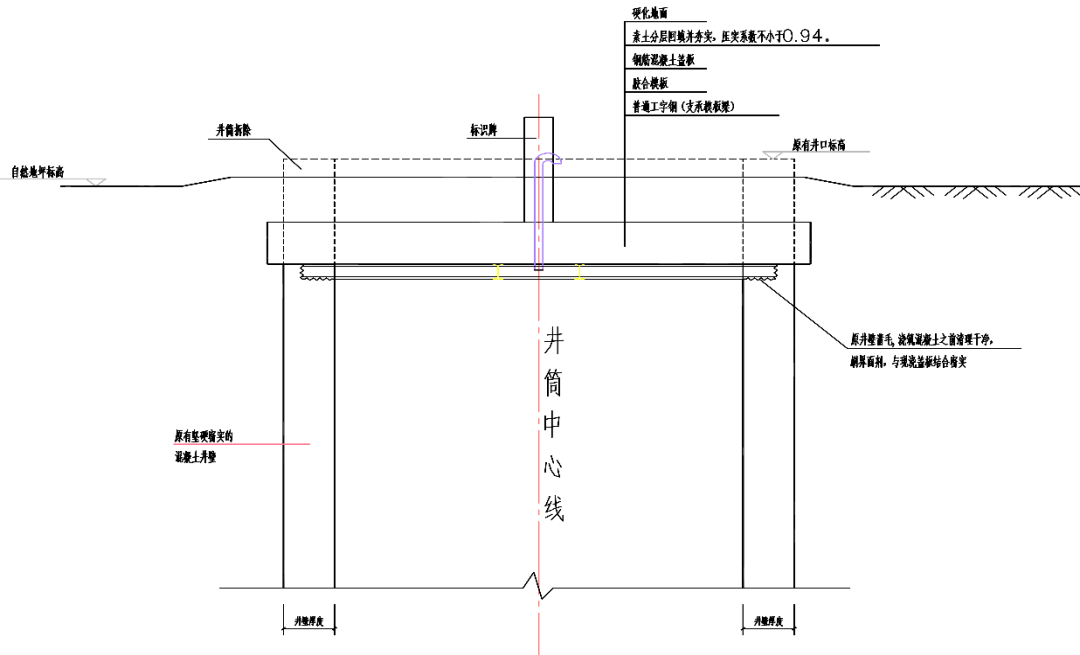
图 5-1 竖井井筒剖面图
