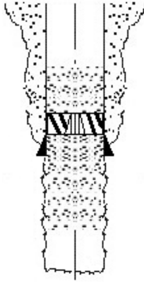
图 5-4 水泥承留器封堵裸眼示意图
