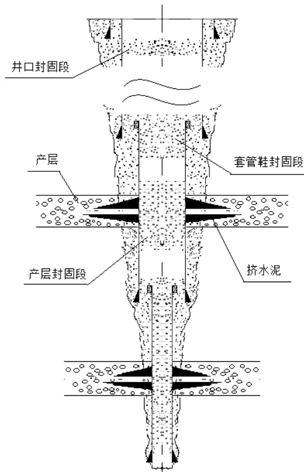
图 5-12 高风险井封井示意图
