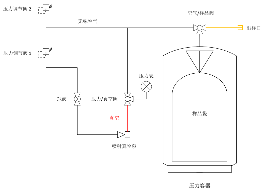
附图 C.1 压力稀释法示意图
