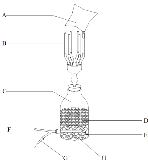
A—嗅辨袋；B—分气器；C—玻璃瓶；D—活性炭；E—分子筛；F—进气口；G—供气量调节阀； H—气体分散管
