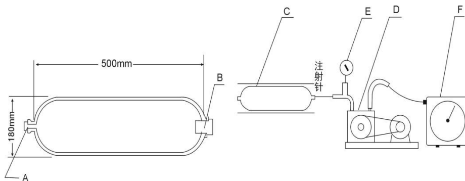
A—进气口硅橡胶塞；B—充填衬袋口硅橡胶塞；C—真空瓶；D—抽气真空泵；E—真空表；F—气量计
