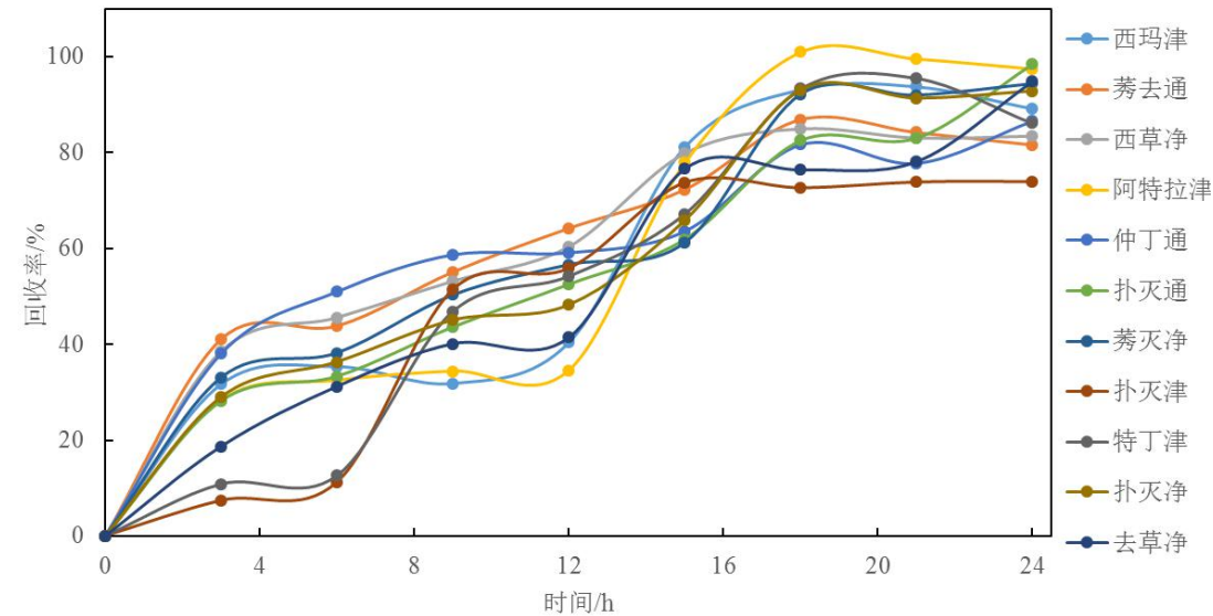
图 5.6-1 不同提取时间下的索氏提取回收率
