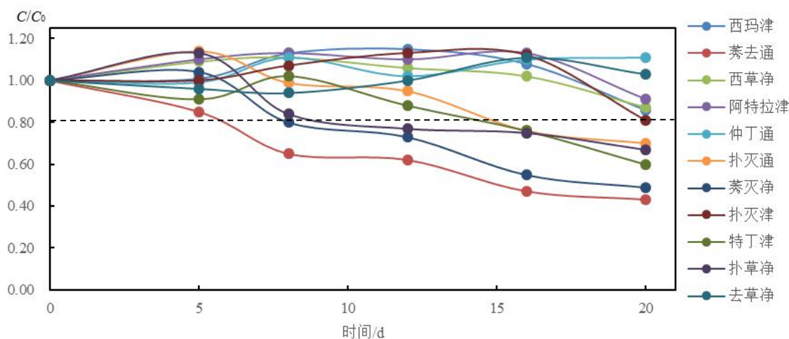
图 5.5-2 11 种均三嗪类农药在土壤样品中含量变化趋势图
