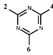
图 2-1 均三嗪化合物基本结构
