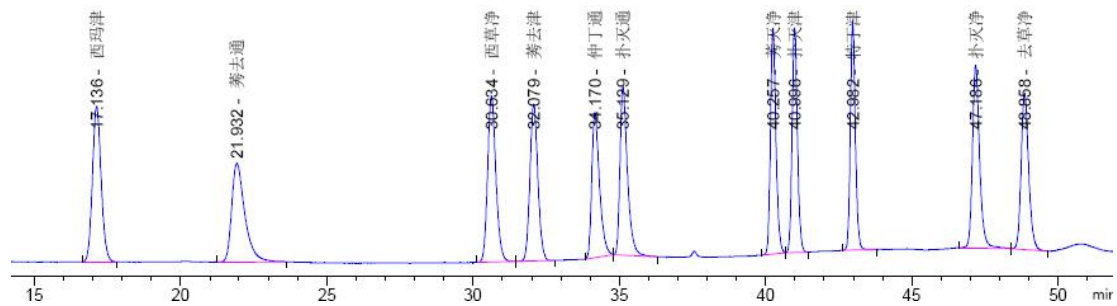
C.硅胶柱净化后样品提取液色谱图
