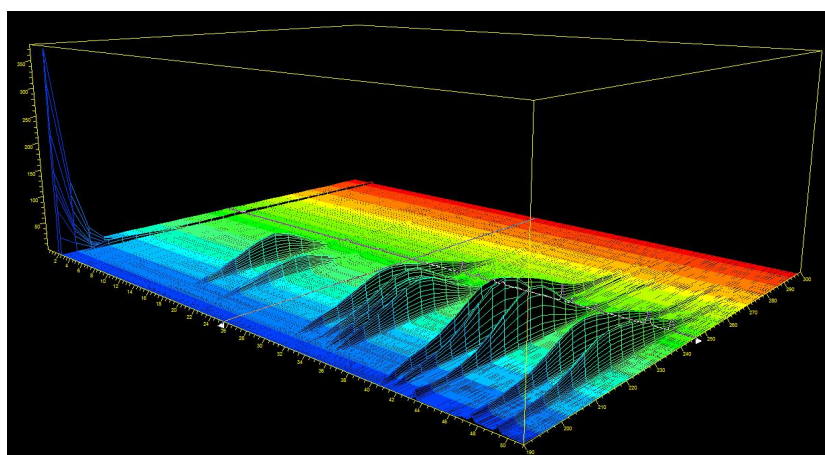
B.DAD 三维扫描谱图
