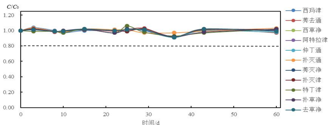
图 5.5-4 11 种均三嗪类农药在样品提取液中浓度变化趋势图
