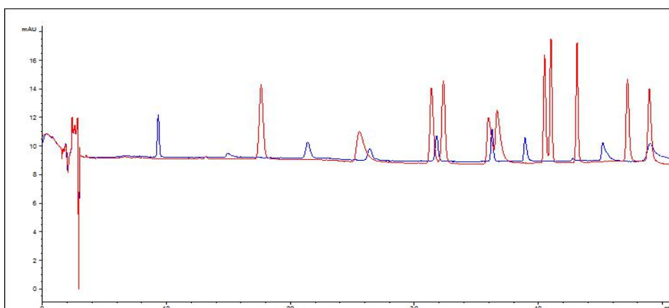
C.净化前酚类化合物与均三嗪类农药液相色谱图 ( \rho=1.00 \text{ mg/L} )
