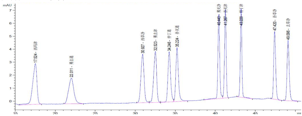
A. 柱温 25 °C
