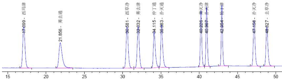
E.氨丙基净化后样品提取液色谱图
