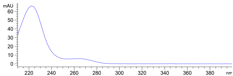
D. 阿特拉津
