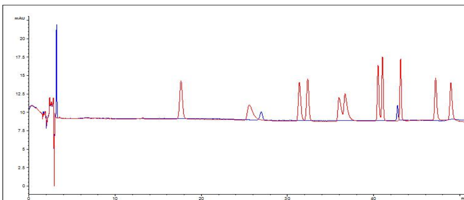
B.邻苯二甲酸酯类化合物与均三嗪类农药液相色谱图 ( \rho=1.00 \text{ mg/L} )
