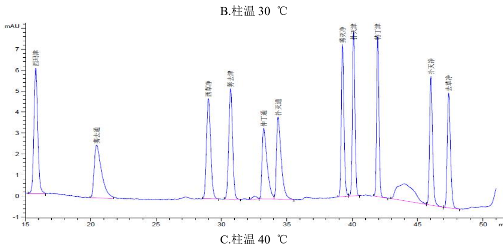
图 5.6-8 不同柱温时 11 种均三嗪类农药液相色谱图 ( \rho=0.50 \text{ mg/L} )
