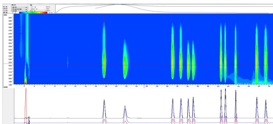
A.DAD 二维扫描谱图
