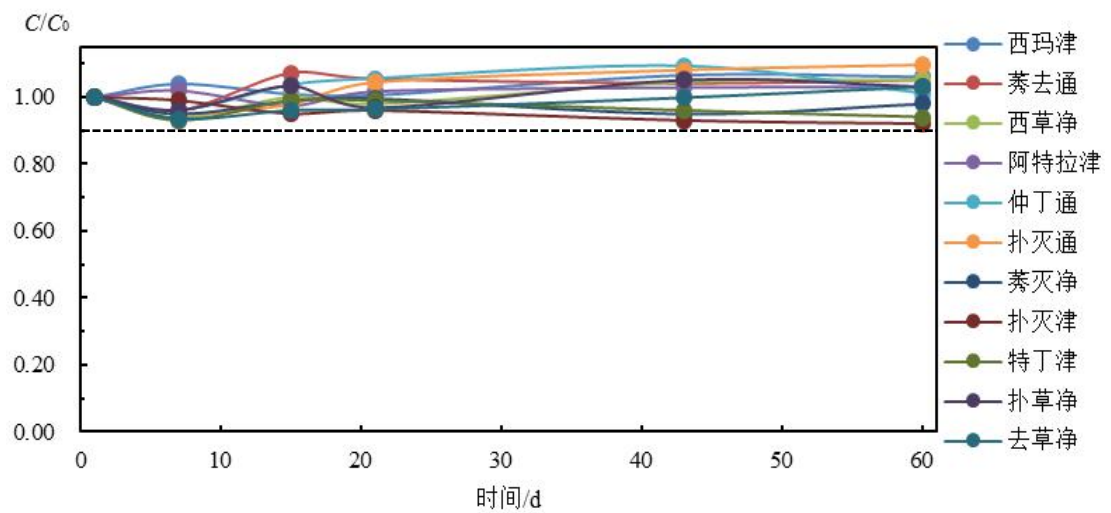
A. 标准使用液 ( \rho=10.0 mg/L)
