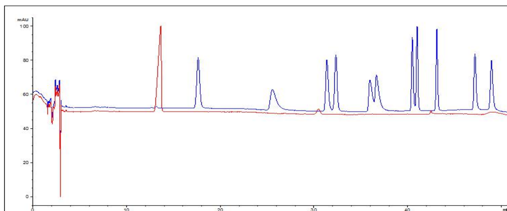
A. 多环芳烃类化合物与均三嗪类农药液相色谱图 ( \rho=1.00 \text{ mg/L} )
