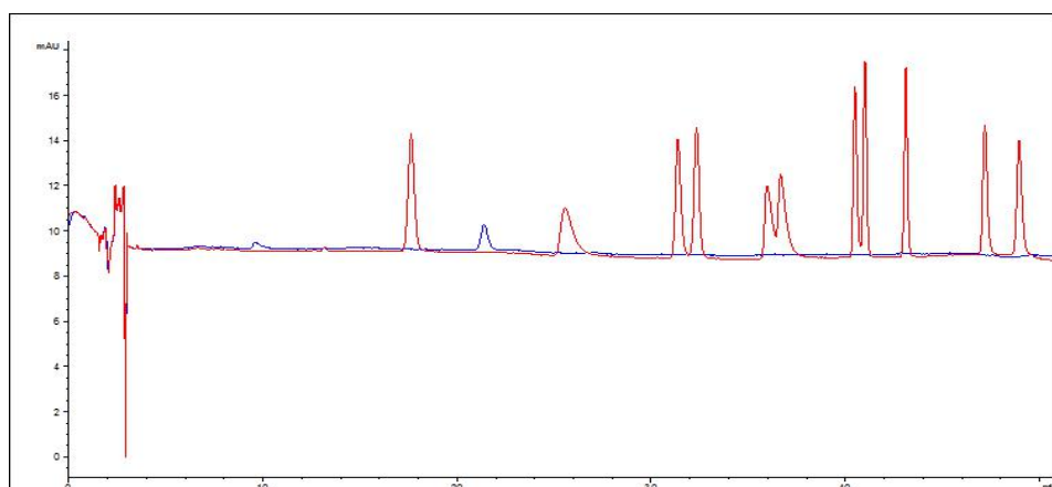
D.净化后酚类化合物与均三嗪类农药液相色谱图 ( \rho=1.00 \text{ mg/L} )
