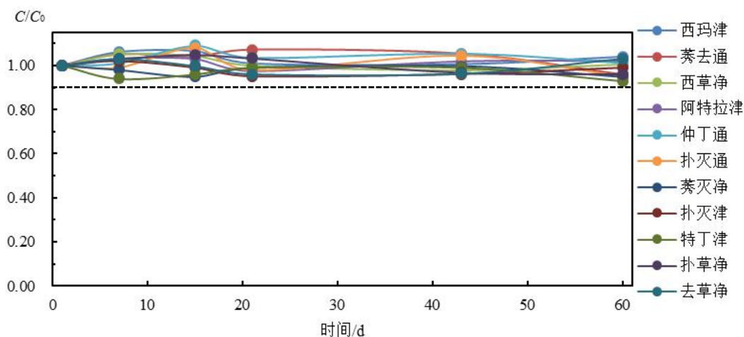
图 5.5-1 标准使用液中 11 种均三嗪类农药含量变化趋势图
