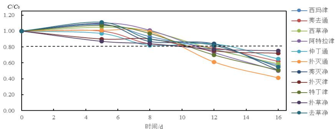
图 5.5-3 11 种均三嗪类农药在沉积物样品中含量变化趋势图
