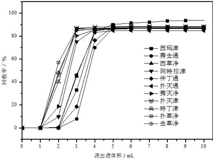
图 5.6-3 11 种均三嗪类农药在固相净化小柱上的流出曲线（氨基柱）
