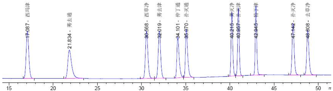
D.氨基柱净化后样品提取液色谱图
