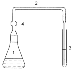
砷化氢发生与吸收装置图
