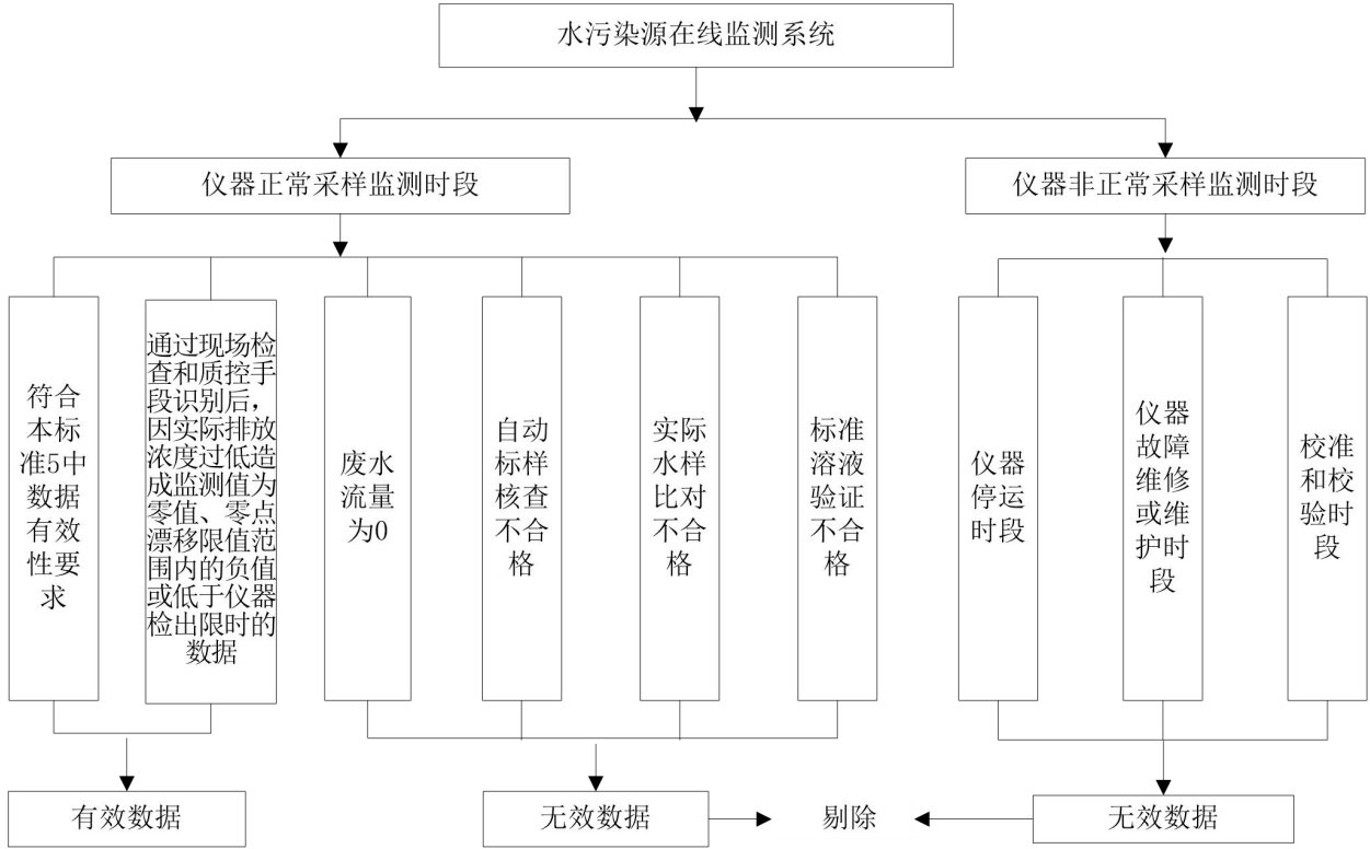
图1 水污染源在线监测系统数据有效性判别流程图
