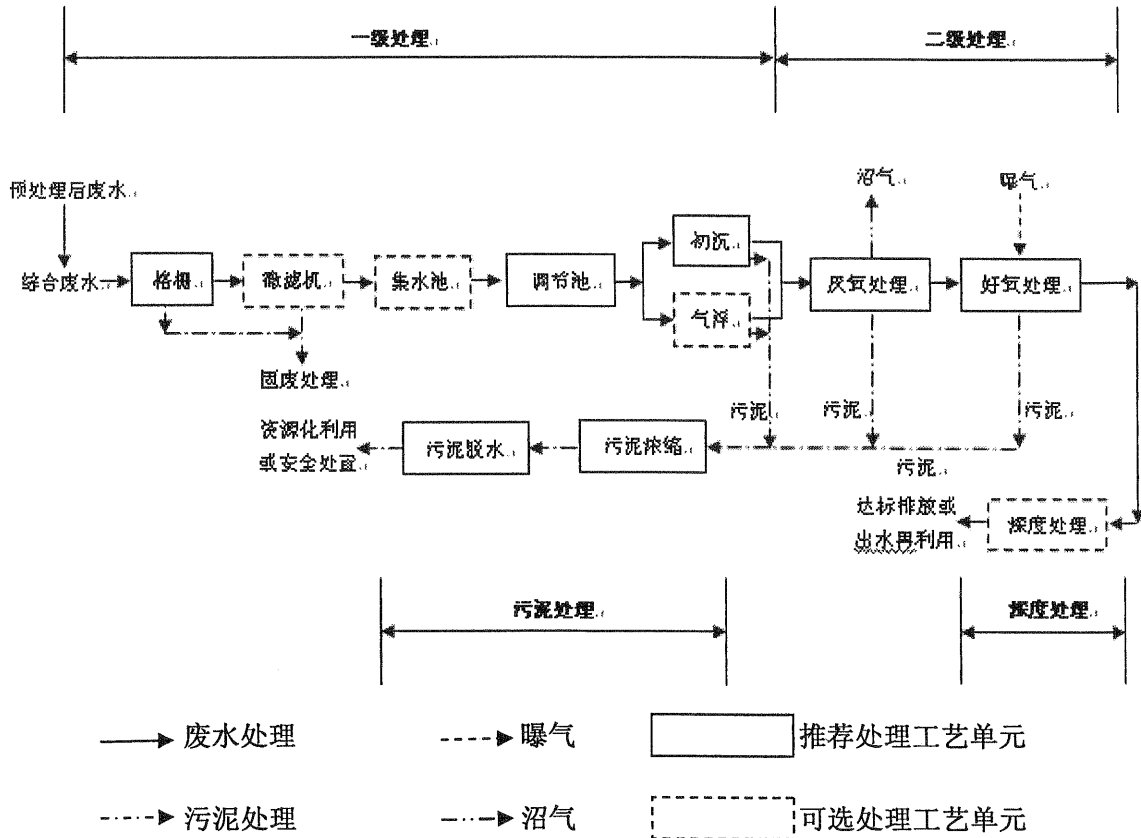
图 1 软饮料制造废水污染治理一般工艺流程
