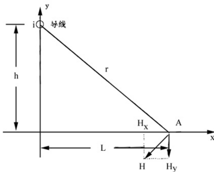
图 D1 磁场向量图
