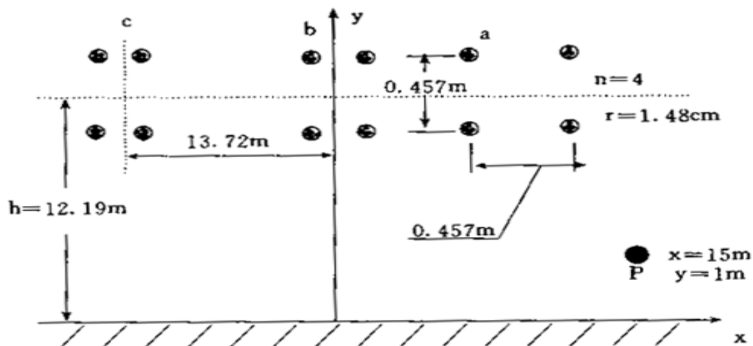
图 C4 计算例图
