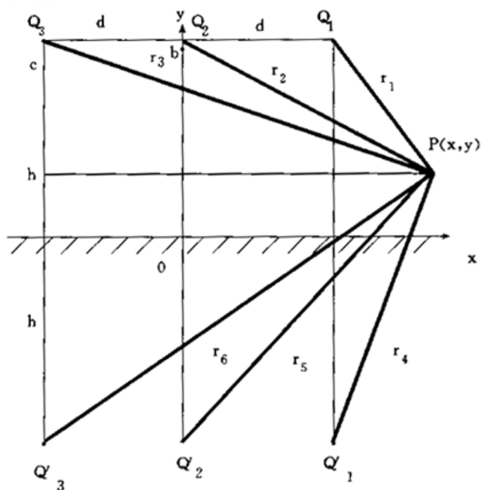
图 C5 各导线坐标图
